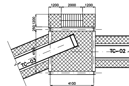
PLANTA DO TRANSPORTADOR TC-03 (TO-03) ESC.1:100
