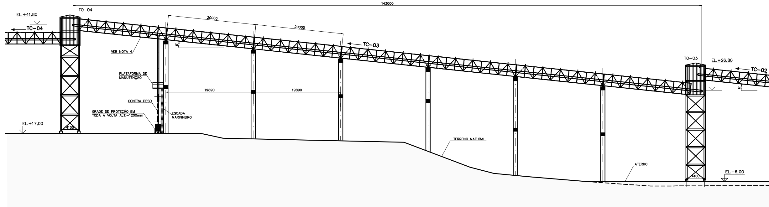
VISTA DO TRANSPORTADOR TC-03 ESC.1:250
