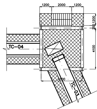
PLANTA DO TRANSPORTADOR TC-03 (TO-04) ESC.1:100
