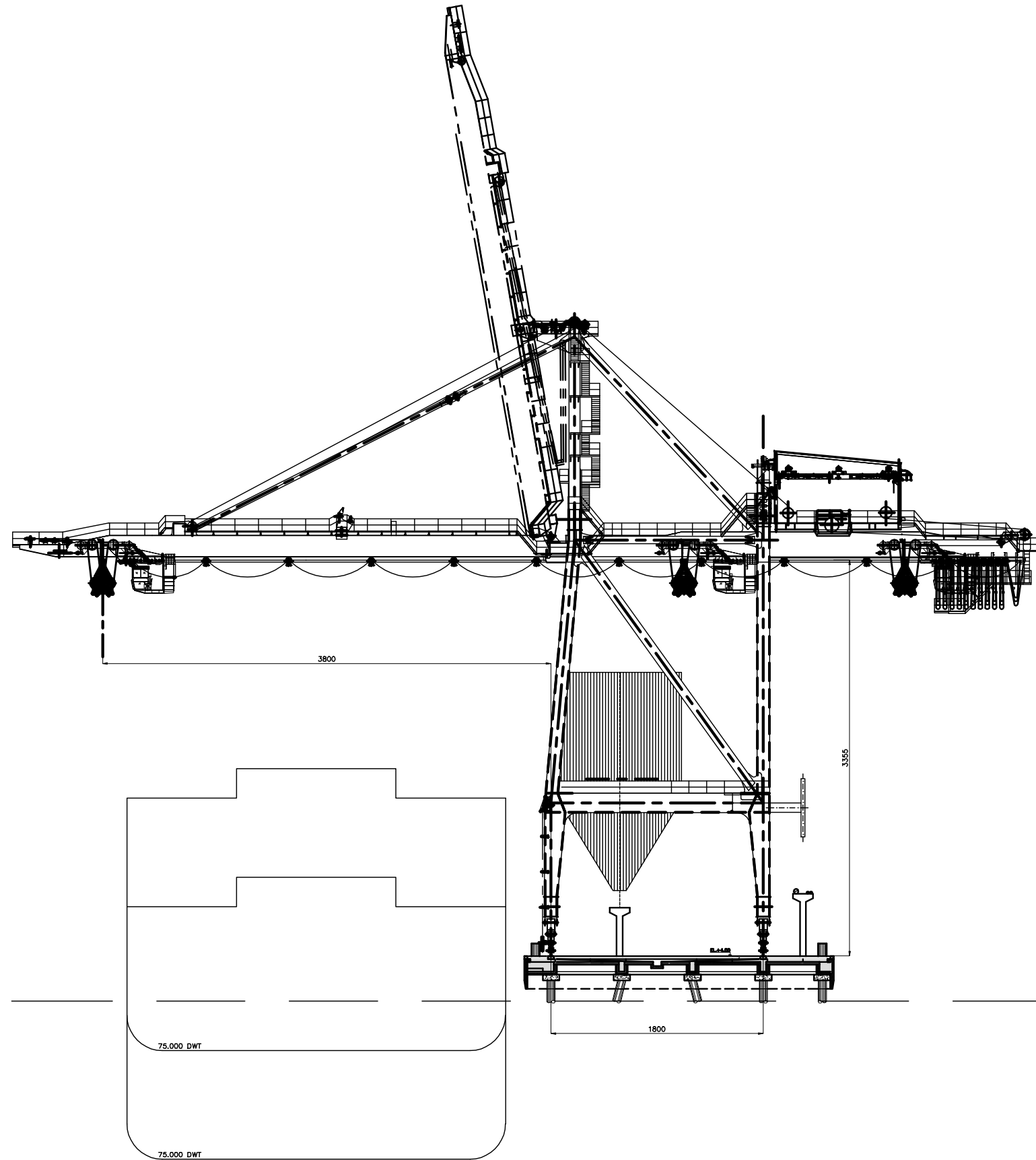
CORTE TÍPICO DO CAIS ESC.1:500
