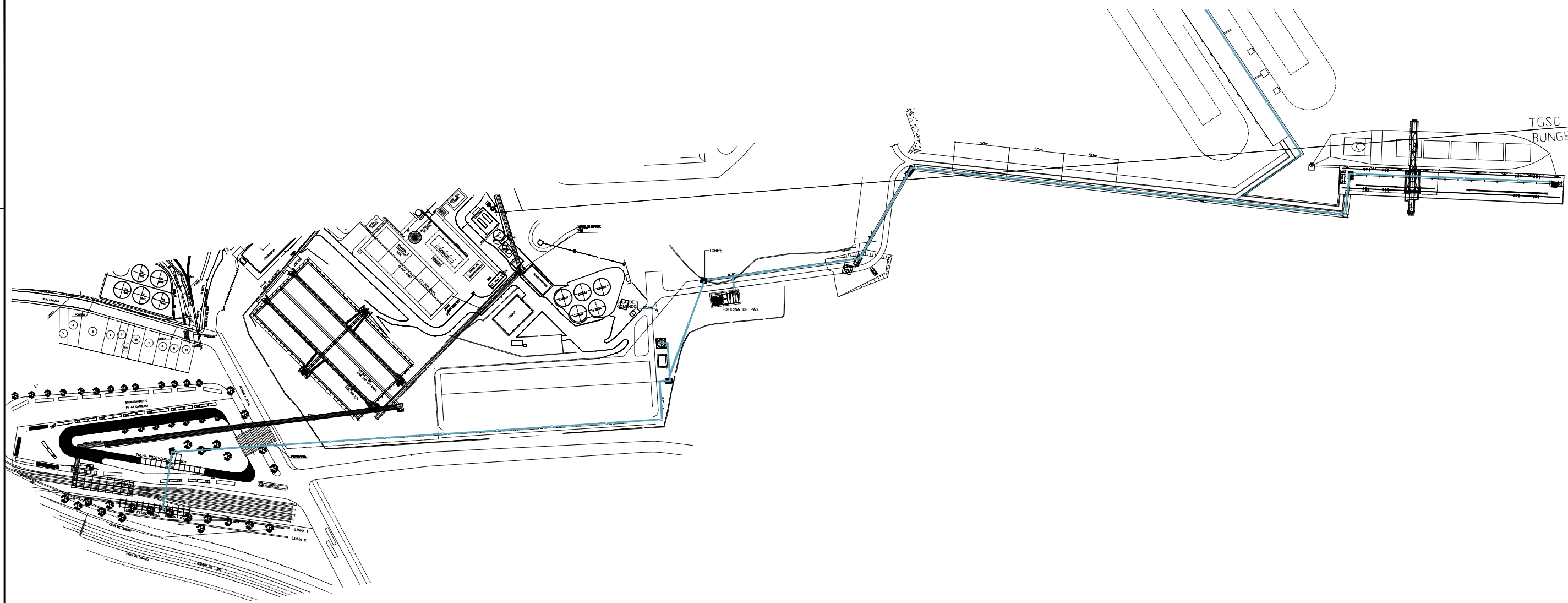
IMPLANTAÇÃO GERAL DA REDE DE ÁGUA DE COMBATE À INCENDIO ESC. 1/1200
