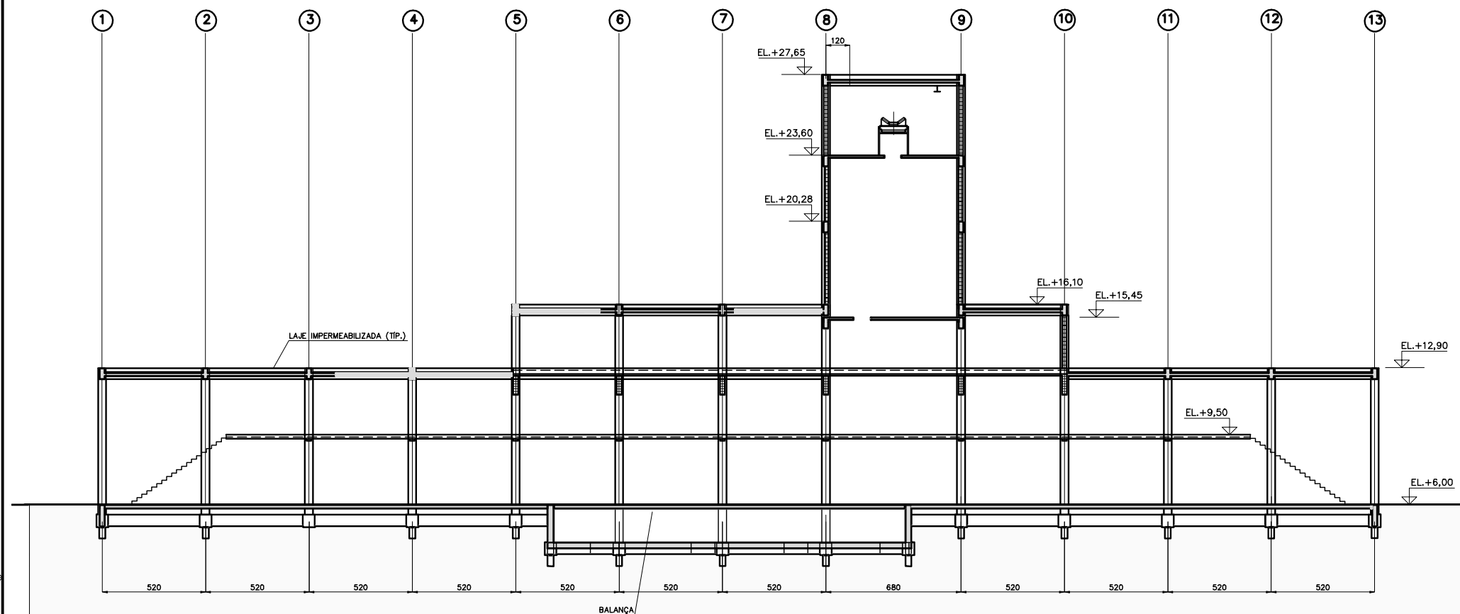
CORTE LONGITUDINAL – TULHA FERROVIÁRIA ESC.1:125
