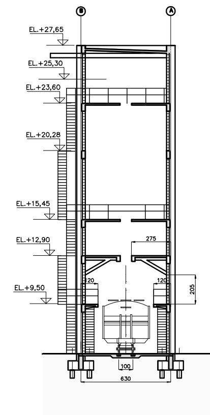
CORTE TRANSVERSAL – TULHA FERROVIÁRIA ESC.1:125
