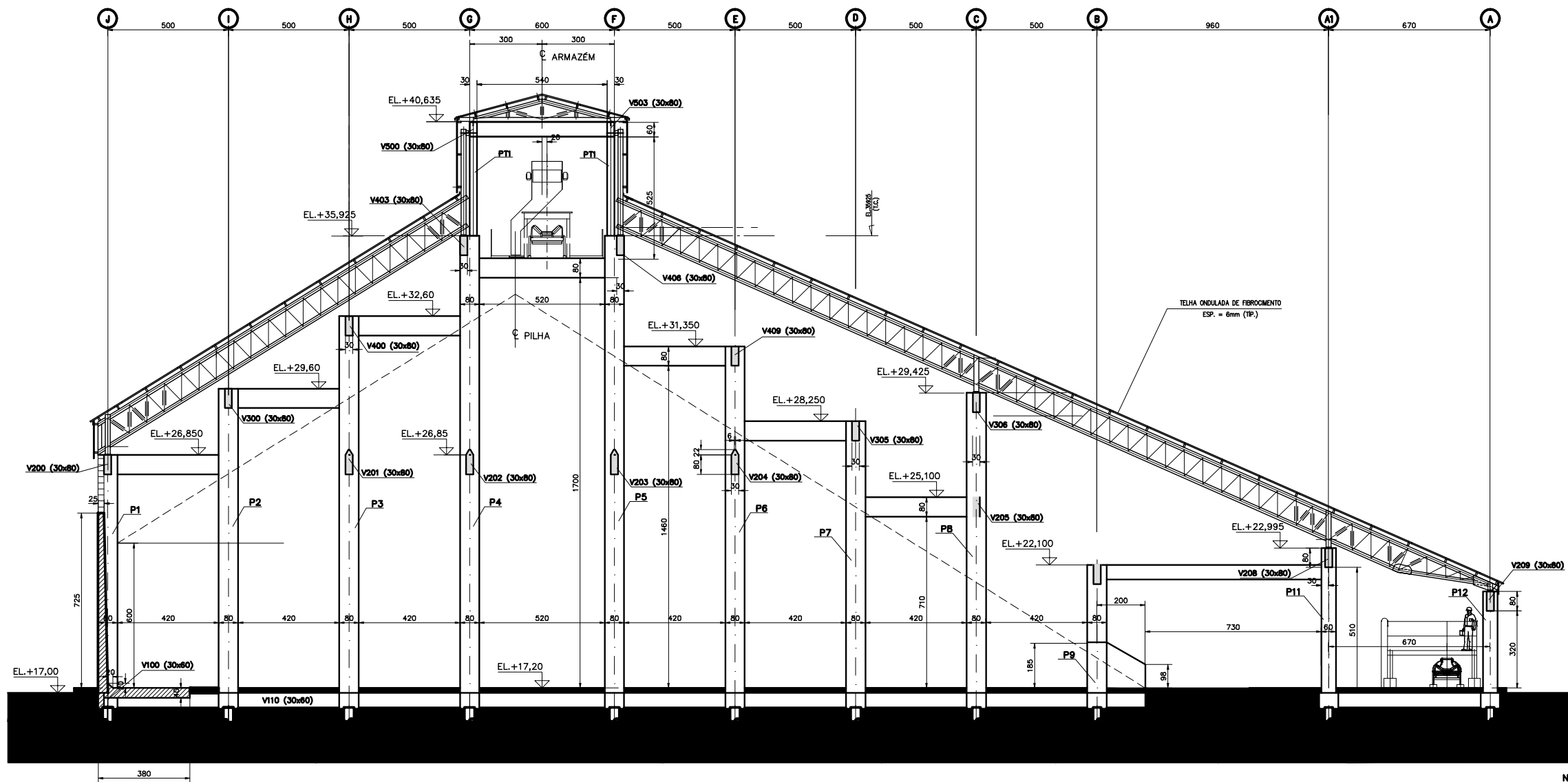
CORTE A-A (TÍPICO) ESC.1:100
