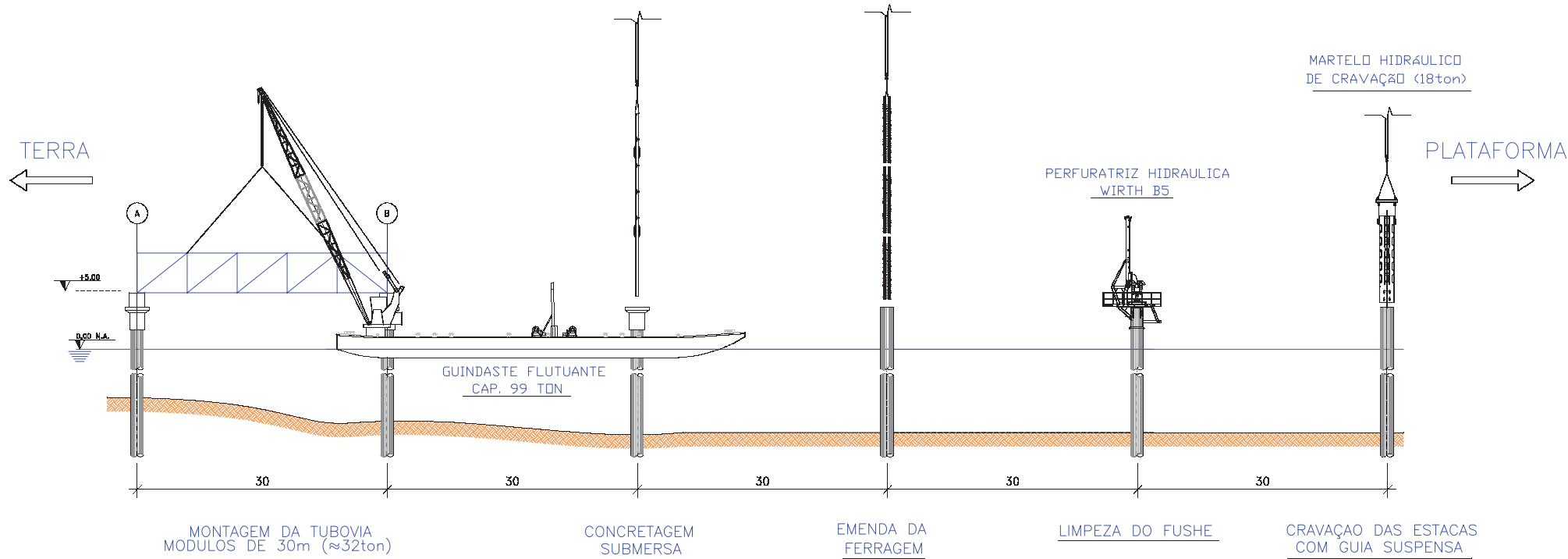
CORTE - EXECUÇÃO TUBOVIA ESCALA 1:12,5
