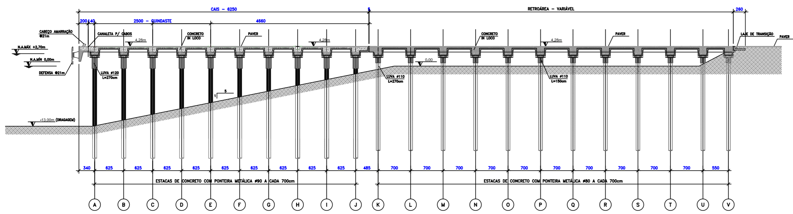
CORTE TRANSVERSAL DO CAIS E PLATAFORMA ESC. 1/500 DIMENSÕES EM CENTÍMETROS EXCETO ONDE INDICADO
