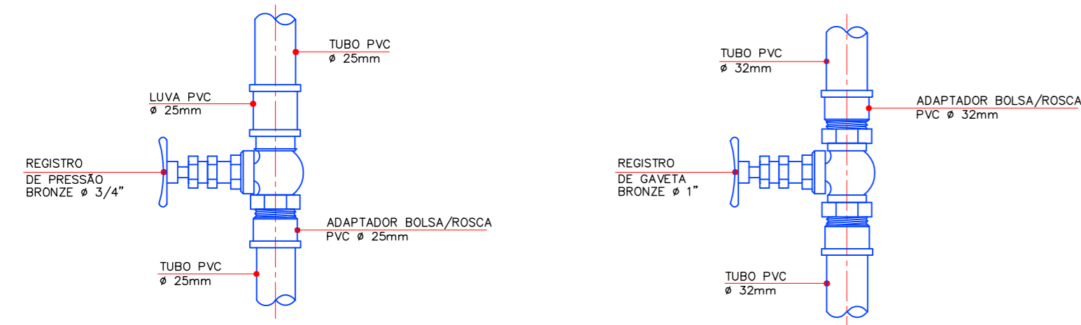
REGISTRO DE GAVETA DETALHE 2 SEM ESCALA
