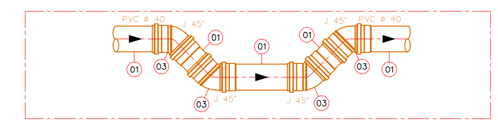
DETALHE 01 SIFÃO-VISTA LATERAL SEM ESCALA
