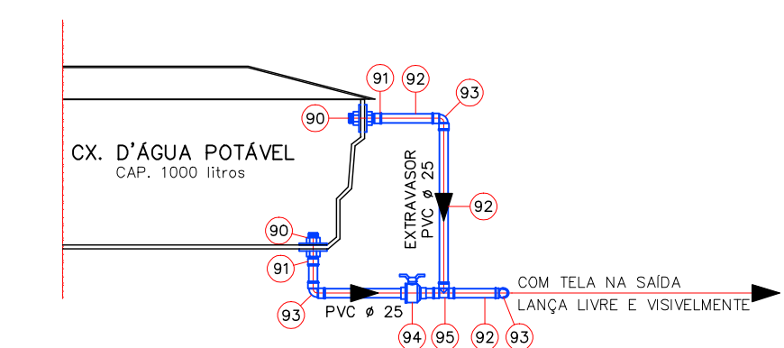
DETALHE 03 EXTRAVASOR/LIMPEZA SEM ESCALA
