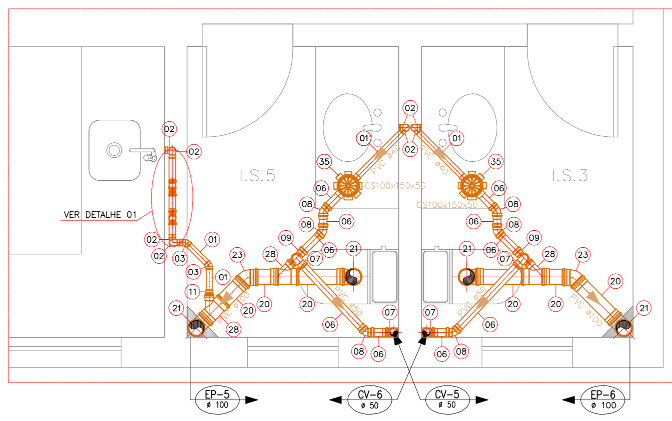
CENTRO ADMINISTRATIVO 3º PAVTO ESGOTO-DETALHE BANHEIROS 01 AO 14 ESCALA 1:25
