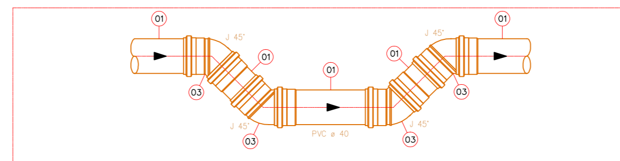
DETALHE 01 SIFÃO SEM ESCALA
