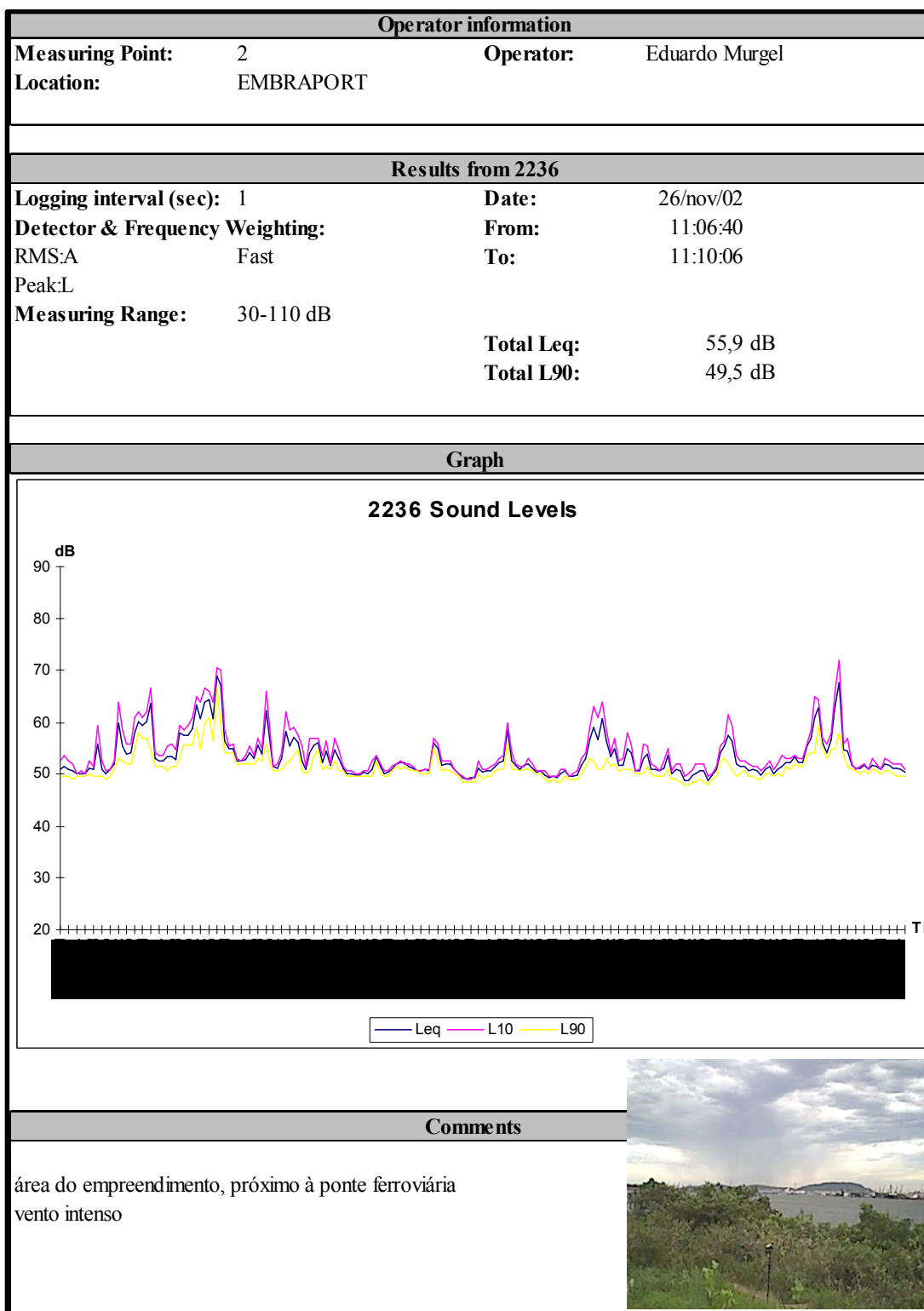
Figura 8.1- 5– Caracterização dos Níveis de Ruído Ponto 2
