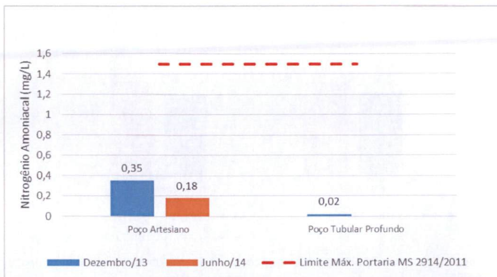
Gráfico 5-11: Resultados analíticos para o Nitrogênio Amoniacal nos poços artesiano e tubular profundo, nos meses de estudo.
