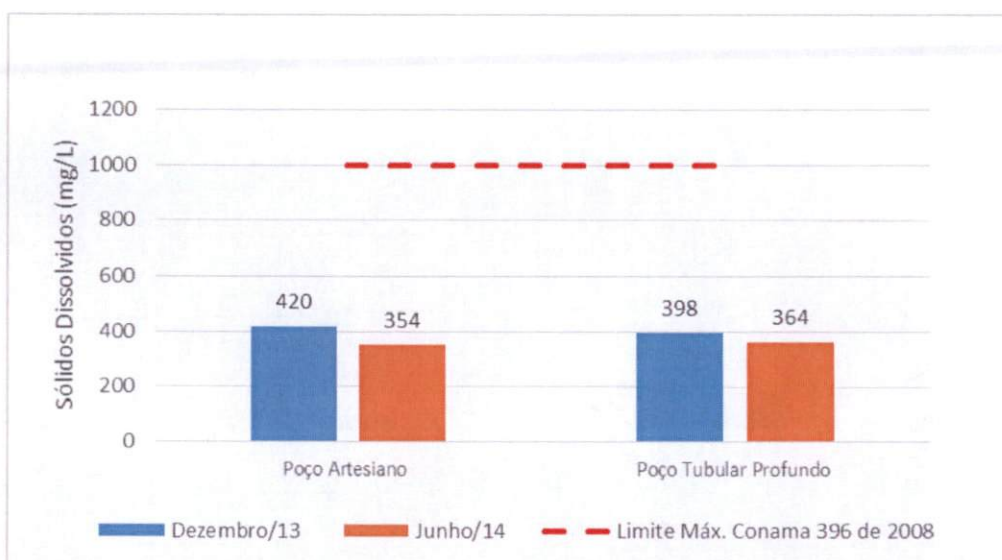
Gráfico 5-13: Resultados analíticos para os Sólidos Dissolvidos Totais nos poços artesiano e tubular profundo, nos meses de estudo.
