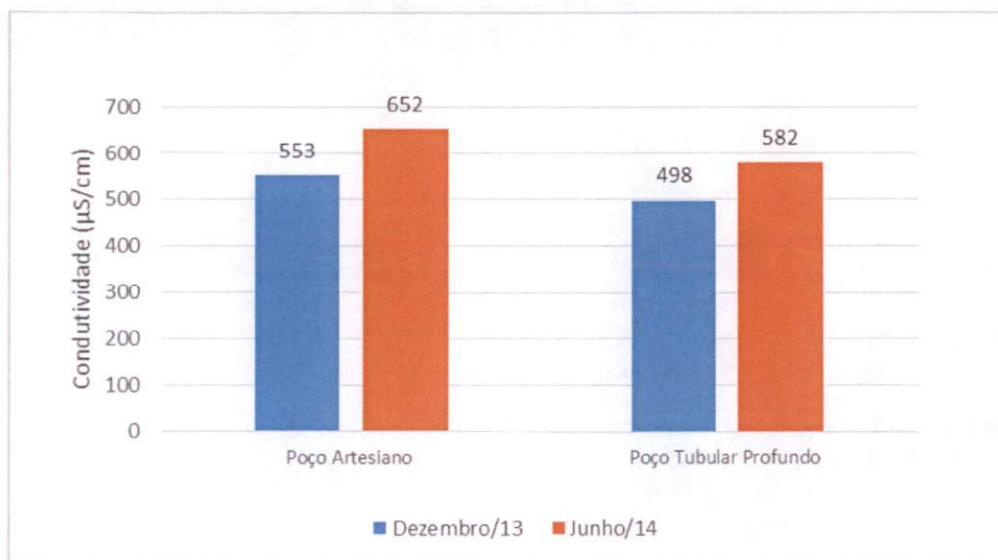
Gráfico 5-6: Resultados analíticos para a Condutividade nos poços artesiano e tubular profundo, nos meses de estudo.
