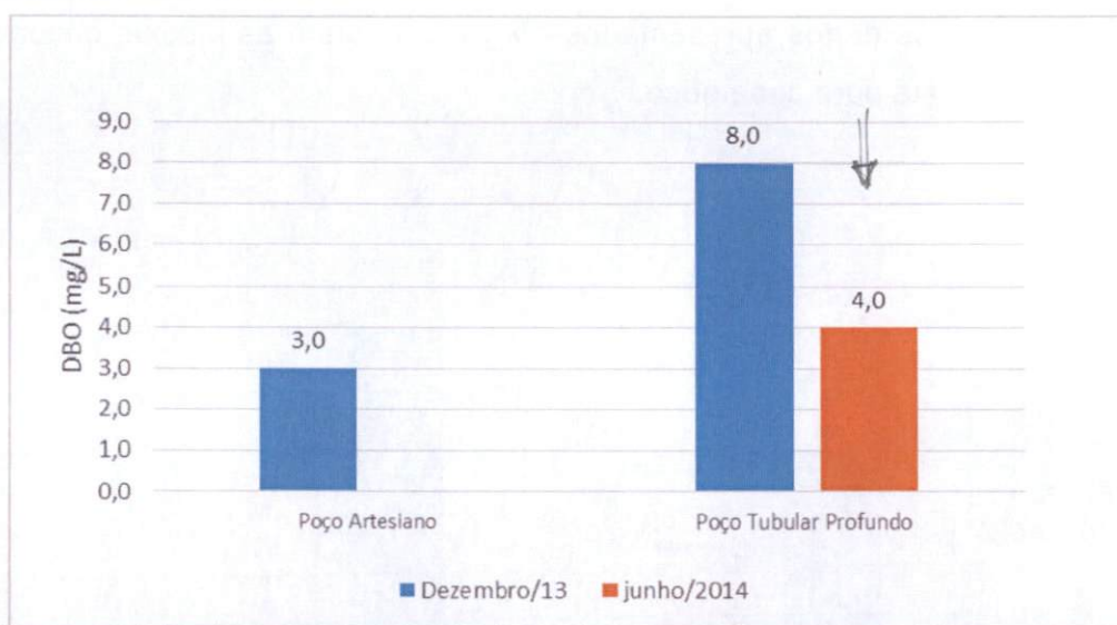
Gráfico 5-7: Resultados analíticos para a DBO nos poços artesiano e tubular profundo, nos meses de estudo.
