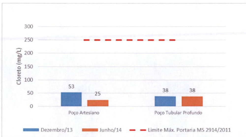
Gráfico 5-5: Resultados analíticos para o Cloreto Total nos poços artesiano e tubular profundo, nos meses de estudo.
