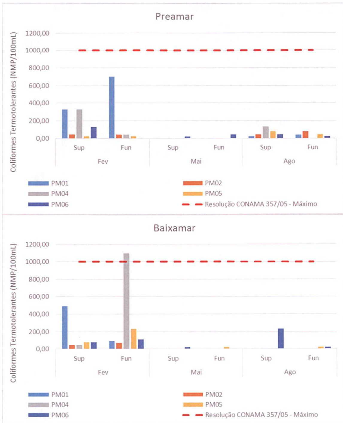
Gráfico 5-22: Valores de coliformes termotolerantes das estações do rio Barra Nova nas profundidades de superfície e fundo sob condição de preamar e baixamar ao longo das campanhas de monitoramento.
