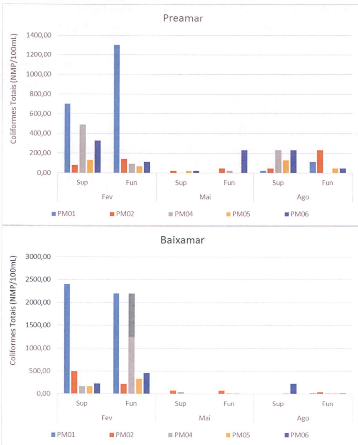
Gráfico 5-23: Valores de coliformes totais das estações do rio Barra Nova nas profundidades de superfície e fundo sob condição de preamar e baixamar ao longo das campanhas de monitoramento.
