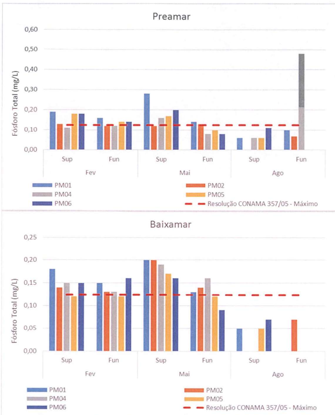
Gráfico 5-16: Valores de Fósforo total das estações do rio Barra Nova nas profundidades de superfície e fundo sob condição de preamar e baixamar ao longo das campanhas de monitoramento.
