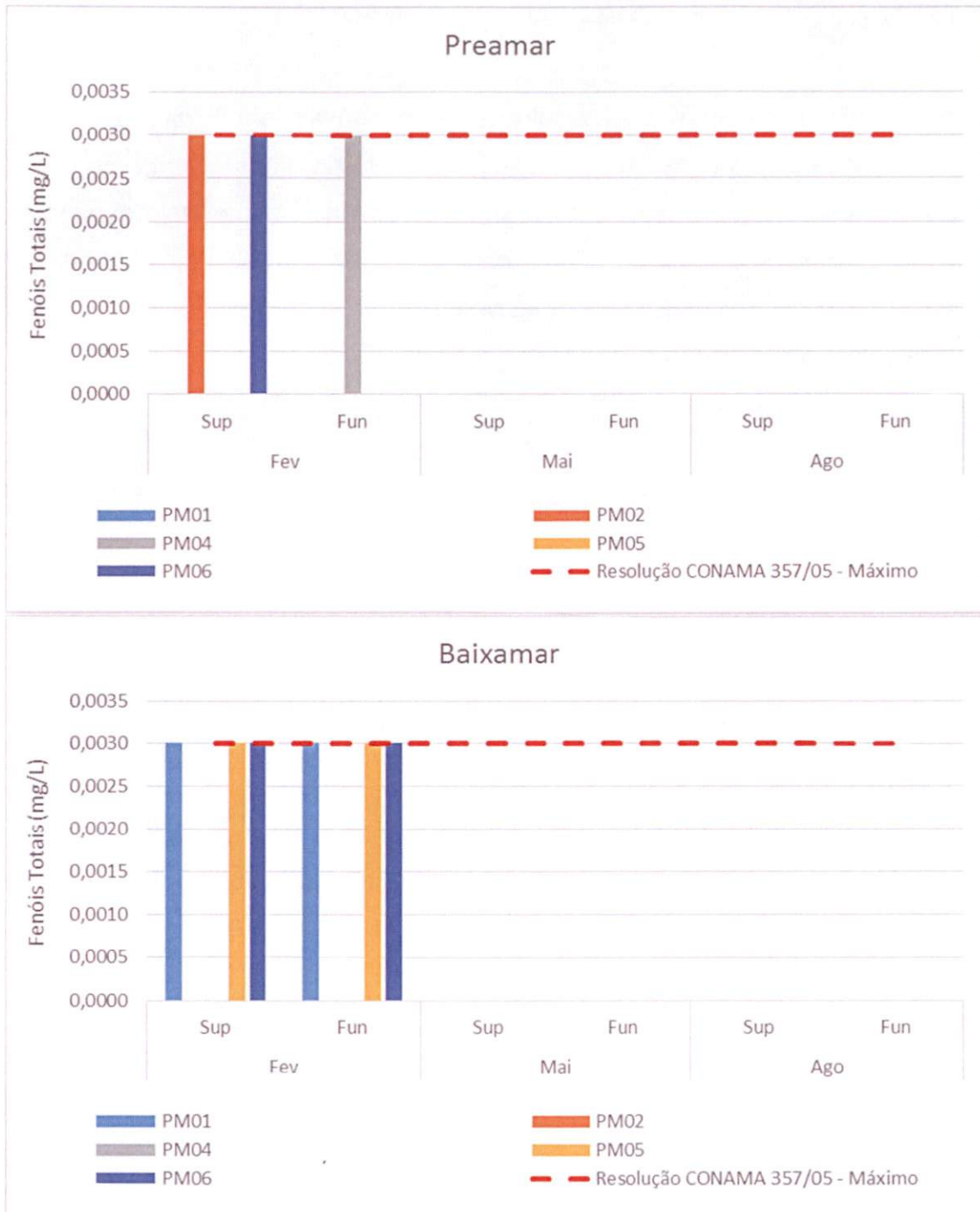
Gráfico 5-25: Valores de fenóis totais das estações do rio Barra Nova nas profundidades de superfície e fundo sob condição de preamar e baixamar ao longo das campanhas de monitoramento.
