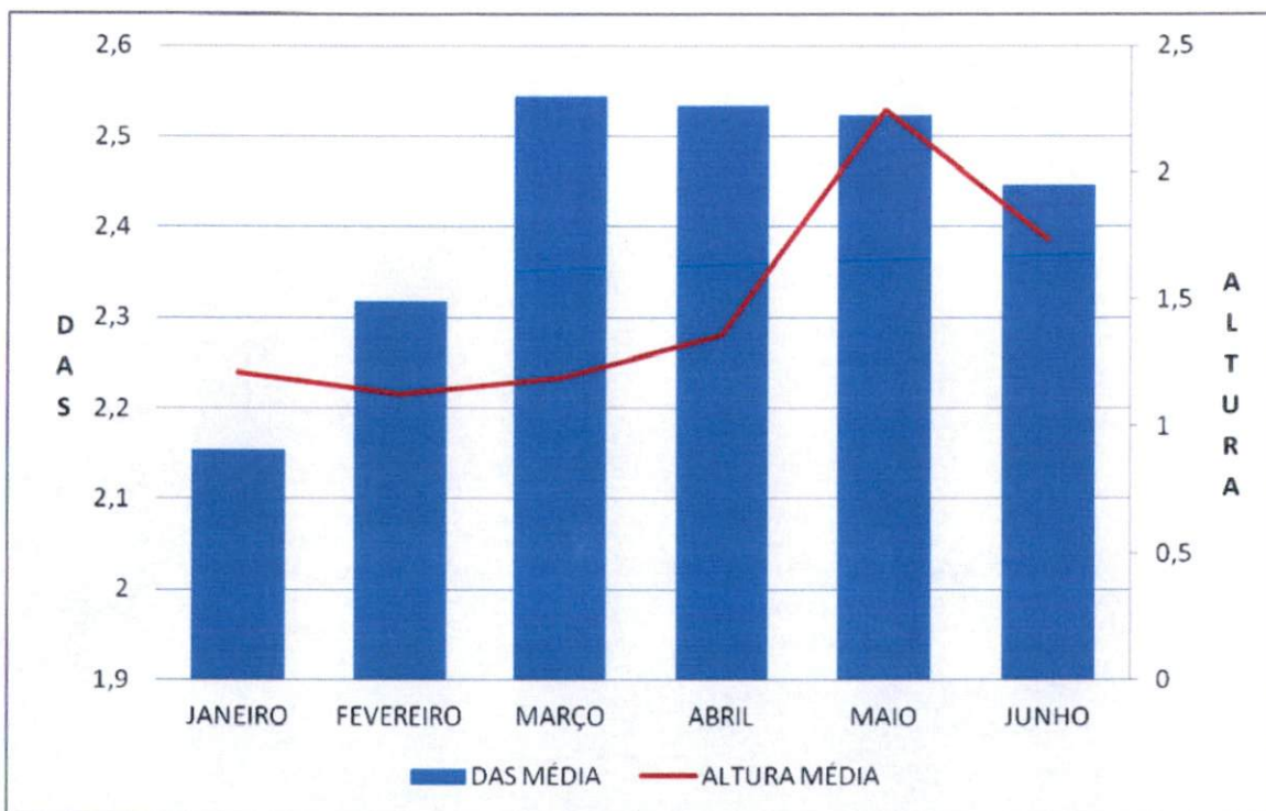
Gráfico 1: Dados dendrométricos médios levantados entre os meses de janeiro a junho de 2015. DAS Média – Diâmetro Médio na Altura do Solo, em centímetros e Altura Média em metros.
