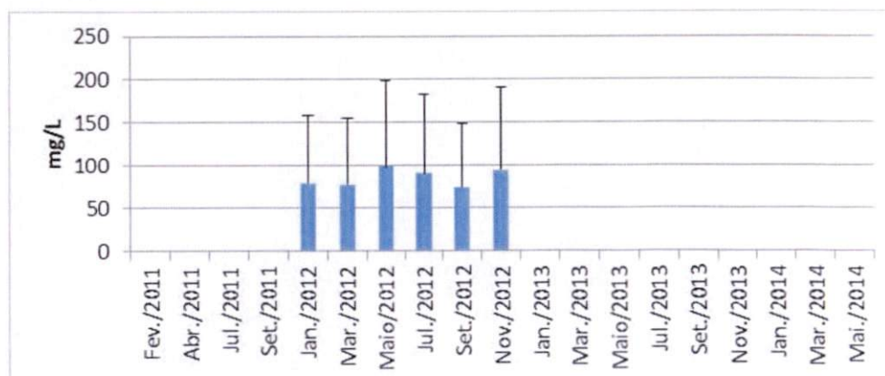
Figura 7-23: Valores de óleo vegetais (mg/L) ao longo das estações de monitoramento, na temporada de 2011 a 2014.
