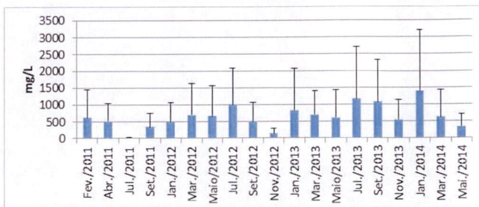
Figura 7-5: Valores de DBO (mg/L) ao longo das campanhas de monitoramento, na temporada de 2011 a 2014.
