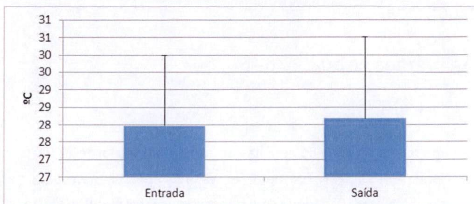
Figura 7-2: Valores de temperatura, em graus Celsius (°C), ao longo das estações de monitoramento, entre os pontos de coleta, na temporada de 2011 a 2014.
