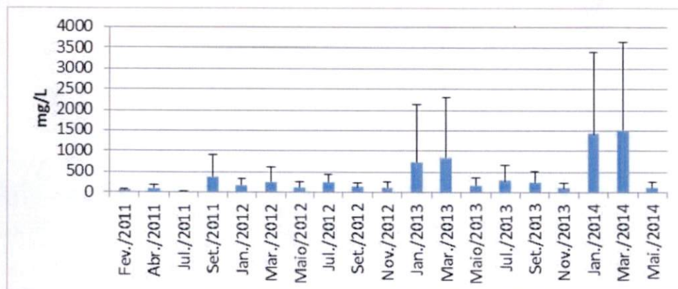
Figura 7-17: Valores de sólidos dissolvidos totais (mg/L) ao longo das campanhas de monitoramento, na temporada de 2011 a 2014.
