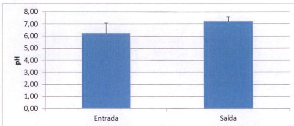
Figura 7-4: Valores obtidos para pH ao longo das estações de monitoramento, entre os pontos de coleta, na temporada de 2011 a 2014.
