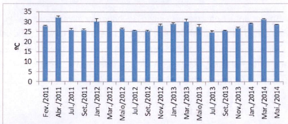
Figura 7-1: Valores de temperatura, em graus Celsius (°C), ao longo das campanhas de monitoramento, na temporada de 2011 a 2014.
