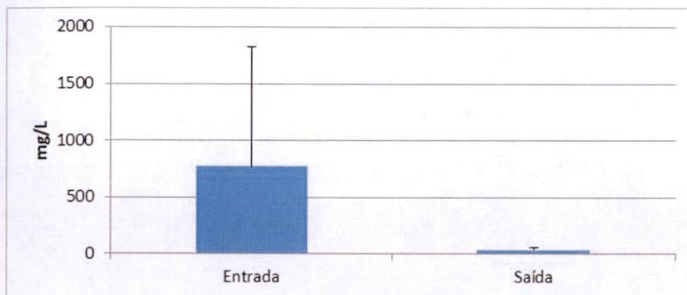
Figura 7-16: Valores de sólidos suspensos totais (mg/L) ao longo das estações de monitoramento, entre os pontos de coleta, na temporada de 2011 a 2014.
