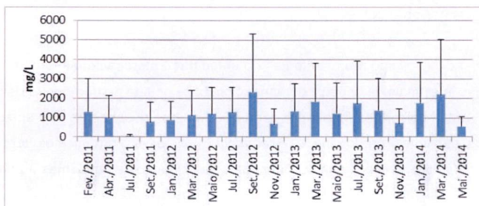
Figura 7-7: Valores de DQO (mg/L) ao longo das campanhas de monitoramento, na temporada de 2011 a 2014.
