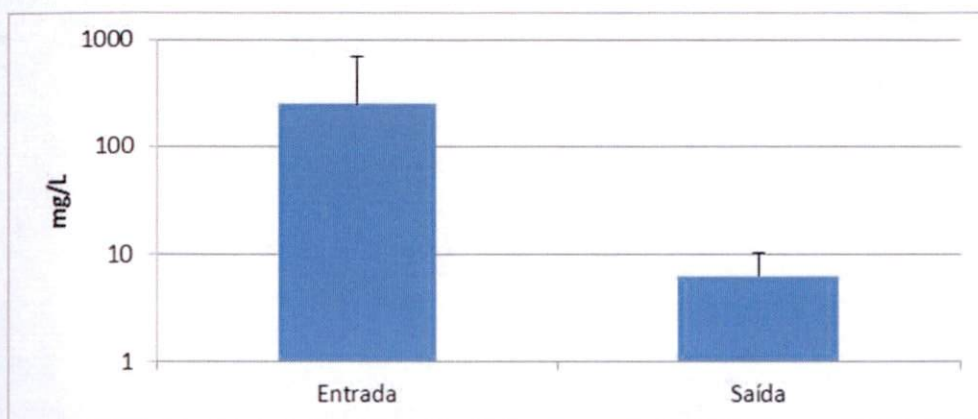
Figura 7-12: Valores de concentração na superfície, em miligramas por litro (mg/L) de óleos e graxas ao longo das estações de monitoramento, entre os pontos de coleta, na temporada de 2011 e 2014.
