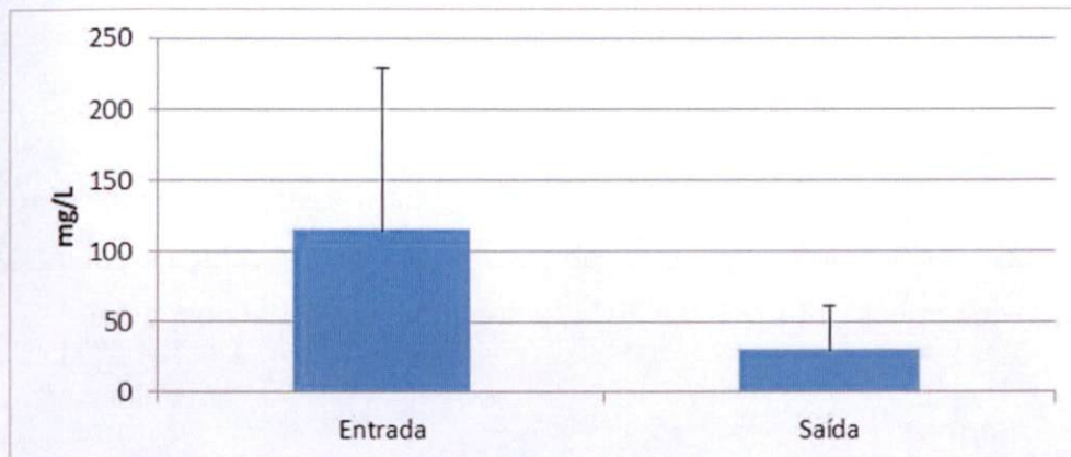
Figura 7-24: Valores de óleo vegetais (mg/L) ao longo das estações de monitoramento, entre os pontos de coleta, na temporada de 2011 a 2014.
