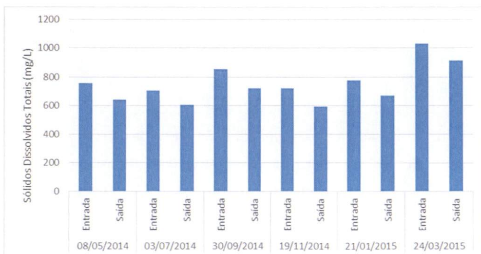
Gráfico 6-6: Valores de sólidos dissolvidos totais ao longo das campanhas de monitoramento da ETE.
