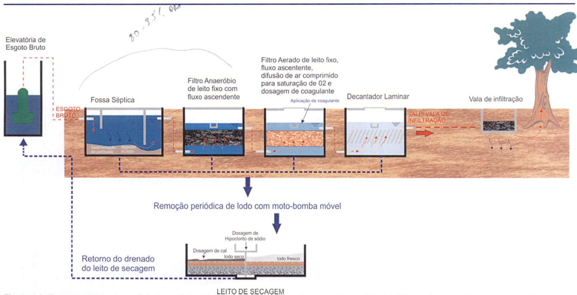
Figura 4-1: Fluxograma das etapas de tratamento implantada no Terminal Norte Capixaba. Fonte: Relatório Técnico Anual do Monitoramento da Estação de Tratamento de Esgoto Sanitário Instalada no Terminal Norte Capixaba (TNC) - Ano de 2011.
