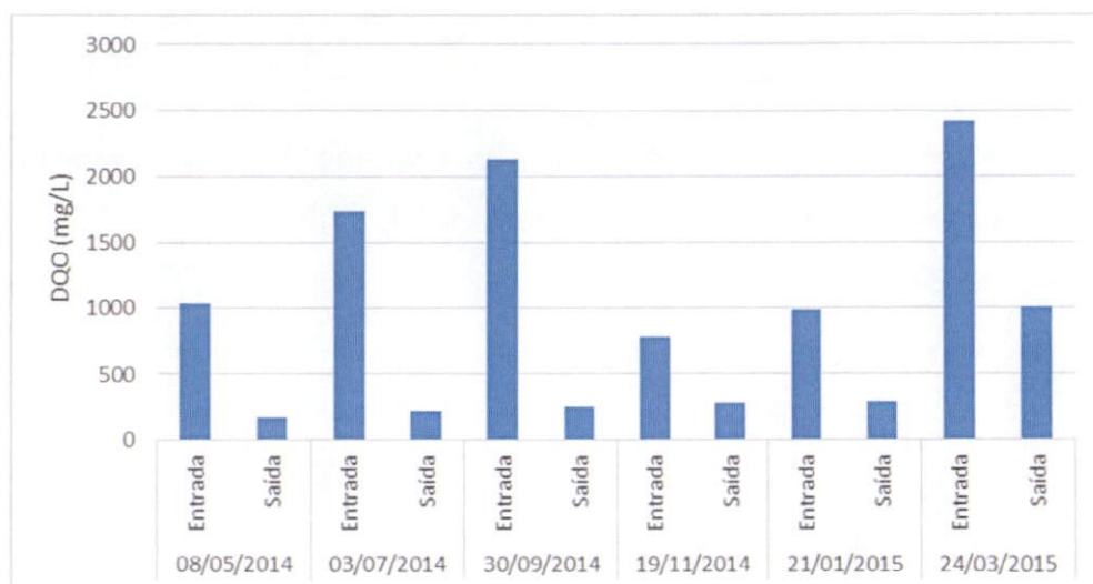
Gráfico 6-3: Valores de DQO ao longo das campanhas de monitoramento da ETE.
