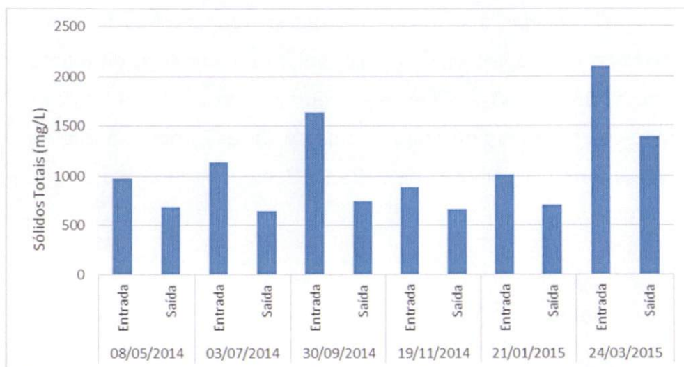
Gráfico 6-8: Valores de sólidos totais ao longo das campanhas de monitoramento da ETE.
