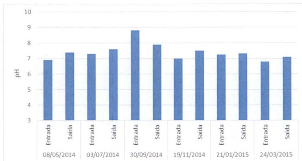
Gráfico 6-1: Valores de pH ao longo das campanhas de monitoramento da ETE.
