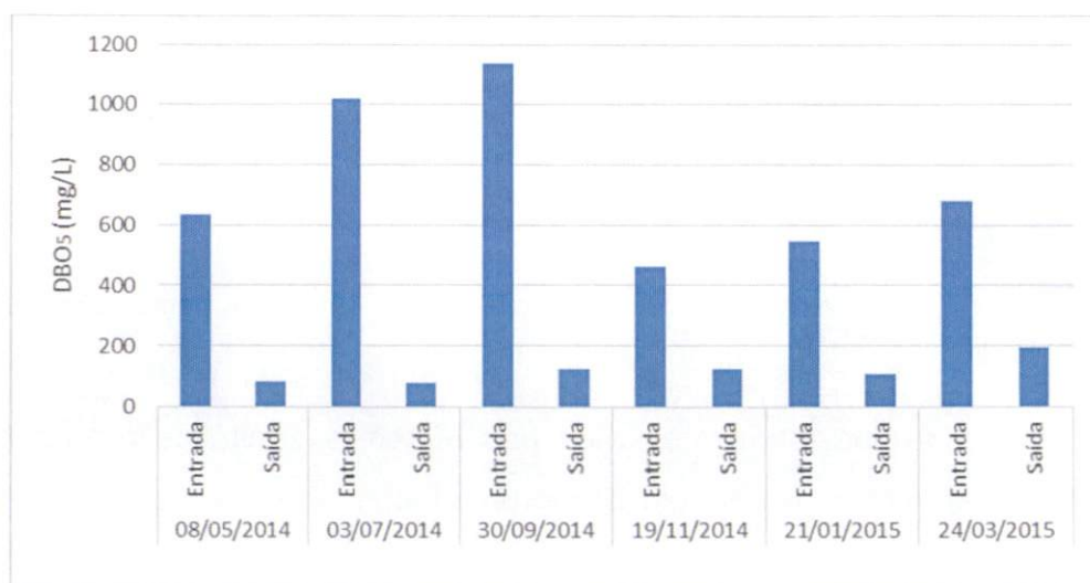
Gráfico 6-4: Valores de DBO5 ao longo das campanhas de monitoramento da ETE.
