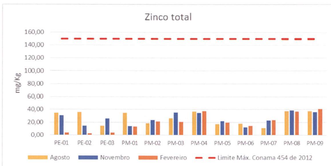
Gráfico 5-5: Concentração de Zinco Total no sedimento estuarino e marinho nas campanhas de agosto e novembro de 2013 e fevereiro de 2014.
