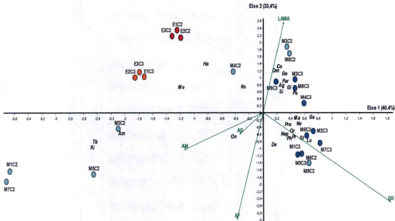
Figura V.1.2 - 5 - Análise de Correlação Canônica (CCA) entre os dados de granulometria e abundância dos principais organismos (fauna total – Campanha 02 e 85% indivíduos – Campanha 03) do zoobentos de fundo inconsolidado na área de influência do Terminal Norte Capixaba. (Legenda: AF – areia fina, AM – areia média, AG – areia grossa, GR – grânulo; LAMA – lama. Estuário: ● Camp 03 e ● Camp 02; Marinho ● - Camp 03 e ● - Camp 02. Pontos estuarinos – E; pontos marinhos - M; * - espécies encontradas; → - fatores edáficos (granulometria).
