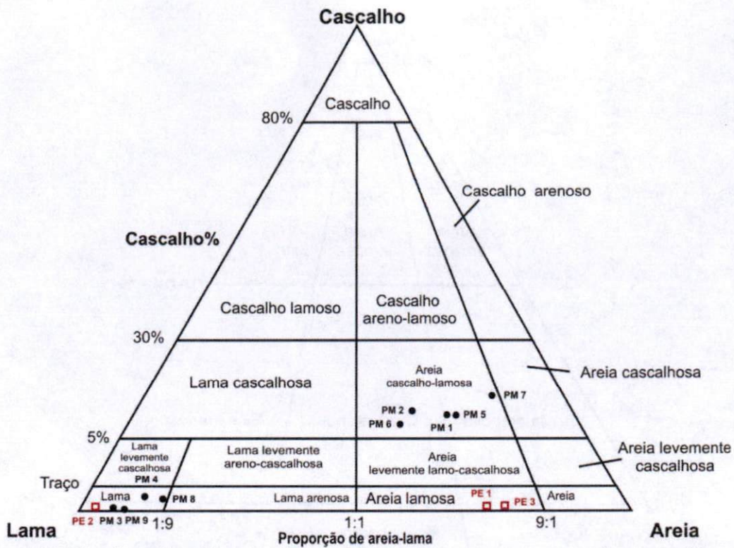
Figura V.2.2 – 2 - Classificação dos sedimentos de acordo com o diagrama triangular Lama-Areia-Cascalho.
