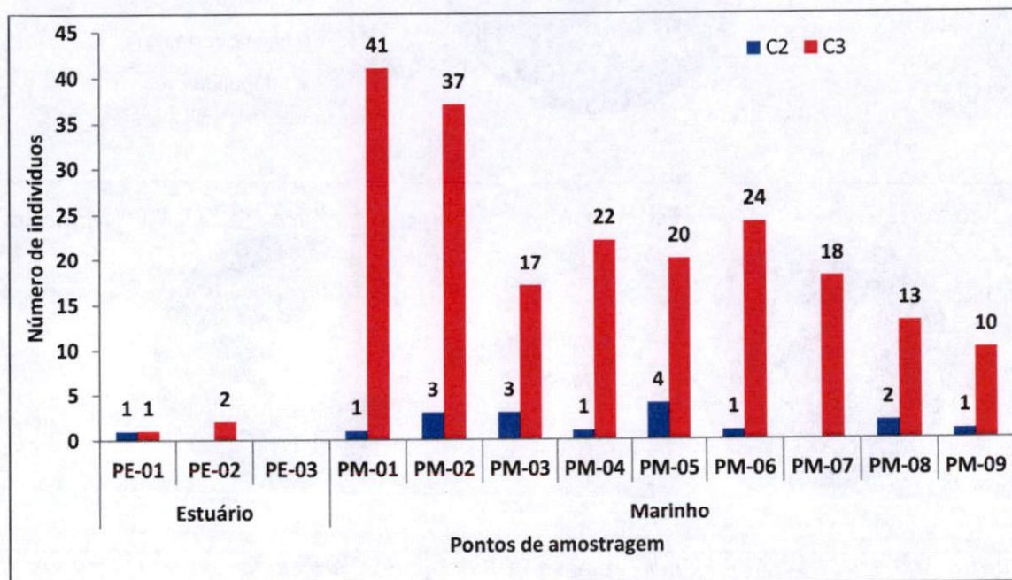
Figura V.1.1 – 2 – Número total de indivíduos coletado ao longo dos 12 pontos amostrais na Área de Influência do Terminal Norte Capixaba (dezembro/2011 (c1) e março/2012 (c2)).
