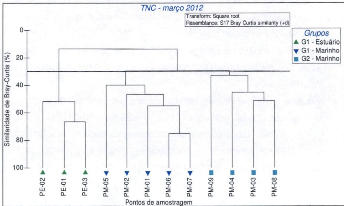
Figura V.1.2 – 3 – Valores da análise multivariada da comunidade entre as duas campanhas (dezembro/2011 e março/2012) MDS (a), e a distribuição para a segunda campanha (MDS – b; e Cluster- c) entre os 12 pontos amostrais na área de influência do Terminal Norte Capixaba (março/2012).
