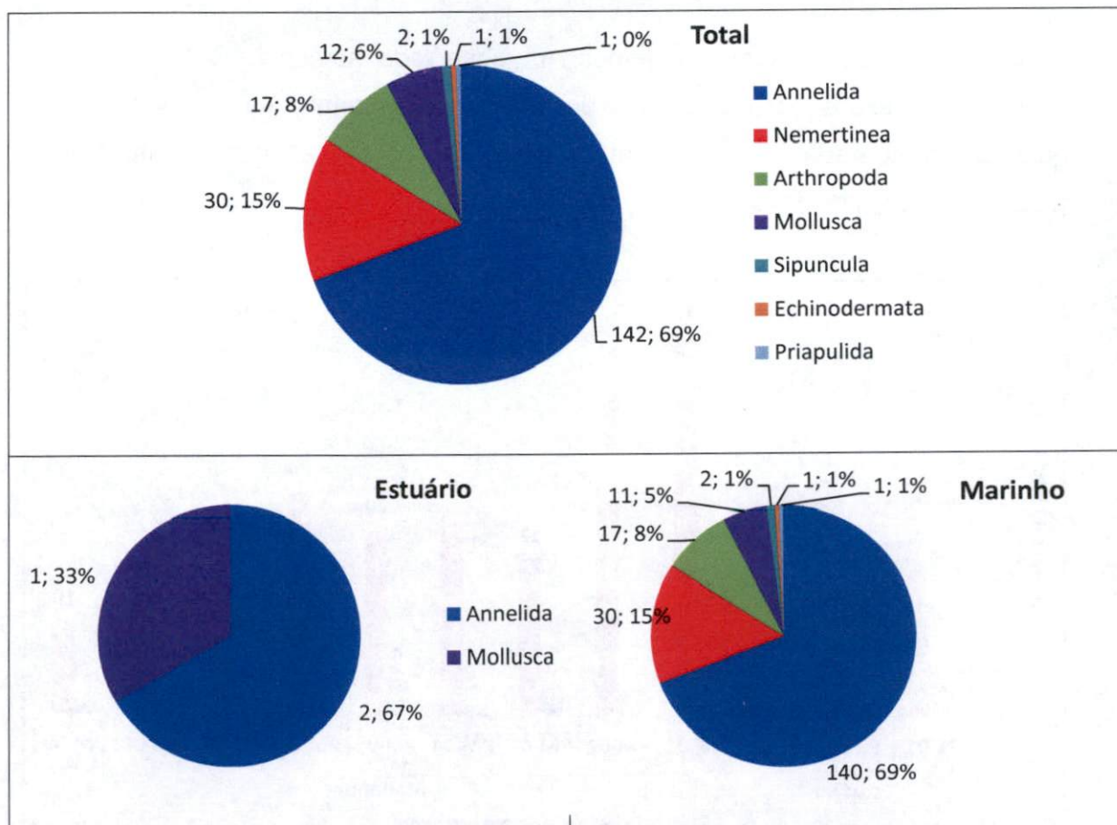
Figura V.1.1 - 1 – Abundância relativa (%) total dos principais grandes grupos de organismos da comunidade bentônica associada ao sedimento marinho e estuarino da Área de Influência do Terminal Norte Capixaba que ocorreram nos 12 pontos amostrais (março/2012 – campanha 03).
