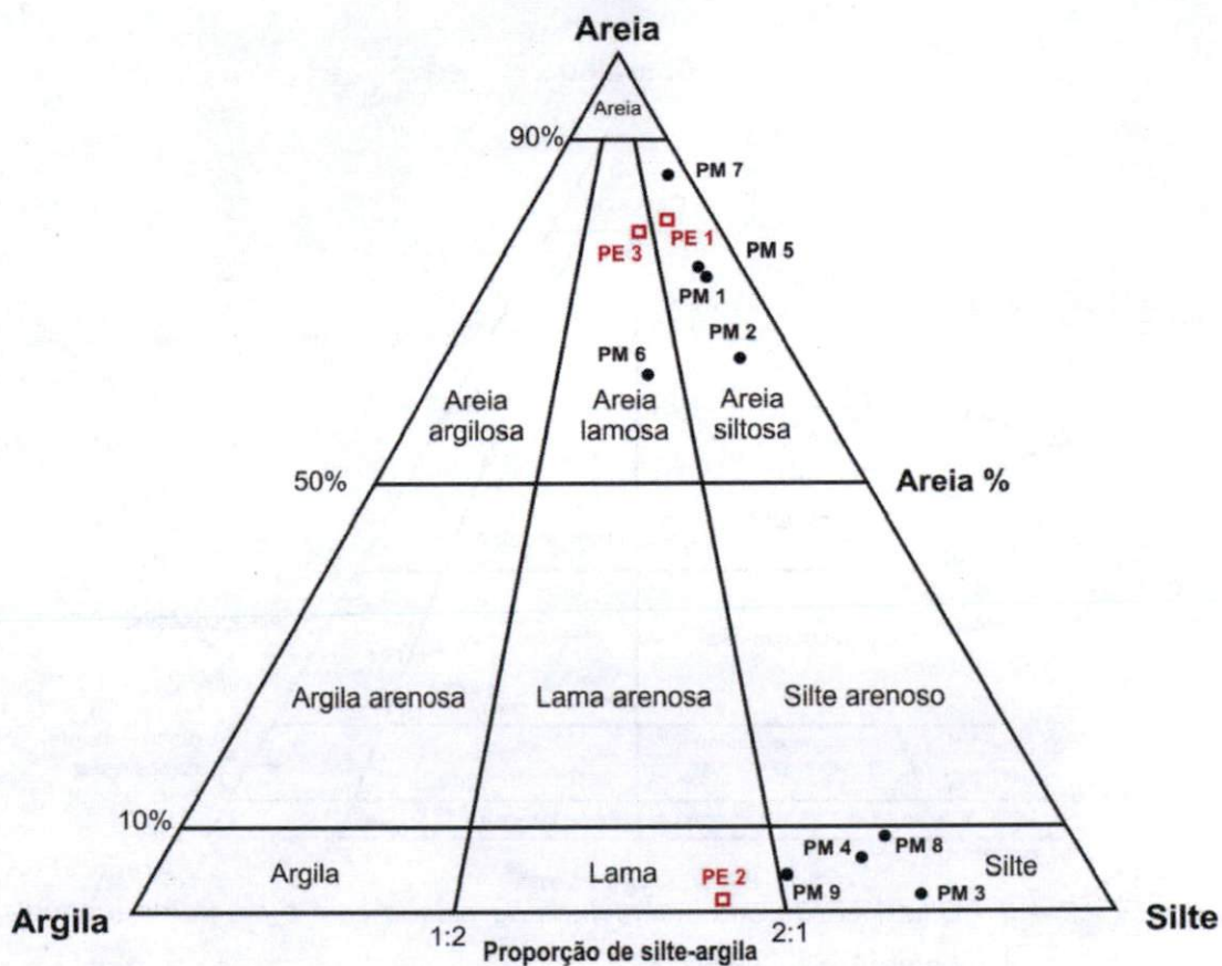
Figura V.2.2 – 1 - Classificação dos sedimentos de acordo com o diagrama triangular Argila-Silte-Areia.
