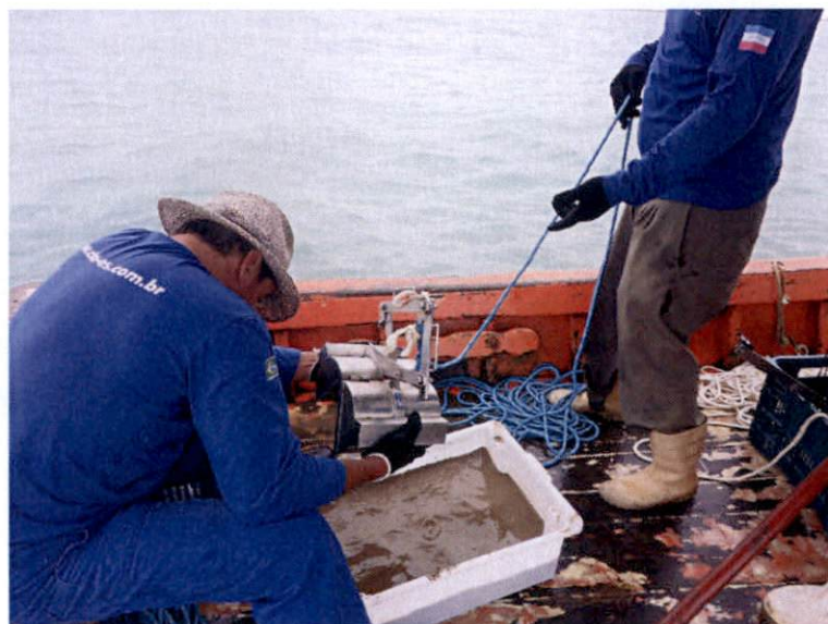
Figura 4-1: Demonstração da coleta de sedimento com draga de Petersen .
