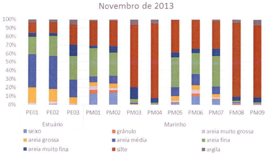
Gráfico 5-7: Granulometria do sedimento estuarino e marinho da campanha de Novembro de 2013.
