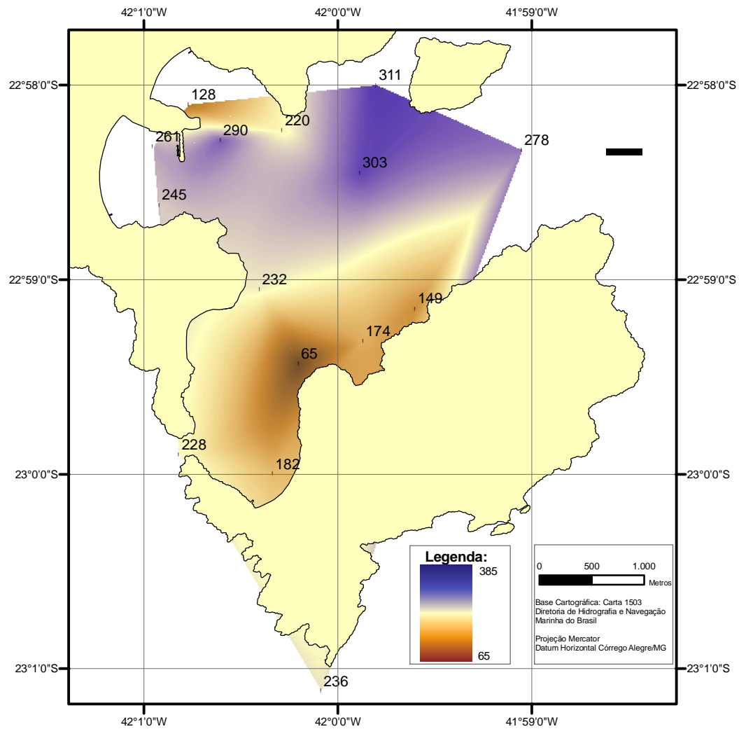
Figura 5.1.50: Distribuição dos valores de demanda química de oxigênio no fundo da Enseada dos Anjos.
