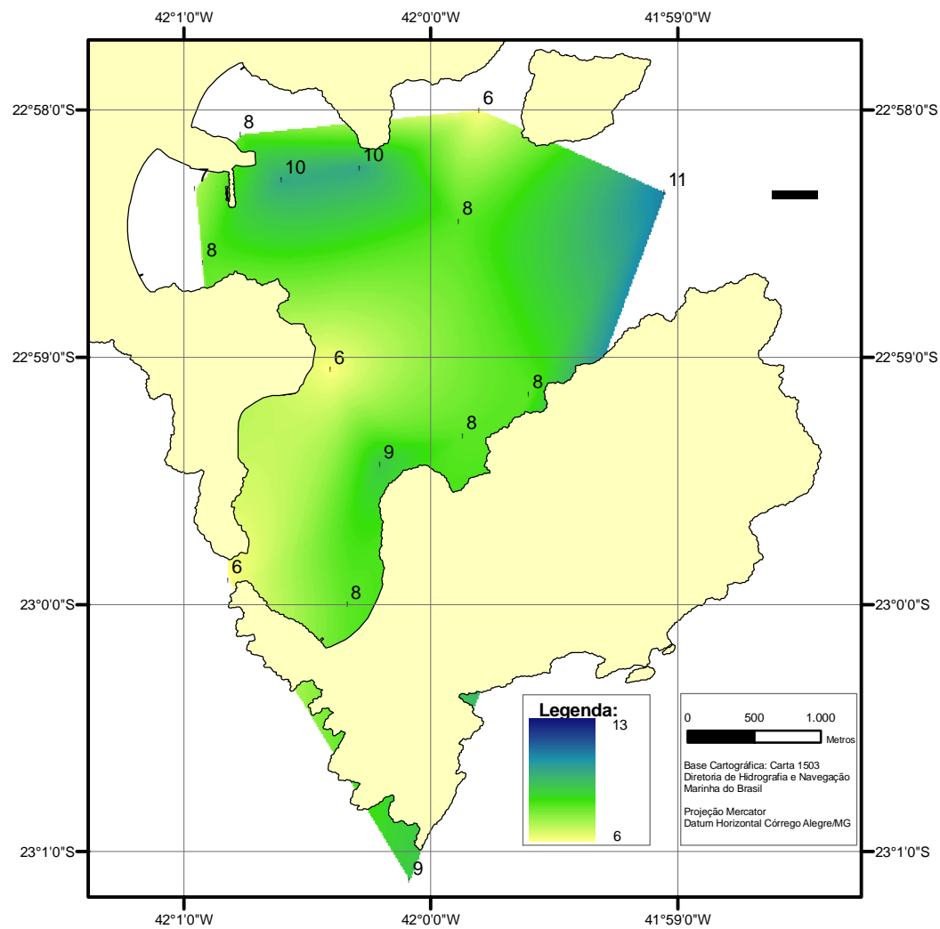
Figura 5.1.46: Distribuição das concentrações do carbono orgânico no fundo da Enseada dos Anjos
