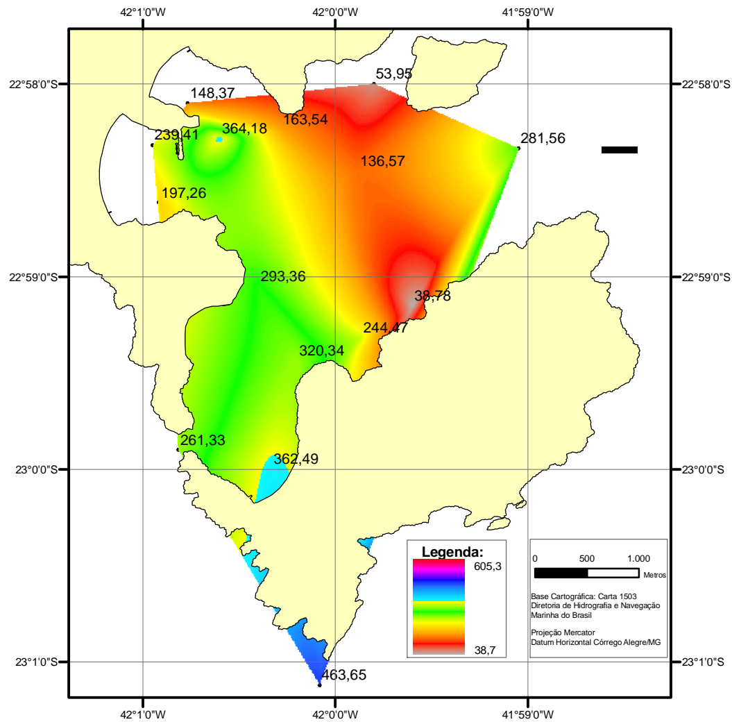
Figura 5.1.42: Distribuição das concentrações de nitrogênio total no fundo da Enseada dos Anjos.
