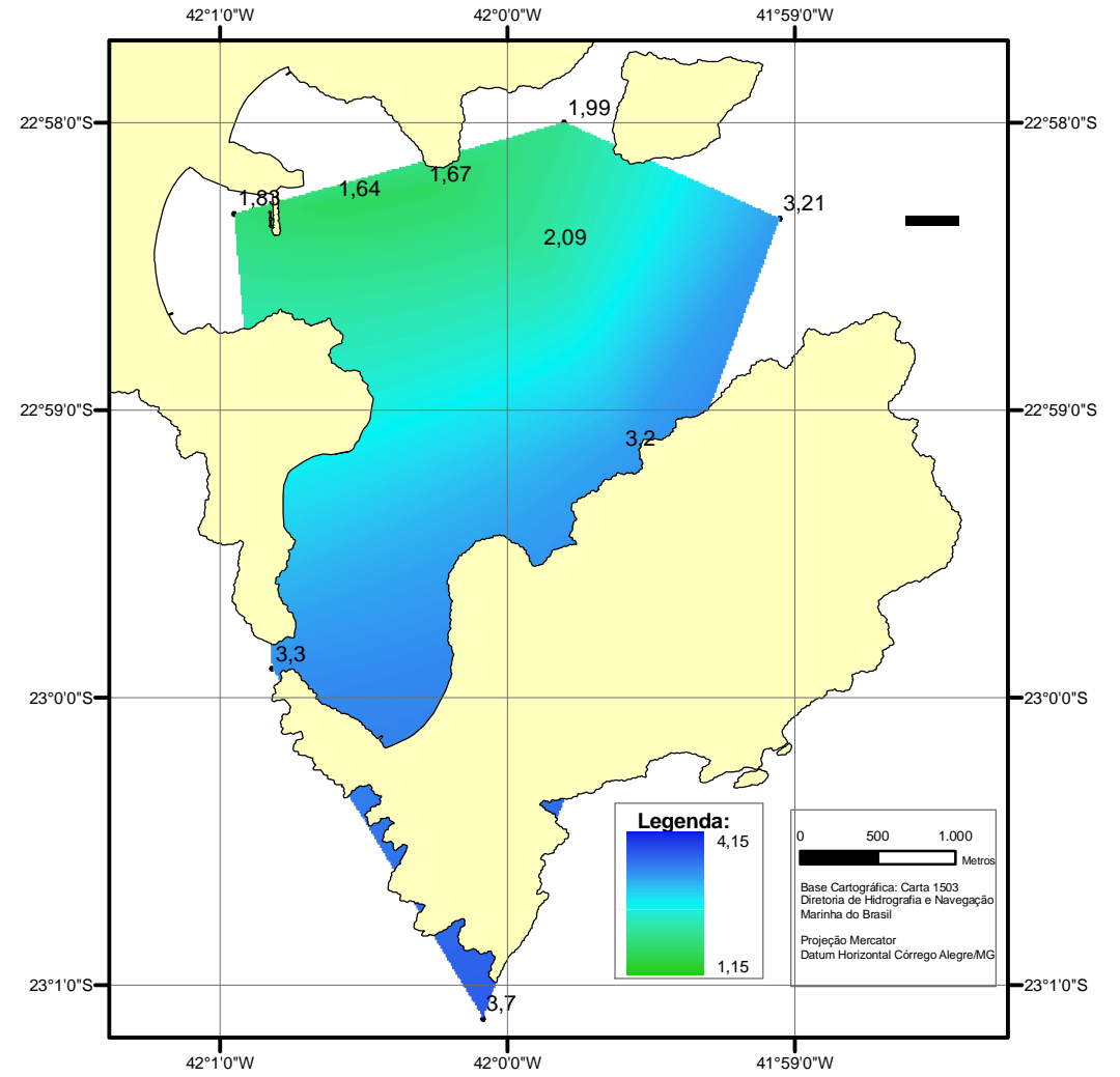
Figura 5.1.39: Distribuição das concentrações de clorofila-a na superfície e meia água da Enseada dos Anjos
