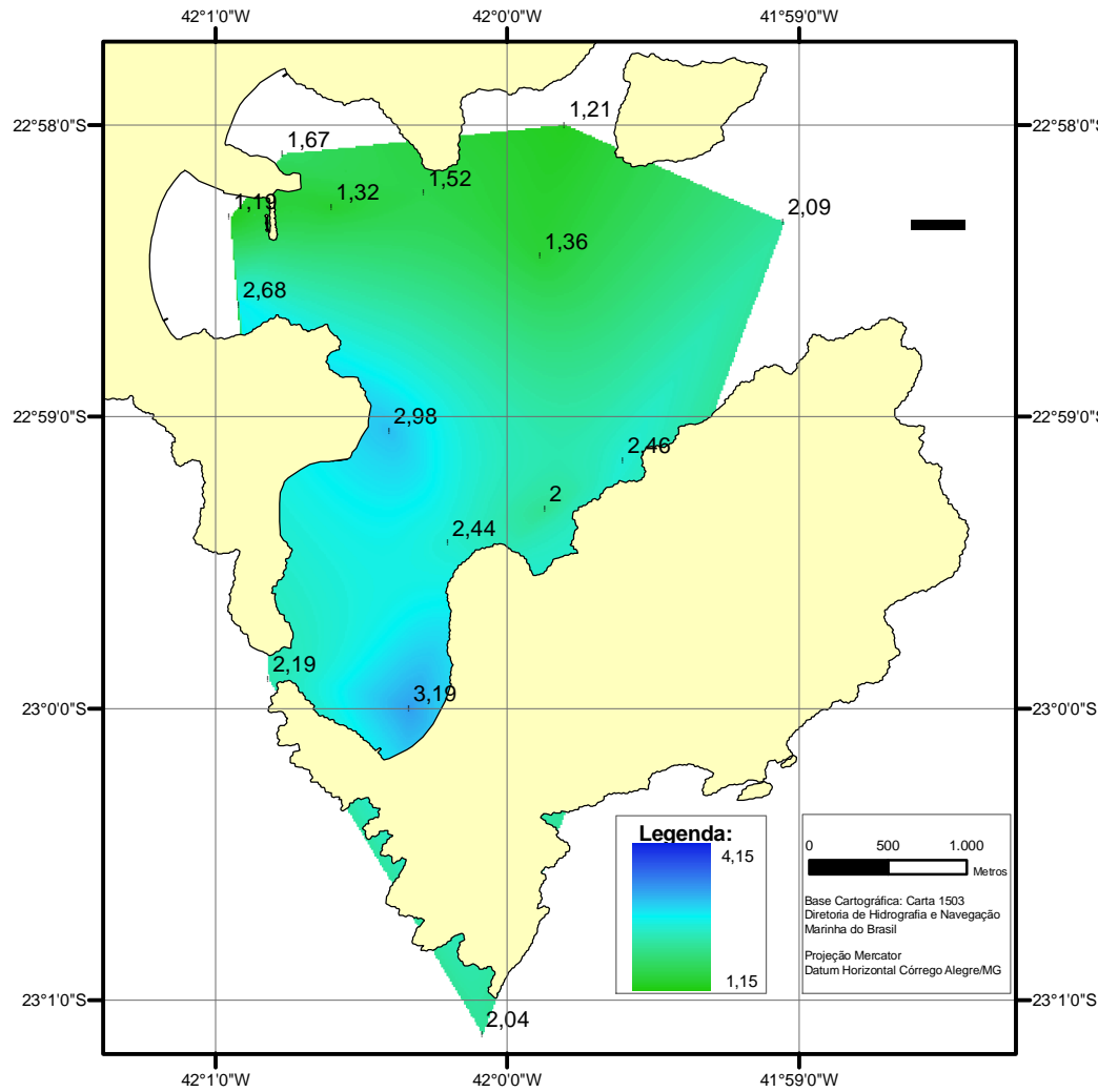
Figura 5.1.39: Distribuição das concentrações de clorofila-a na superfície e meia água da Enseada dos Anjos
