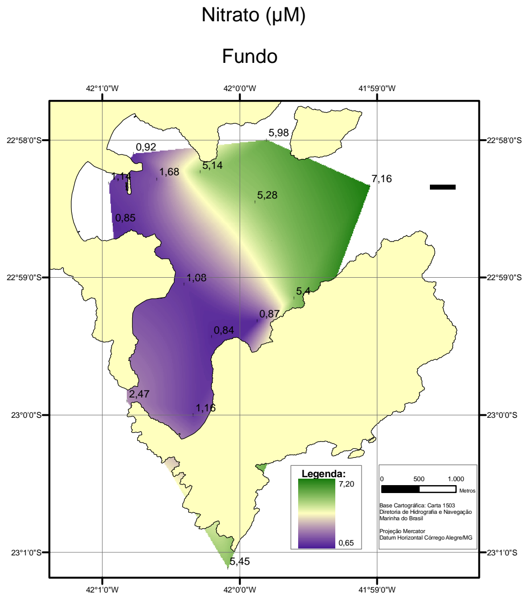
Figura 5.1.34: Distribuição das concentrações de nitrato no fundo da Enseada dos Anjos.
