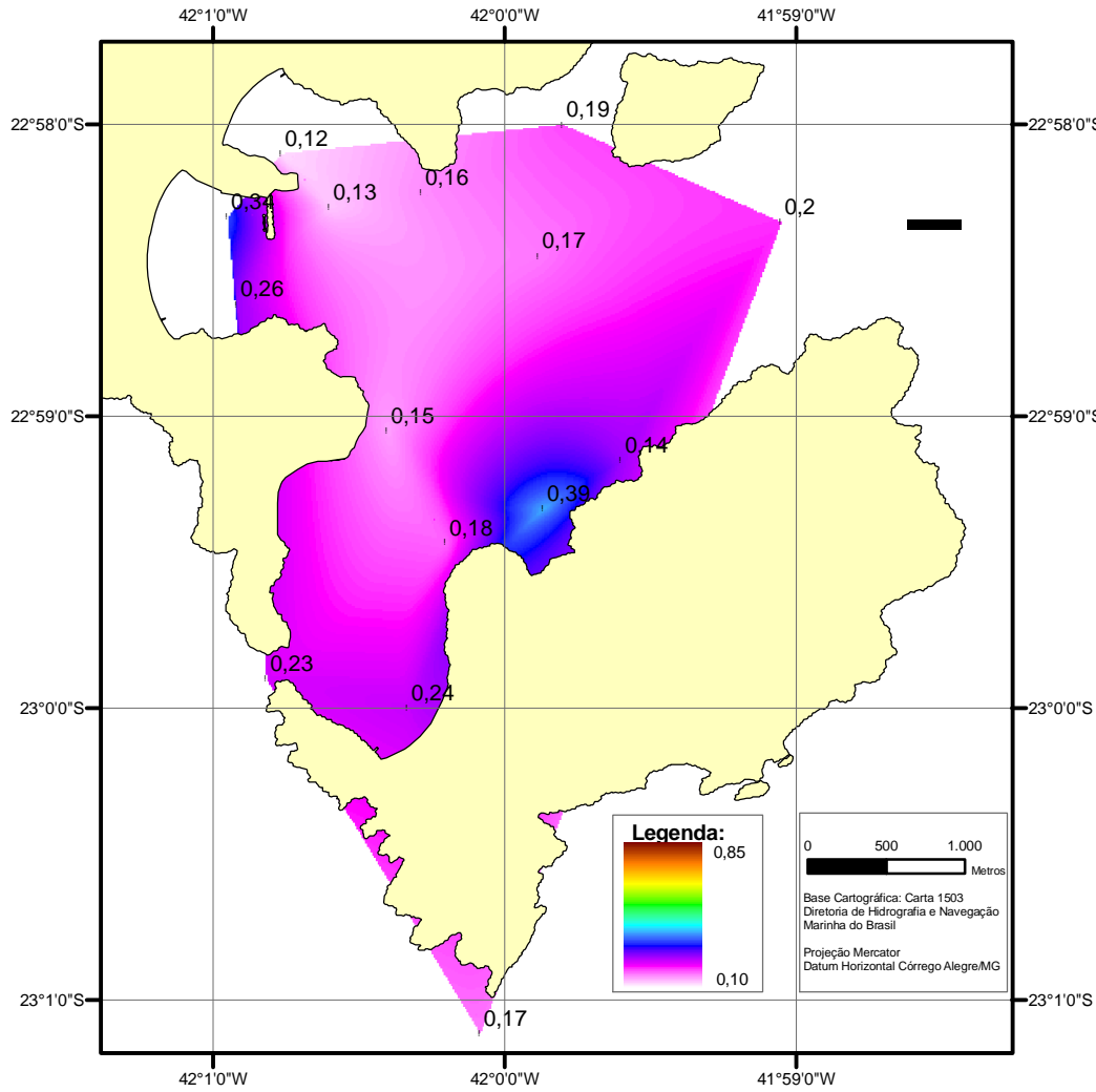
Figura 5.1.31: Distribuição das concentrações de fosfato na superfície e meia água da Enseada dos Anjos
