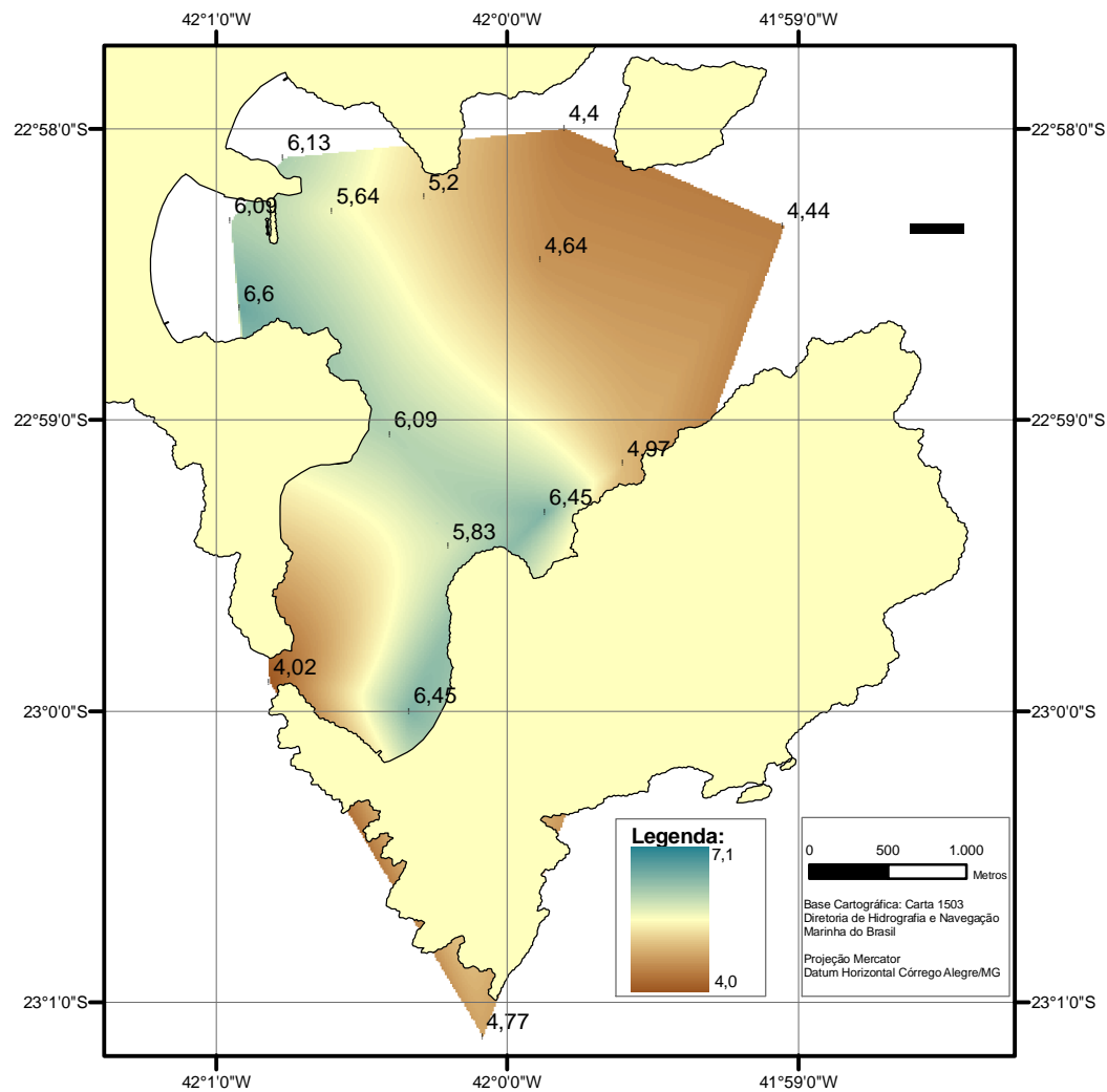
Figura 5.1.25: Distribuição das concentrações de oxigênio dissolvido no fundo da Enseada dos Anjos.
