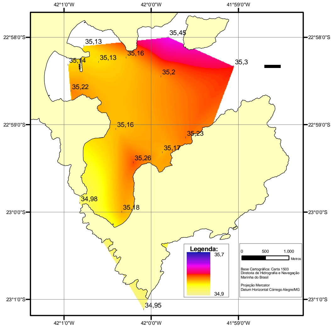
Figura 5.1.22: Distribuição dos valores de salinidade na superfície e meia água da Enseada dos Anjos
