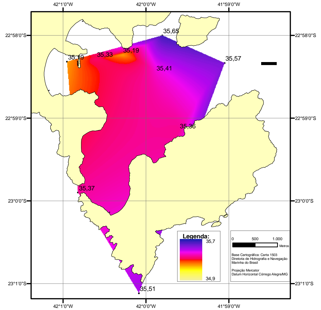
Figura 5.1.22: Distribuição dos valores de salinidade na superfície e meia água da Enseada dos Anjos
