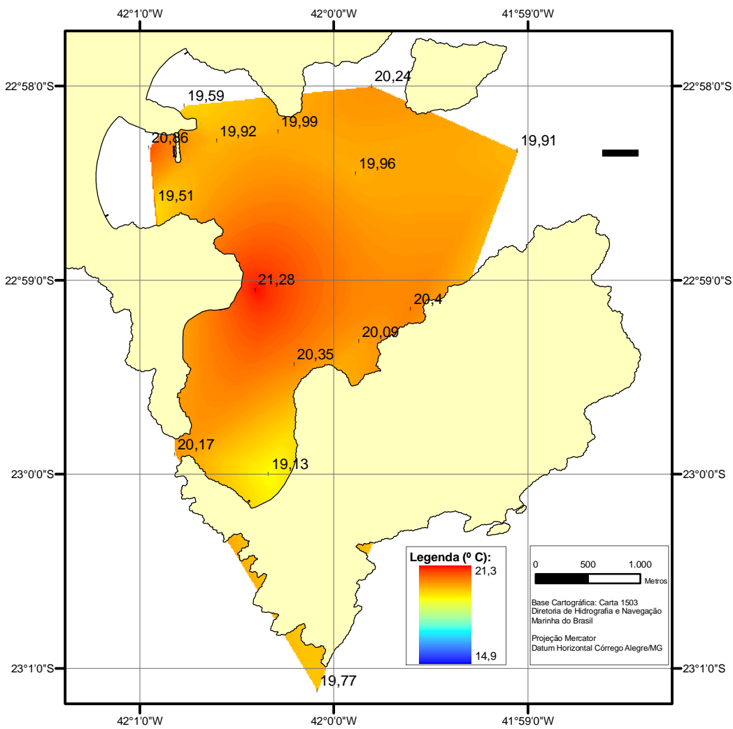
Figura 5.1.20: Distribuição dos valores de temperatura na superfície e meia água da Enseada dos Anjos
