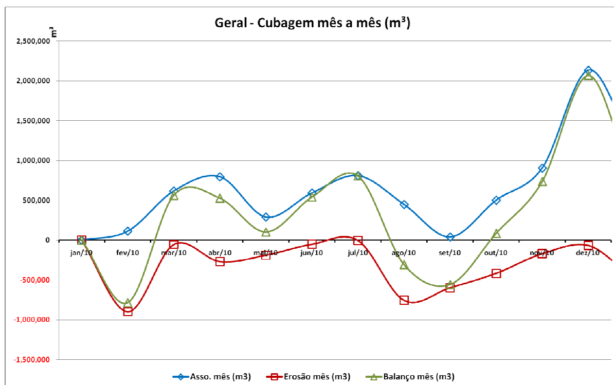
Figura I.6 - Curvas de volumes cubados (normalizados) no projeto em cada mês a partir de janeiro comparado ao mês imediatamente anterior.
