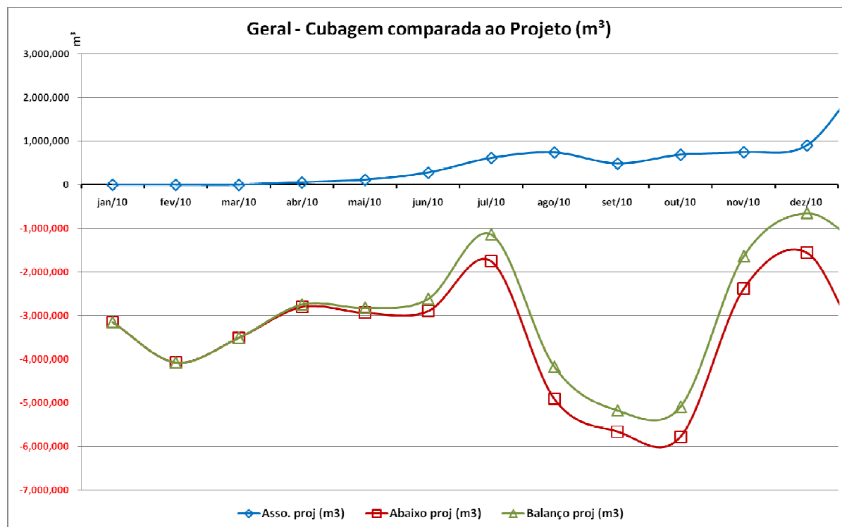
Figura I.4 - Curvas de volumes cubados (normalizados) no projeto em cada mês a partir de janeiro frente o projeto.
