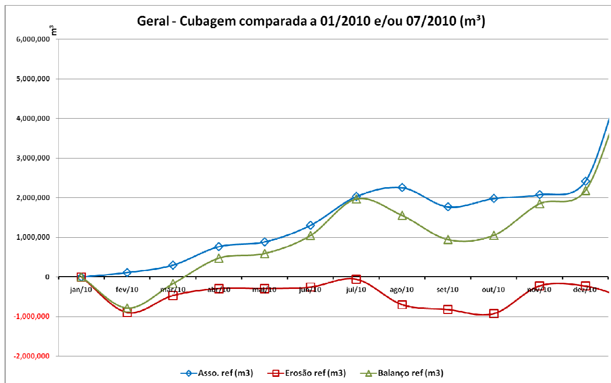
Figura I.5 - Curvas de volumes cubados (normalizados) no projeto em cada mês a partir de janeiro frente ao mês de referência (01/2010 para Trechos III, IV e V; 07/2010 para Trechos I e II).
