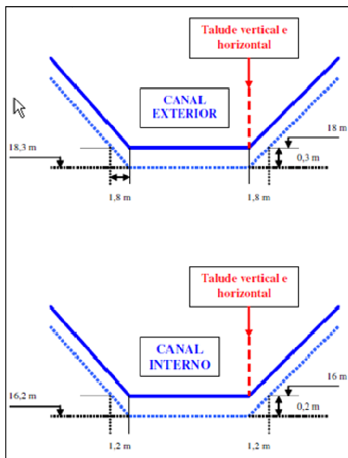
Figura I.2: Ilustração do critério adotado para cálculos dos volumes e das tolerâncias horizontal e vertical
