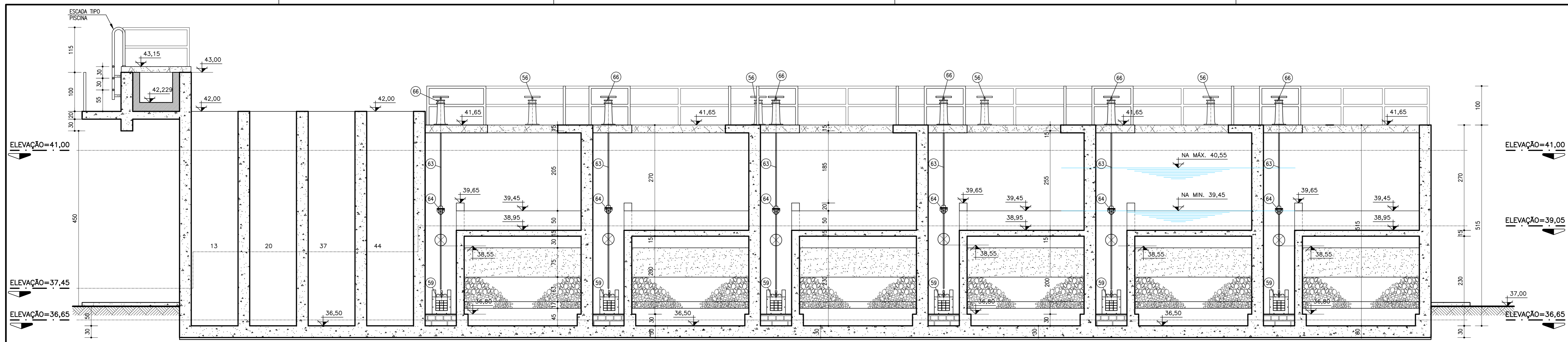
CORTE N-N
