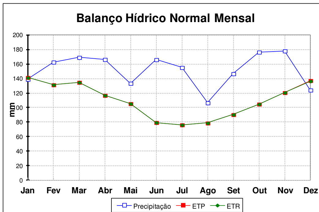
Figura 4.6 - Balanco Hídrico Climatológico – Método Thornthwaite & Mather (1955)
