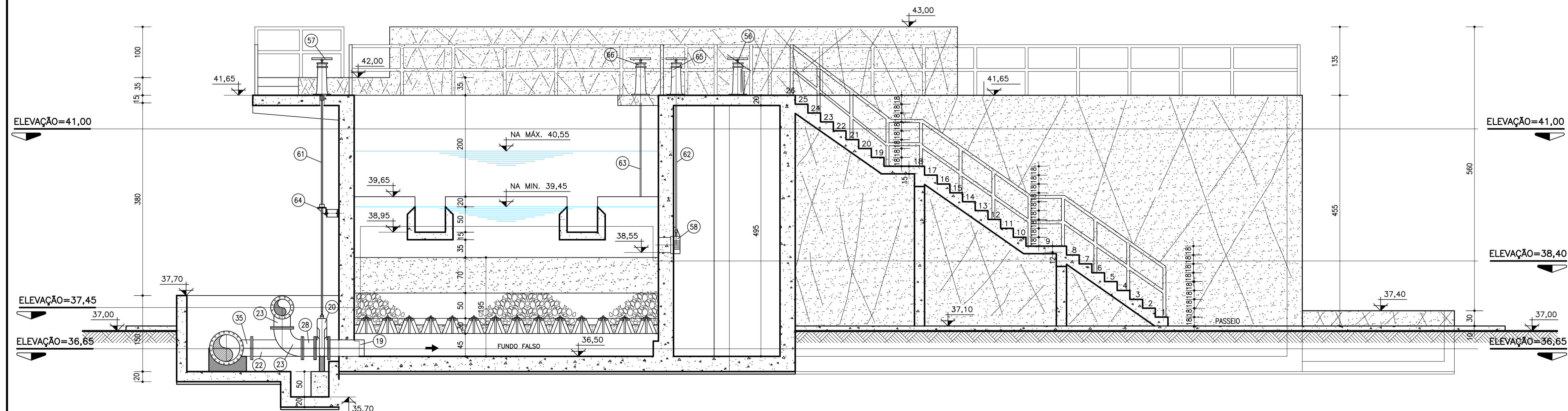
CORTE I-I ESC. 1:50
