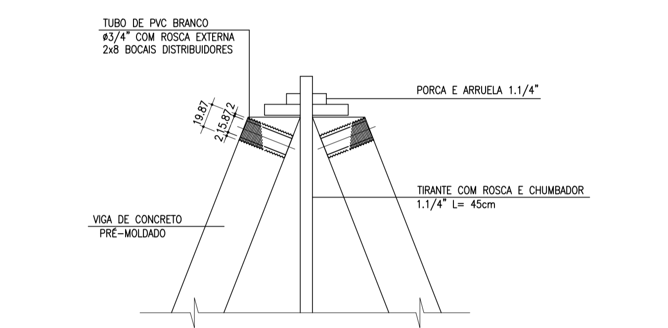
DETALHE F SEM ESCALA (DIMENSÕES EM MILÍMETROS)
