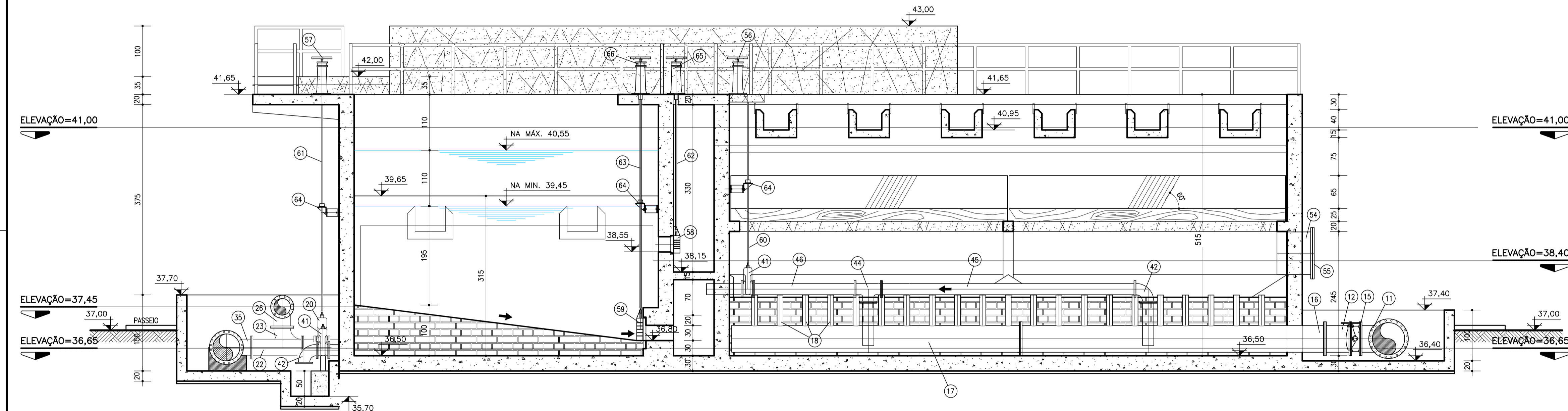
CORTE H-H ESC. 1:50
