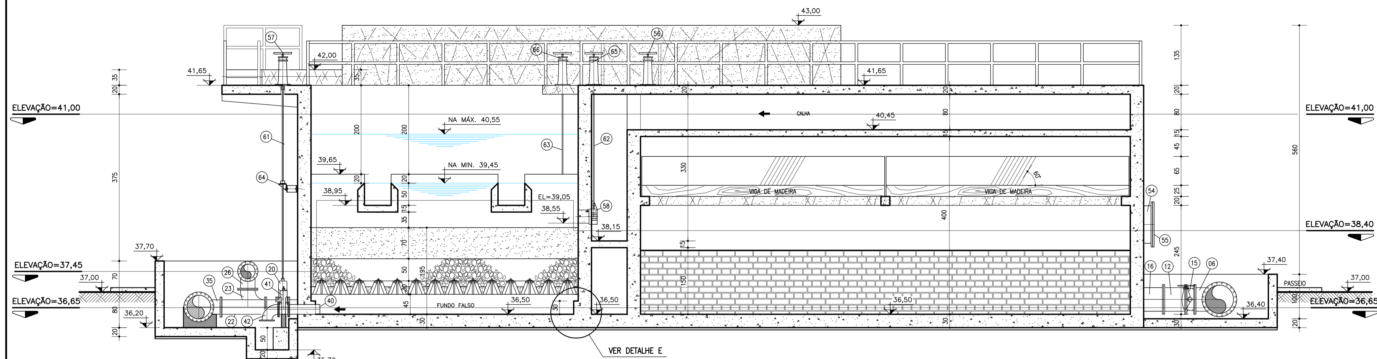
CORTE G-G ESC. 1:50
