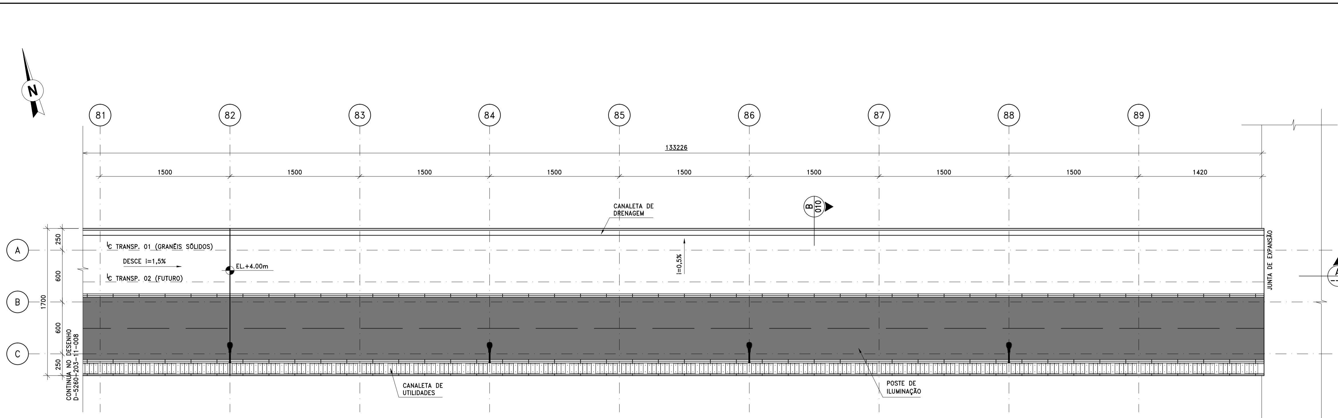
ARRANJO GERAL - TRECHO 09 ESCALA 1:250
