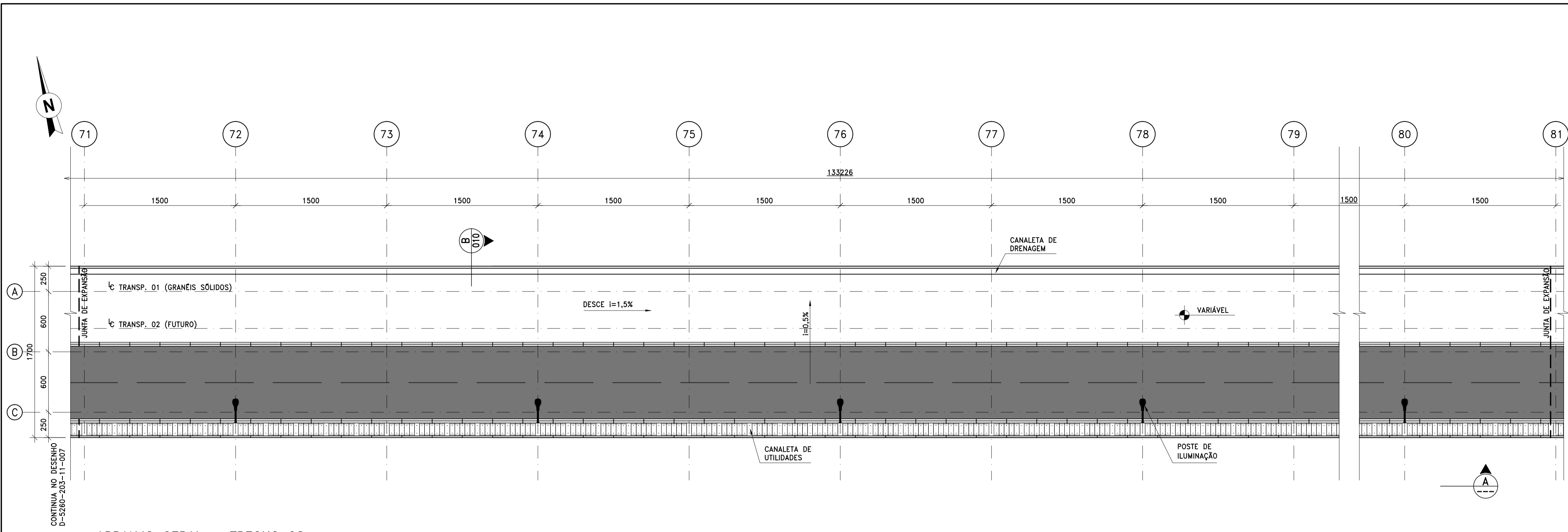
ARRANJO GERAL - TRECHO 08 ESCALA 1:250
