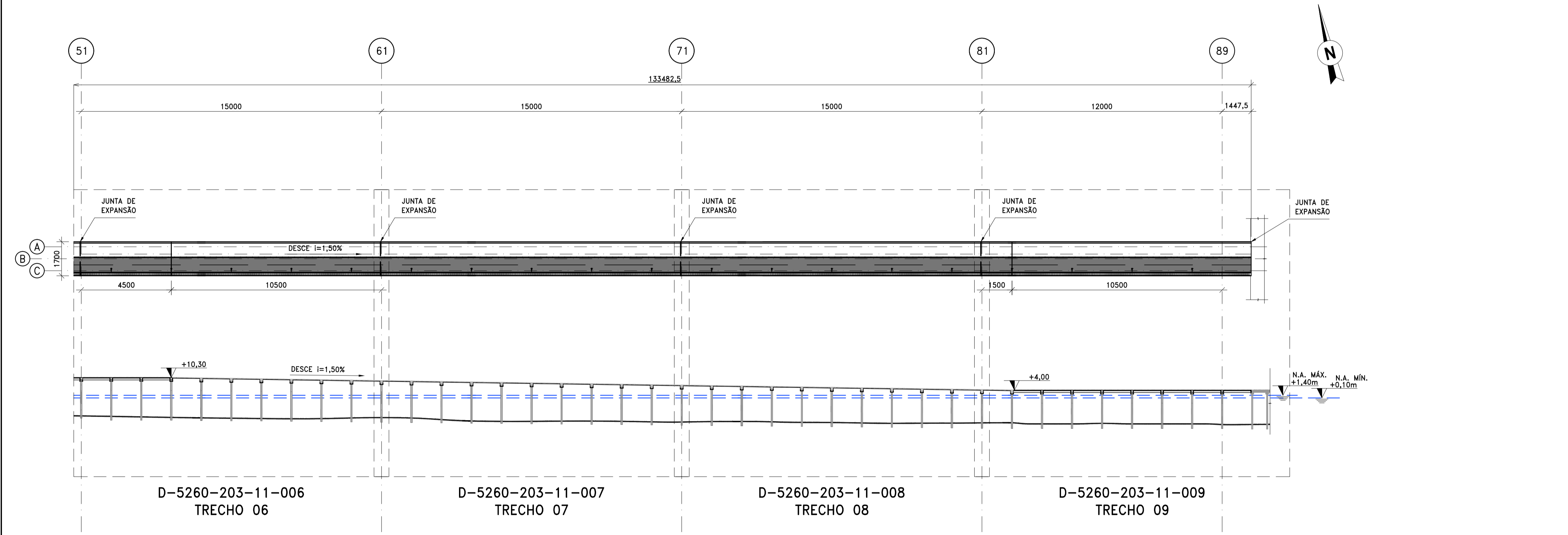
LAYOUT GERAL DA PONTE DE ACESSO ESCALA 1:250
