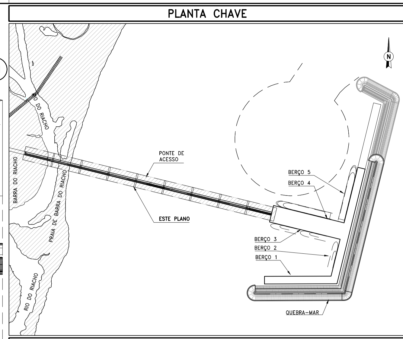
PLANTA CHAVE
