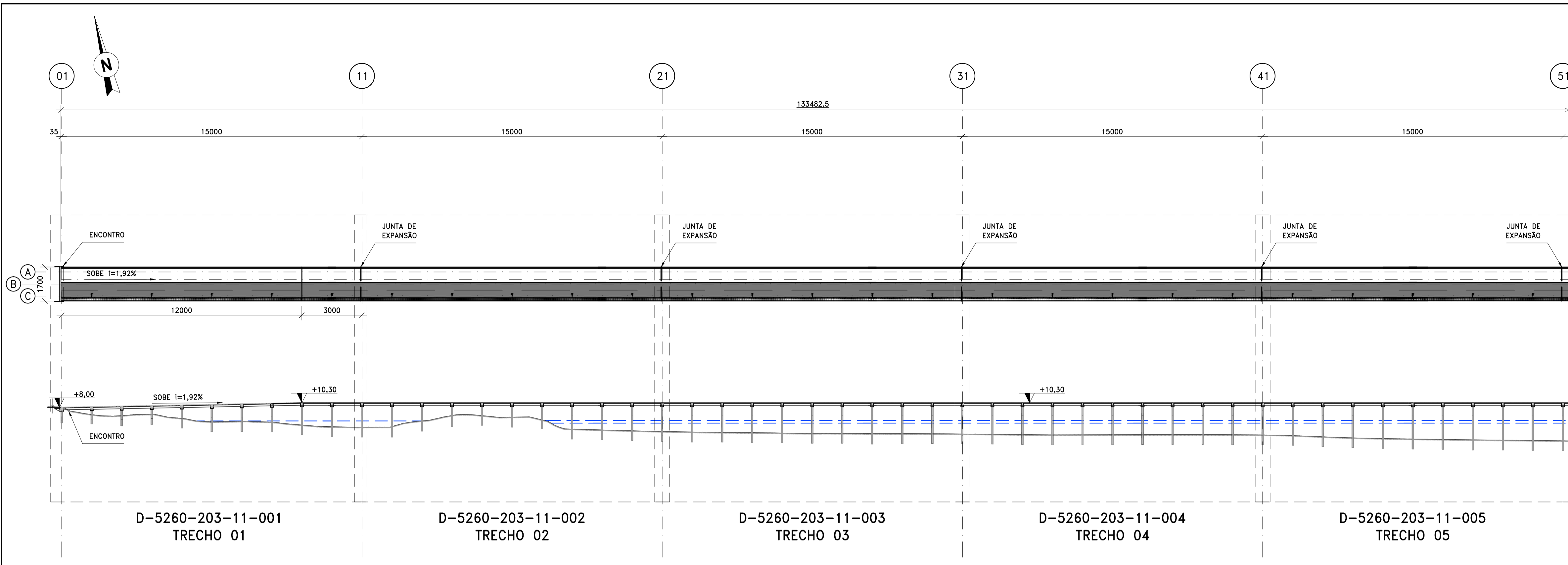
PLANTA CHAVE
