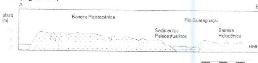
Figura 2.6 – Perfil topográfico transversal da planície costeira
