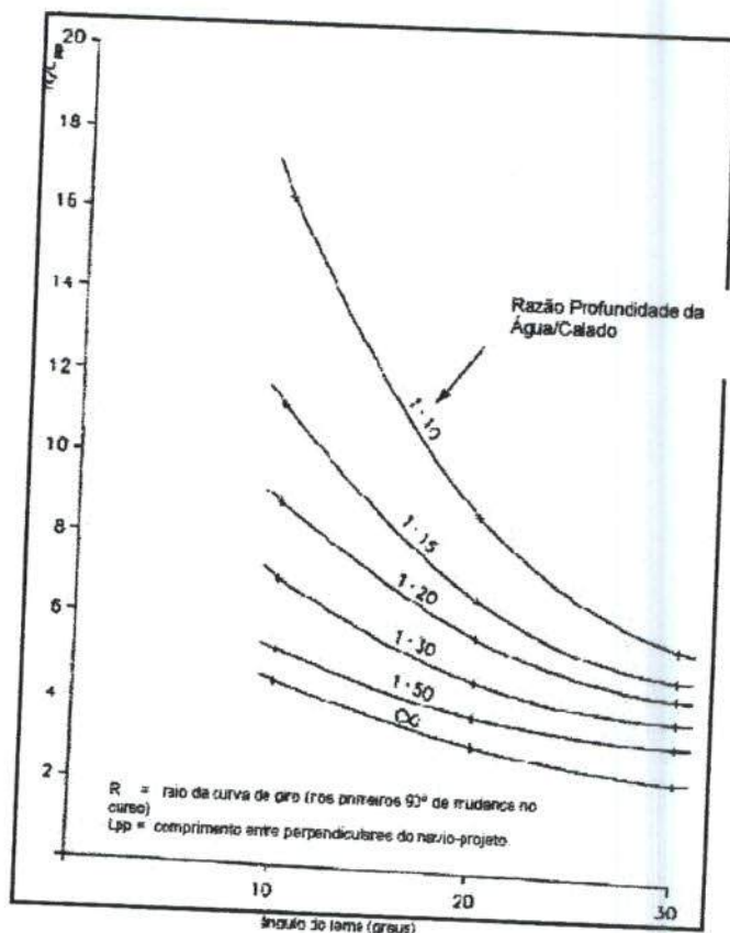
Figura 5.8 – Raio de Curva de Giro em Função do Ângulo de Leme e Profundidade da Água (Com Base em Navio Porta-Conteineres com um hélice/um leme) (PIANC)
