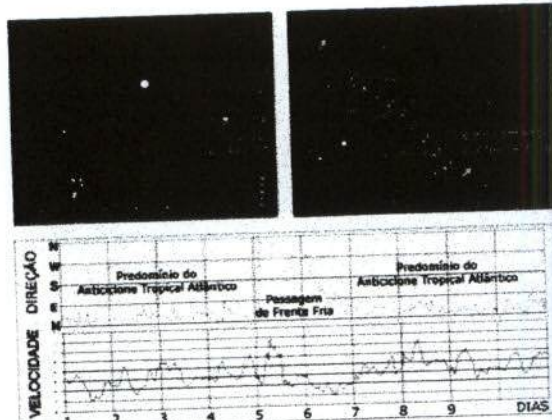
Figura 2.8: Regime dos Ventos – Ciclo Diário
