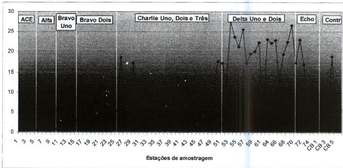
Figura 2.14: Variação das porcentagens de matéria orgânica contida nos sedimentos coletados ao longo do canal de acesso e áreas de controle na baía de Paranaguá.
