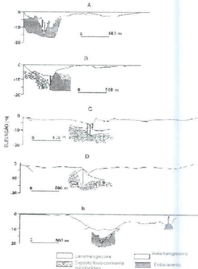
Figura 2.4 – Perfis Estratigráficos normais aos estuários Fonte: ENGEMIN, 2004
