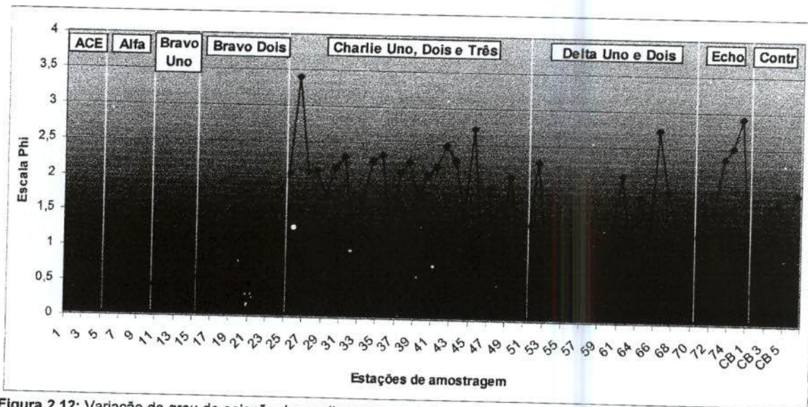
Figura 2.12: Variação do grau de seleção dos sedimentos coletados ao longo do canal de acesso e áreas de controle na baía de Paranaguá.
