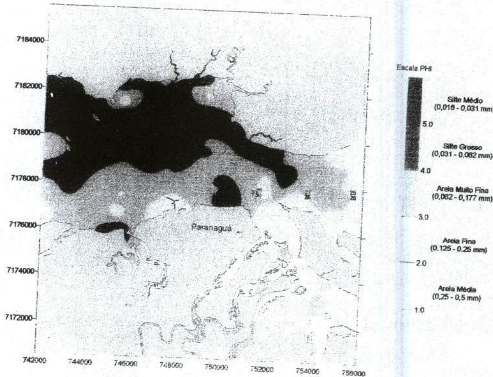
Mapa de Distribuição dos Valores de Média Granulométrica Parte da Área Bravo II, Área Charlie e parte da Área Delta
