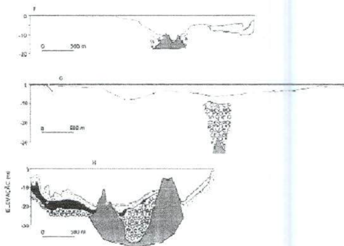
Figura 2.4 - Perfis Estratigráficos normais ao estuário Fonte: Engemin, 2004
