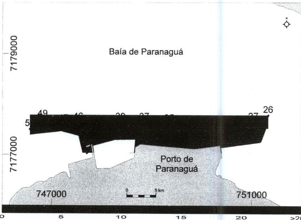
Figura 2.15: Mapa de distribuição dos valores de matéria orgânica contida nos sedimentos das áreas Charlie Uno, Dois e Três.
