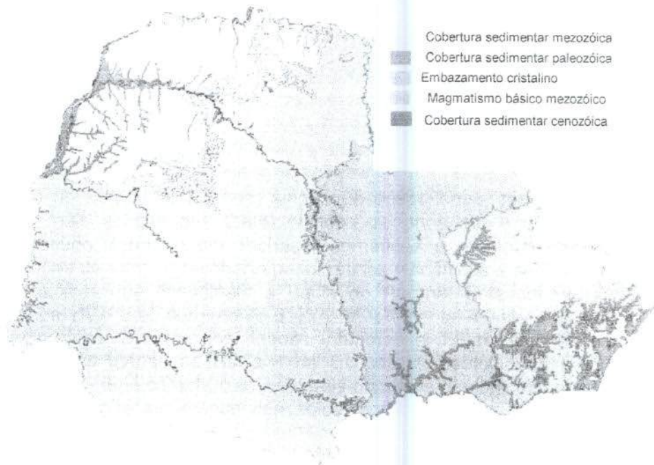
Figura 2.1 – Mapa Geológico do Paraná
