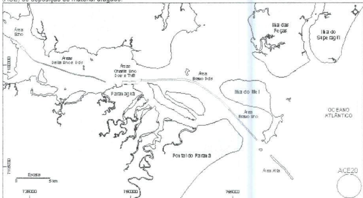
Figura 1.1: Mapa de localização das áreas de dragagem na adjacência e na baía de Paranaguá e da Área Circular Externa (ACE) de deposição de material dragado.
