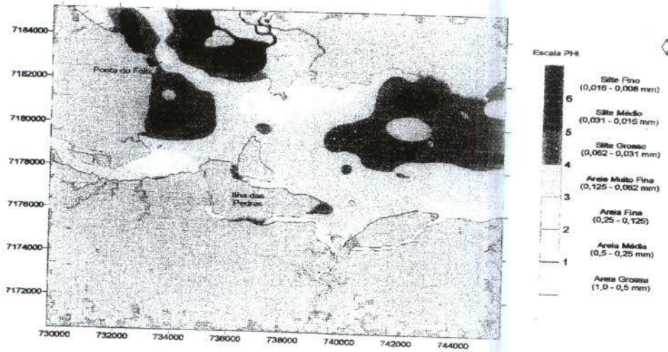
Distribuição dos Valores de Média Granulométrica Área Eono e parte da Área Delta
