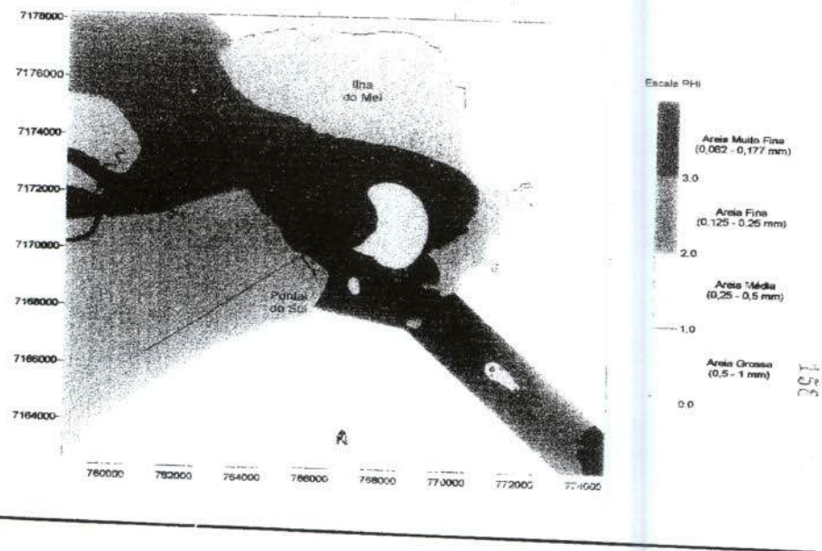
Mapa de Distribuição dos Valores de Média Granulométrica Áreas Alfa, Bravo Uno e Parte da Área Bravo Dois (SE-NW)
