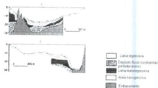
Figura 2.4 – Perfis Estratigráficos normais aos estuários Fonte: ENGEMIN, 2004
