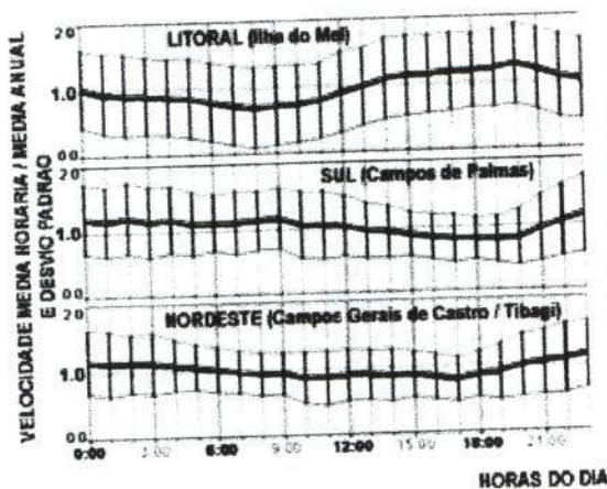
Figura 2.8: Regime dos Ventos – Ciclo Diário
