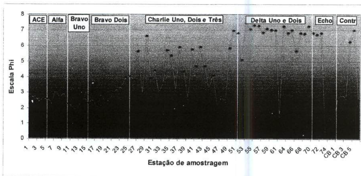
Figura 2.10: Variação do diâmetro médio de grão nos sedimentos coletados ao longo do canal de acesso e áreas de controle na baía de Paranaguá.
