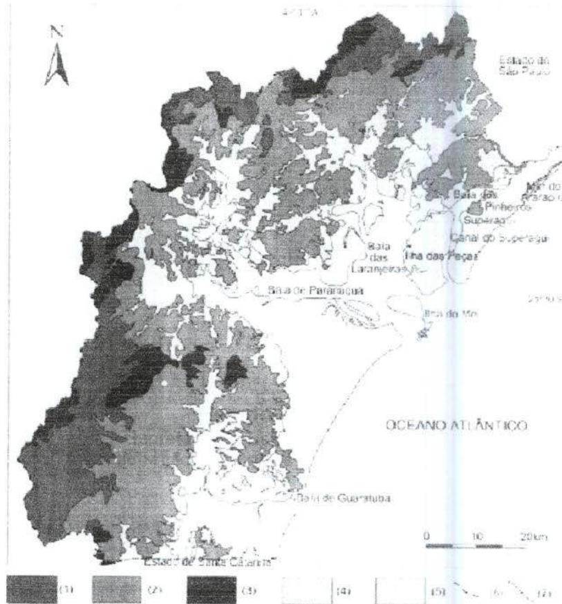
Figura 2.5 - Principais unidades geomorfológicas da região litorânea do Estado do Paraná. (1) planaltos, (2) serras originadas por dissecção de borda de planalto, (3) serras originadas por erosão diferencial, (4) talus, leques aluviais e planícies aluviais. (5) planície costeira. (6) divisor de águas e (7) limite interestadual.
