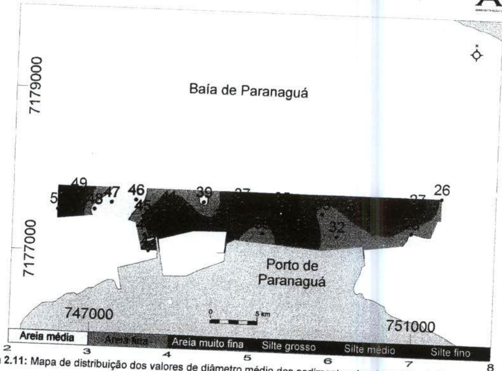
Mapa de Distribuição dos Valores de Média Granulométrica Áreas Alfa, Bravo Uno e Parte da Área Bravo Dois (SE-NW)
