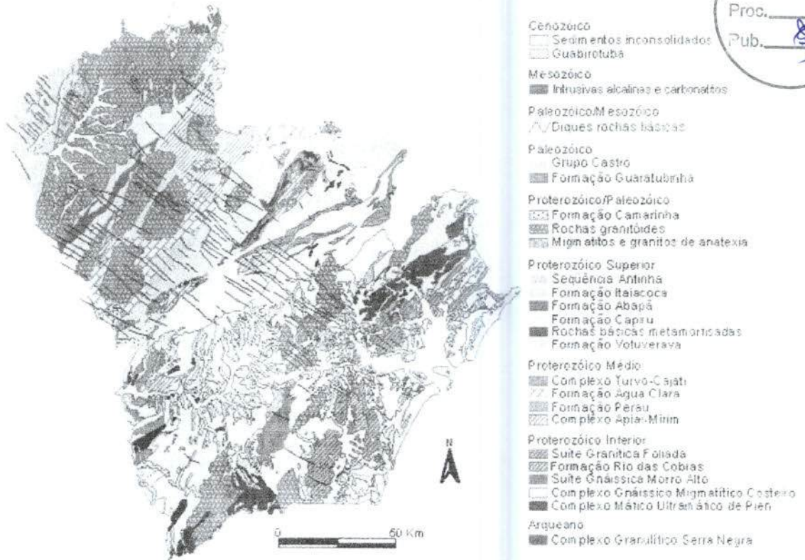
Figura 2.2 – Principais unidades geológicas do escudo Fonte: MINEROPAR
