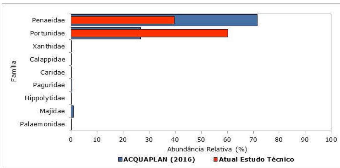
Gráfico 8.238 - Abundância de Indivíduos das famílias das espécies representantes da carcinofauna aferidas para a Área de Estudo para a determinação da Área de Influência Direta das Obras de Ampliação do Porto de Paranaguá, PR., considerando os levantamentos elaborados por ACQUAPLAN (2016) e o atual estudo.
