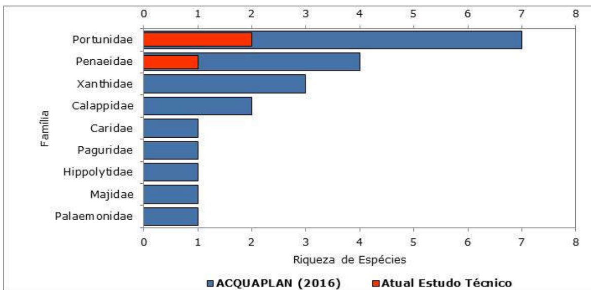
Gráfico 8.237 - Riqueza de Espécies das famílias das espécies da carcinofauna aferidas para a Área de Estudo para a determinação da Área de Influência Direta das Obras de Ampliação do Porto de Paranaguá, PR.; considerando os levantamentos elaborados por ACQUAPLAN (2016) e o atual estudo.
