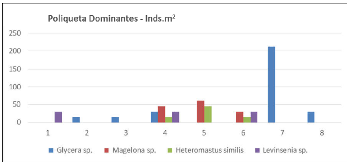
Gráfico 8.2.30 - Densidade média por m 2 das morfoespécies de poliqueta numericamente dominantes encontrados no mês de junho de 2016 para o estudo referente a ampliação do Porto de Paranaguá, situado no Complexo Estuarino de Paranaguá - CEP.
