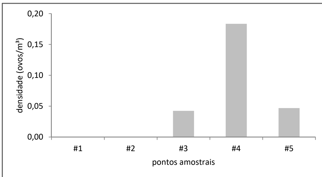
Gráfico 8.2.22 - Densidade de ovos de peixes (nº/m³) para cada ponto amostral, distribuídos no complexo estuarino Baía de Paranaguá (mais precisamente na área de estudo para determinação da área de influência das obras de Ampliação do Porto de Paranaguá), Paraná, durante a campanha realizada em junho de 2016.
