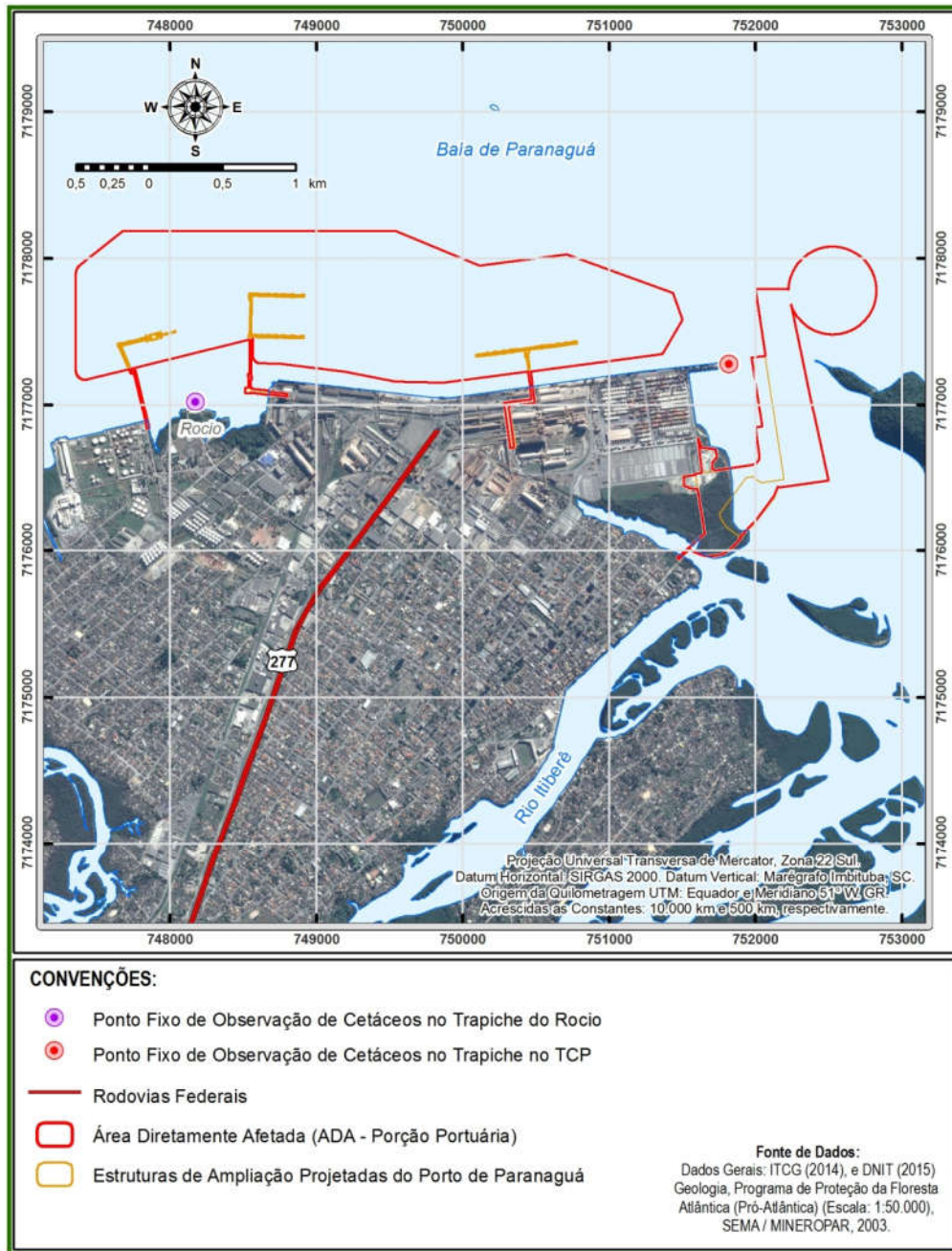
Figura 8.2.68 - Mapa com a localização dos Pontos Fixos de Observação utilizados no monitoramento da baía de Paranaguá (PR).
