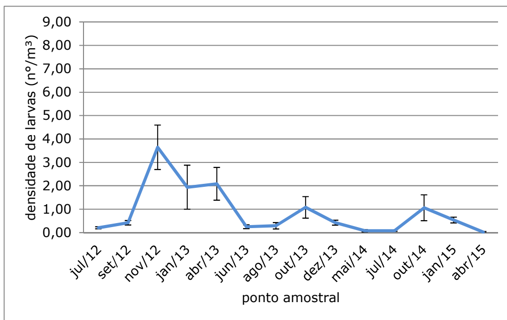
Gráfico 8.2.7 - Distribuição das densidades médias de larvas de peixes obtidas nas 14 campanhas amostrais realizadas no Complexo Estuarino de Paranaguá, PR durante julho/2012 a abril/2015.
