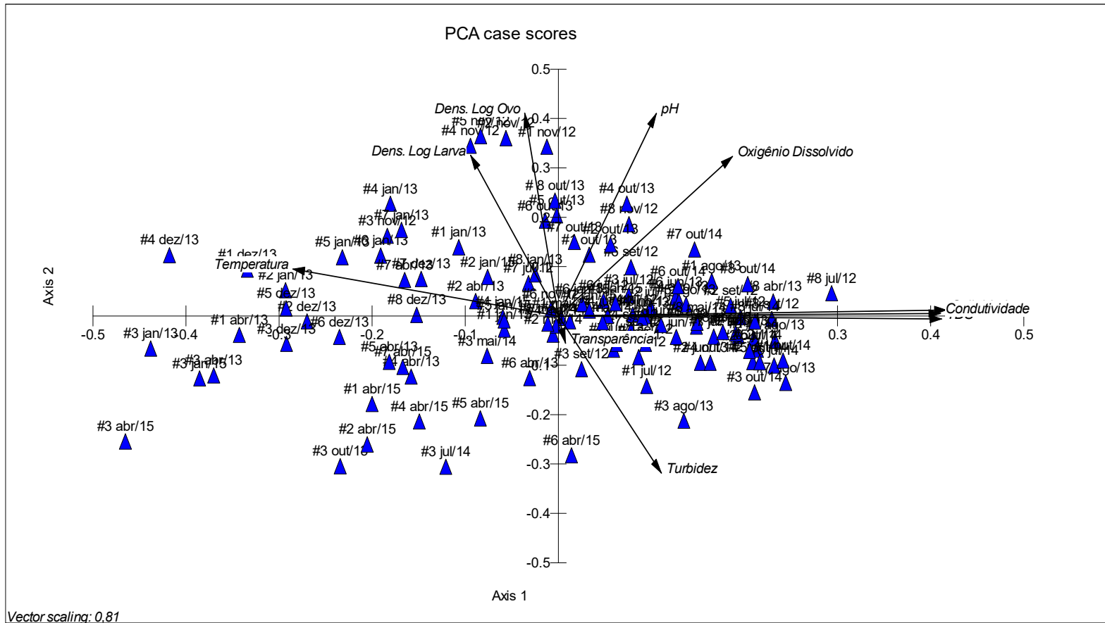
Figura 8.2.43 - Análise de componentes principais, com parâmetros abióticos e dados bióticos, para as 14 campanhas amostrais realizadas no Complexo Estuarino de Paranaguá, PR, entre julho/2012 e abril/2015.
