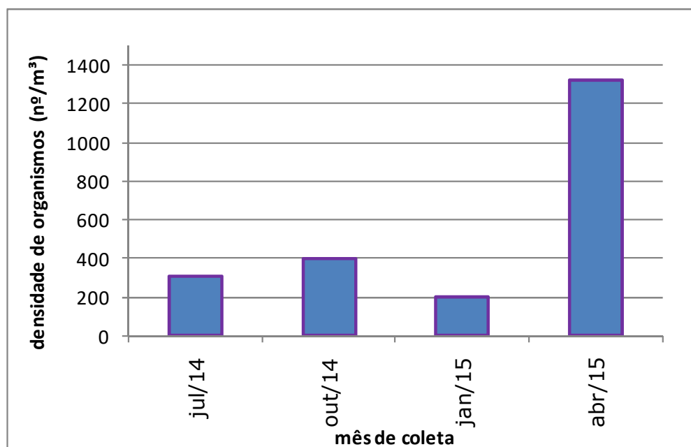
Gráfico 8.2.4 - Densidade média dos organismos zooplanctônicos para o Complexo Estuarino de Paranaguá (PR), durante a fase de operação (da ampliação) do TCP (julho/2014 a abril/2015) conforme resultados obtidos por Acquaplan (2016) no Programa de Monitoramento da Fauna Aquática.
