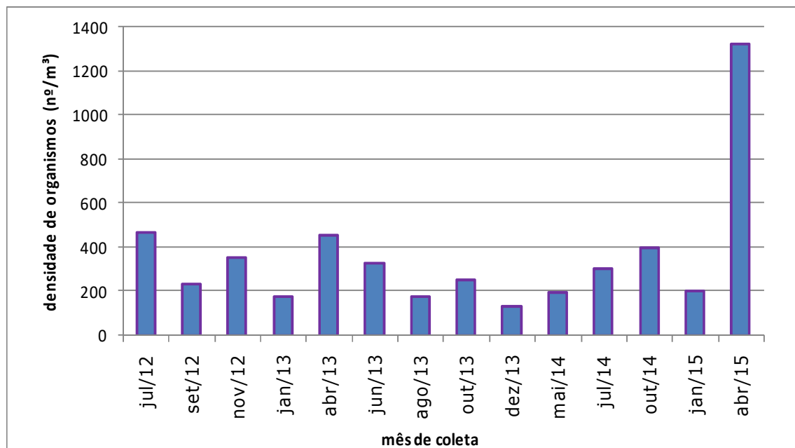
Gráfico 8.2.1 - Densidade média dos organismos zooplanctônicos para o Complexo Estuarino de Paranaguá (PR), durante o período amostral (julho/2012 e abril/2015) realizado no Programa de Monitoramento da Fauna Aquática da ampliação do TCP.
