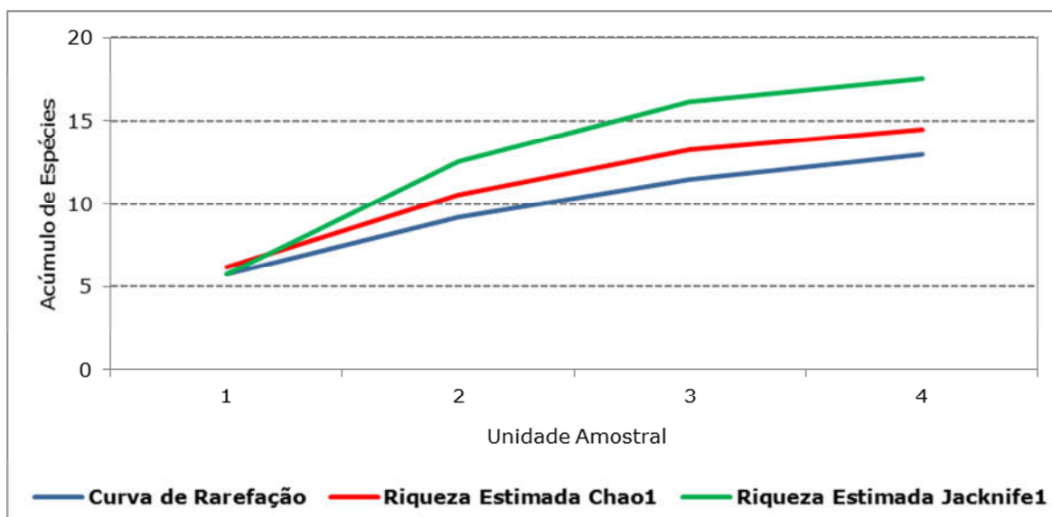
Gráfico 8.2.42 - Curva de Acumulação de Espécies Observada e Curvas de Diversidade Estimada com o Índice de Chao1 e Índice de Jacknife 1 aferidas para as espécies diagnosticadas na Área de Estudo para a determinação da Área de Influência Direta das Obras de Ampliação do Porto de Paranaguá, PR.
