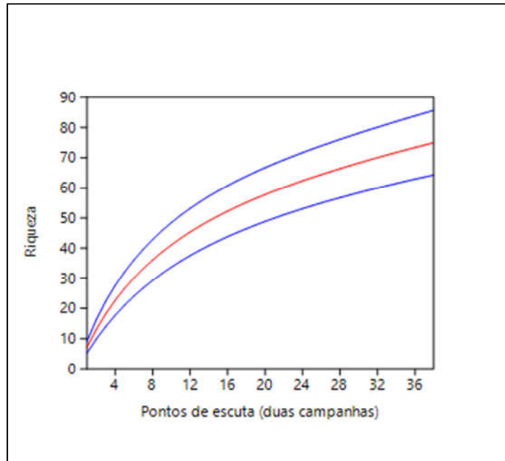
Figura 8.2.26 - Curva de rarefação gerada pelo software PAST.
