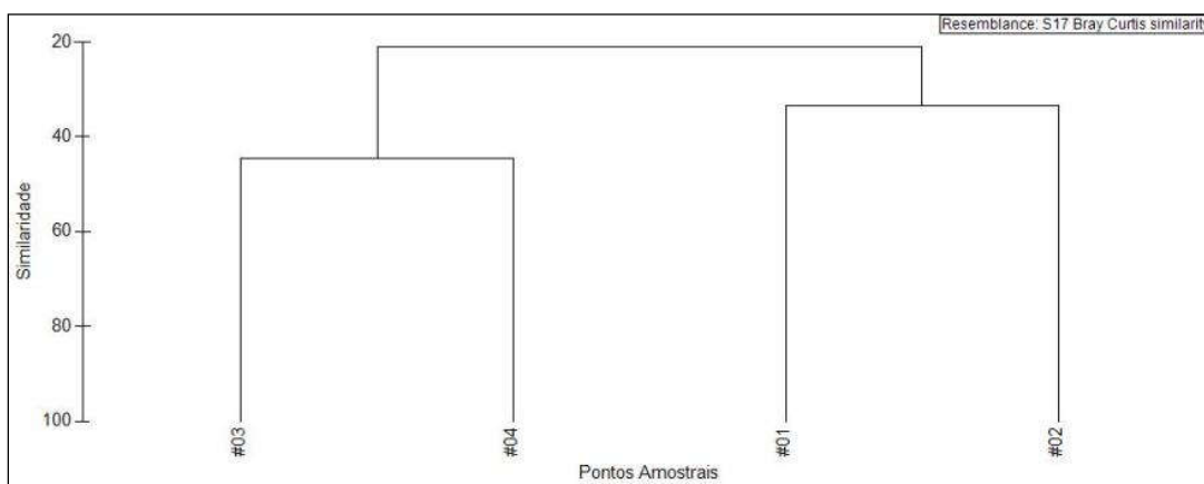
Figura 8.2.54 - Dendrograma da Análise de Agrupamento aferida para as estações amostrais localizadas na Área de Estudo para a determinação da Área de Influência Direta das Obras de Ampliação do Porto de Paranaguá, PR.
