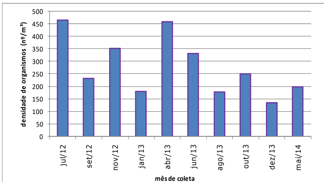
Gráfico 8.2.3 - Densidade média dos organismos zooplânctônicos para o Complexo Estuarino de Paranaguá (PR), durante a fase de implantação da ampliação do TCP (julho/2012 a maio/2014).
