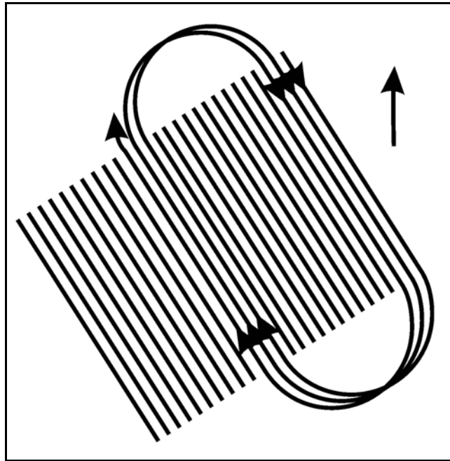
Figura II.2.1.2-3 - Representação gráfica das linhas (transectos), direção e área de manobra da embarcação sísmica.
