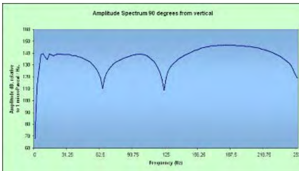
Figura II.2.2.2-4 – Espectro de frequência da fonte do arranjo de canhões de ar de 3.147 pol 3 ; Amplitude x Frequência (horizontal).
