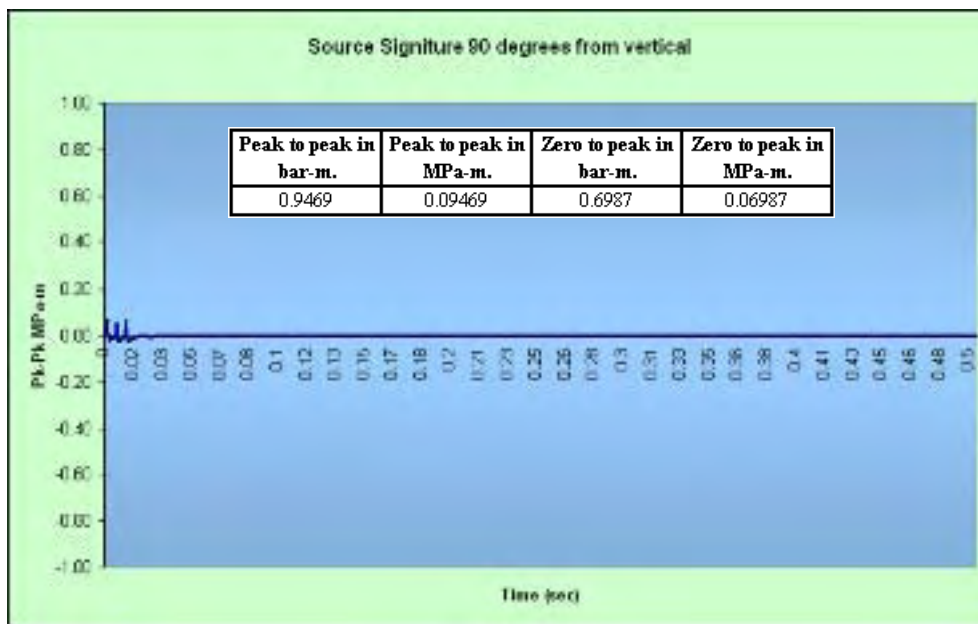
Figura II.2.2.2-3 – Assinatura da fonte do arranjo de canhões de ar de 3.147 pol 3 ; Amplitude x Tempo (horizontal).
