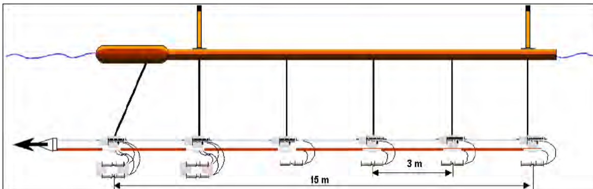
Figura II.2.2.1-1 – Vista lateral do subarranjo de 8 canhões de ar, com 1.049 pol 3 .
