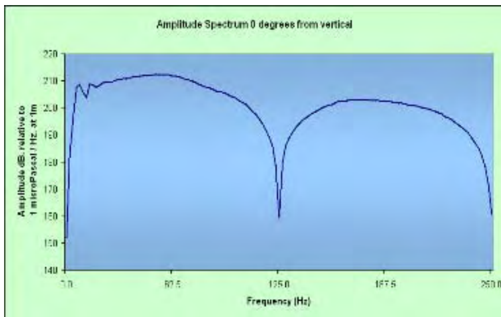
Figura II.2.2.2-2 – Espectro de frequência da fonte do arranjo de canhões de ar de 3.147 pol 3 ; Amplitude x Frequência (vertical).
