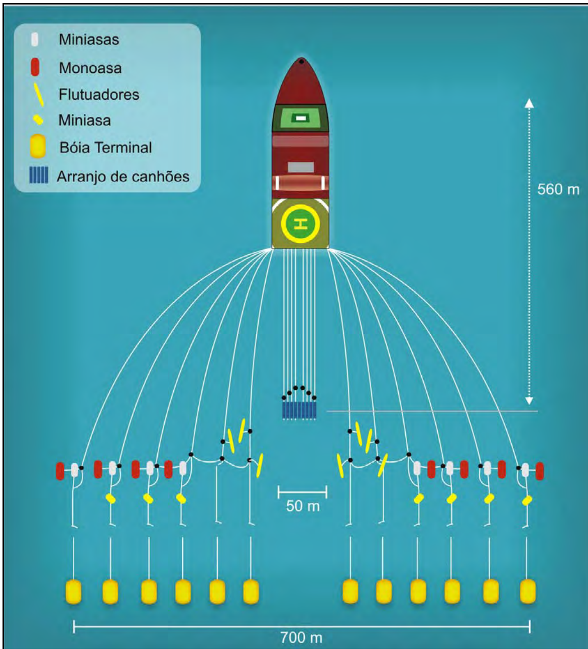
Figura II.2.3-1 – Configuração de um sistema de registro de dados sísmicos com 12 linhas de cabos.
