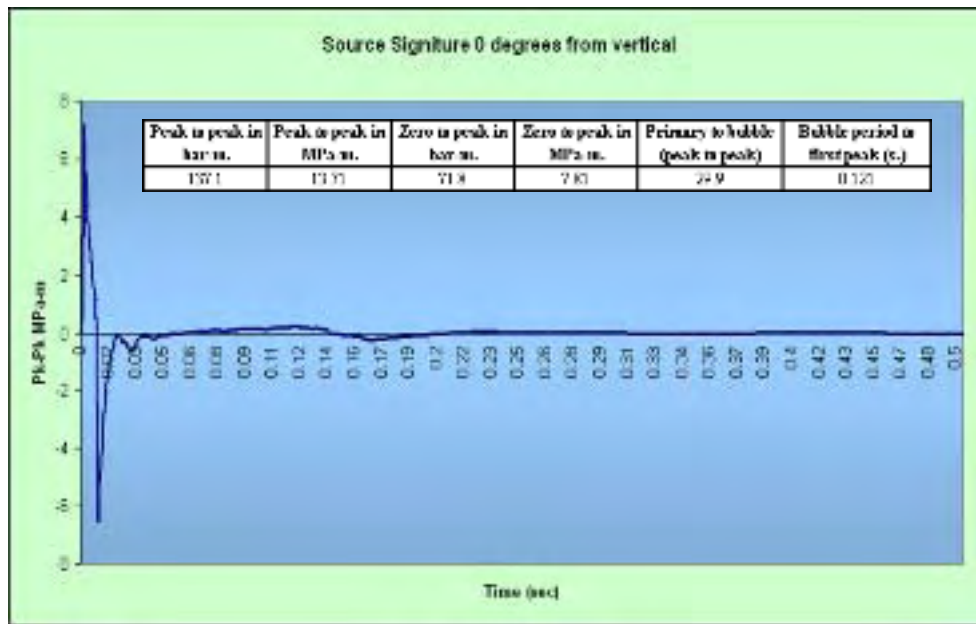
Figura II.2.2.2-1 – Assinatura da fonte do arranjo de canhões de ar de 3.147 pol 3 ; Amplitude x Tempo (vertical).
