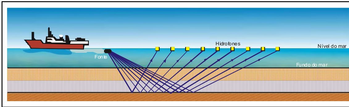
Figura II.2.1.2-2 - Representação gráfica do método de aquisição sísmica por reflexão.
