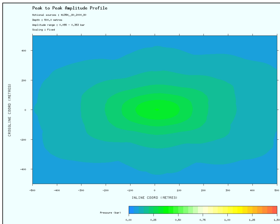
Figura 2.2i – Plano de fundo horizontal (“depth plane”) na amplitude pico-a-pico do arranjo de canhão 4135H_80_2000_80 a uma profundidade de 500 metros (Escala de cores de 0 bar-metros a 1,5 bar-metros equivale a 160dB re 1 \mu Pa a 1m (0.001 bar-meters) a 224dB re 1 \mu Pa a 1m) (CAMPBELL, 2010)
