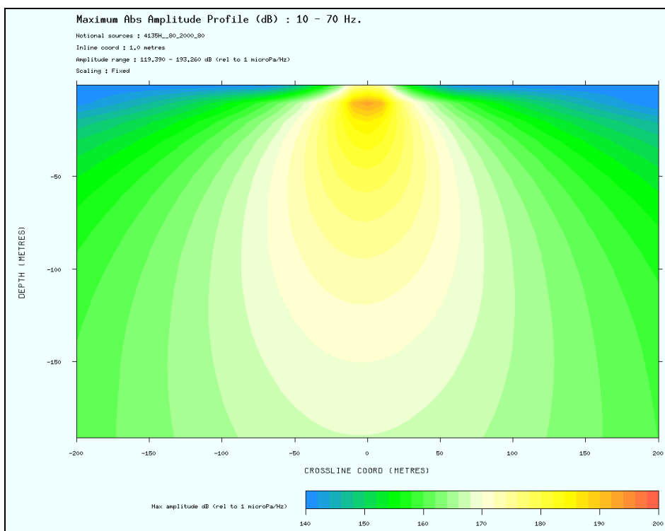
Figura 2.2e – Perfil vertical transversal (“crossline”) na amplitude absoluta máxima do arranjo de canhão 4135H_80_2000_80 a uma profundidade de 200 metros (Escala de cores de 140dB re 1 \mu Pa a 1m (0.001 bar-meters) a 200dB re 1 \mu Pa a 1m) (CAMPBELL, 2010)
