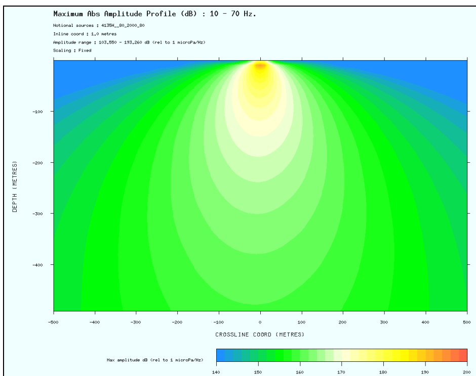
Figura 2.2k – Perfil vertical transversal (“crossline”) na amplitude absoluta máxima do arranjo de canhão 4135H_80_2000_80 a uma profundidade de 500 metros (Escala de cores de 140dB re 1 \mu Pa a 1m (0.001 bar-meters) a 200dB re 1 \mu Pa a 1m) (CAMPBELL, 2010)
