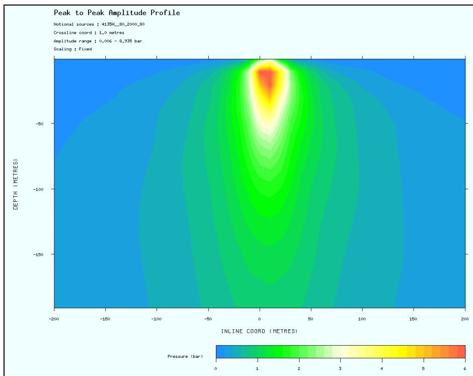
Figura 2.2a – Perfil longitudinal (“inline”) na amplitude pico-a-pico do arranjo de canhão 4135H_80_2000_80 a uma profundidade de 200 metros (Escala de cores de 0 bar-metros a 6 bar-metros equivale a 160dB re 1 \mu Pa a 1m (0.001 bar-meters) a 235dB re 1 \mu Pa a 1m) (CAMPBELL, 2010)
