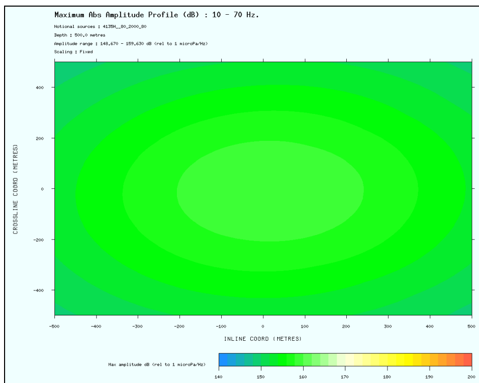
Figura 2.21 – Plano de fundo horizontal (“depth plane”) na amplitude absoluta máxima do arranjo de canhão 4135H_80_2000_80 a uma profundidade de 500 metros (Escala de cores de 140dB re 1 \mu Pa a 1m (0.001 bar-meters) a 200dB re 1 \mu Pa a 1m) (CAMPBELL, 2010)
