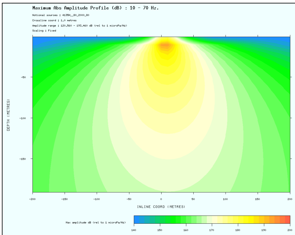
Figura 2.2d – Perfil longitudinal (“inline”) na amplitude absoluta máxima do arranjo de canhão 4135H_80_2000_80 a uma profundidade de 200 metros (Escala de cores de 140dB re 1 \mu Pa a 1m (0.001 bar-meters) a 200dB re 1 \mu Pa a 1m) (CAMPBELL, 2010)
