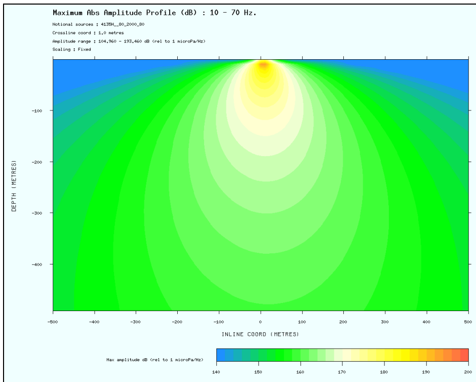
Figura 2.2j – Perfil longitudinal (“inline”) na amplitude absoluta máxima do arranjo de canhão 4135H_80_2000_80 a uma profundidade de 500m (Escala de cores de 140dB re 1 \mu Pa a 1m (0.001 bar-meters) a 200dB re 1 \mu Pa a 1m) (CAMPBELL, 2010)
