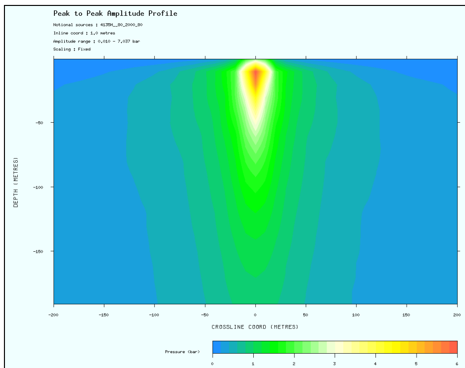
Figura 2.2b – Perfil vertical transversal (“crossline”) na amplitude pico-a-pico do arranjo de canhão 4135H_80_2000_80 a uma profundidade de 200 metros (Escala de cores de 0 bar-metros a 6 bar-metros equivale a 160dB re 1 \mu Pa a 1m (0.001 bar-meters) a 235dB re 1 \mu Pa a 1m) (CAMPBELL, 2010)
