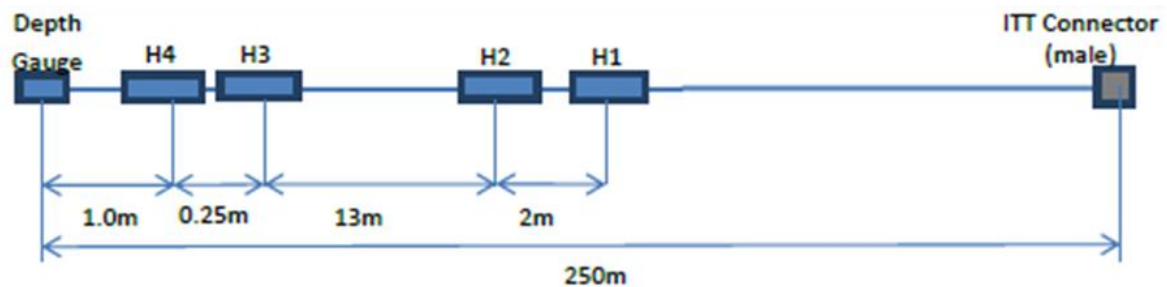
Figura 9.11.6 - Arranjo de hidrofones
