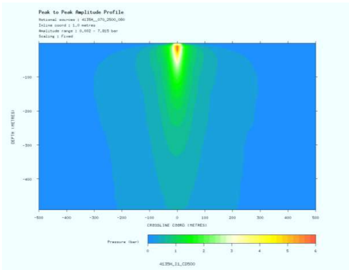
Figura 2.2-2h – Perfil vertical transversal (“crossline”) na amplitude pico-a-pico do arranjo de canhão 4135H_070_2500_080 a uma profundidade de 500 metros (Escala de cores de 0 bar-metros a 1,5 bar-metros equivale a 160dB re 1 \mu Pa a 1m (0.001 bar-meters) a 224dB re 1 \mu Pa a 1m).
