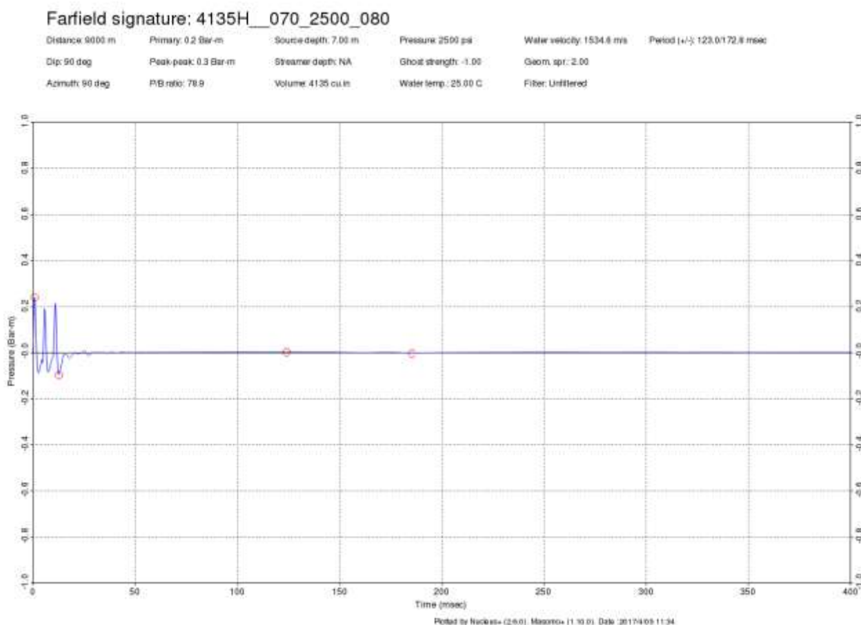
Figura 2.2-1d – Assinatura da fonte (far-field) na horizontal (90   ngulo e 90  azimute) do arranjo 4135H_070_2500_080.
