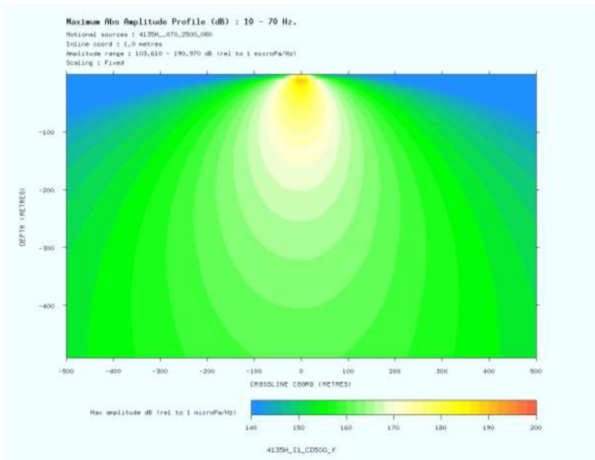
Figura 2.2-2k – Perfil vertical transversal (“crossline”) na amplitude absoluta máxima do arranjo de canhão 4135H_070_2500_080 a uma profundidade de 500 metros (Escala de cores de 140dB re 1 \mu Pa a 1m (0.001 bar-meters) a 200dB re 1 \mu Pa a 1m).
