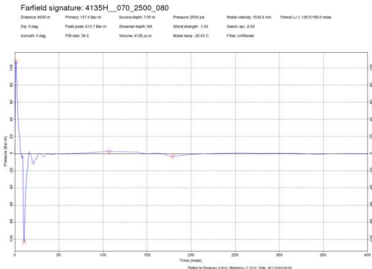
Figura 2.2-1b – Assinatura da fonte (far-field) na vertical (0° ângulo e 0° azimute) do arranjo 4135H_070_2500_080.
