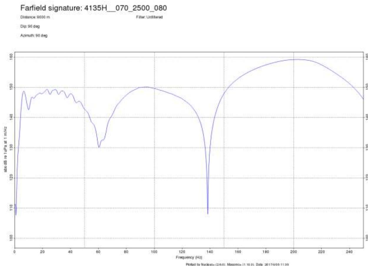
Figura 2.2-1e – Espectro de amplitude horizontal (90° ângulo e 90° azimute) do arranjo 4135H_070_2500_080 nas frequências variáveis entre 0 e 200Hz (Amplitudes em dB re: 1 \mu\text{Pa}/\text{Hz} a 1m da fonte).
