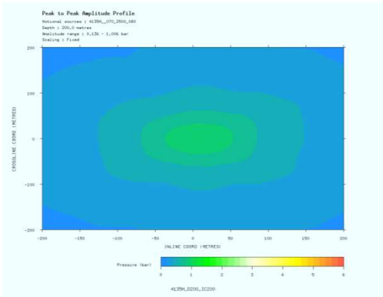
Figura 2.2-2c – Plano de fundo horizontal (“depth plane”) na amplitude pico-a-pico do arranjo de canh o 4135H_070_2500_080 a uma profundidade de 200 metros (Escala de cores de 0 bar-metros a 6 bar-metros equivale a 160dB re 1 Pa a 1m (0.001 bar-meters) a 235dB re 1 Pa a 1m).
