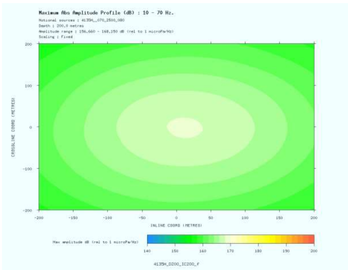
Figura 2.2-2f – Plano de fundo horizontal (“depth plane”) na amplitude absoluta máxima do arranjo de canhão 4135H_070_2500_080 a uma profundidade de 200 metros (Escala de cores de 140dB re 1 \mu Pa a 1m (0.001 bar-meters) a 200dB re 1 \mu Pa a 1m).
