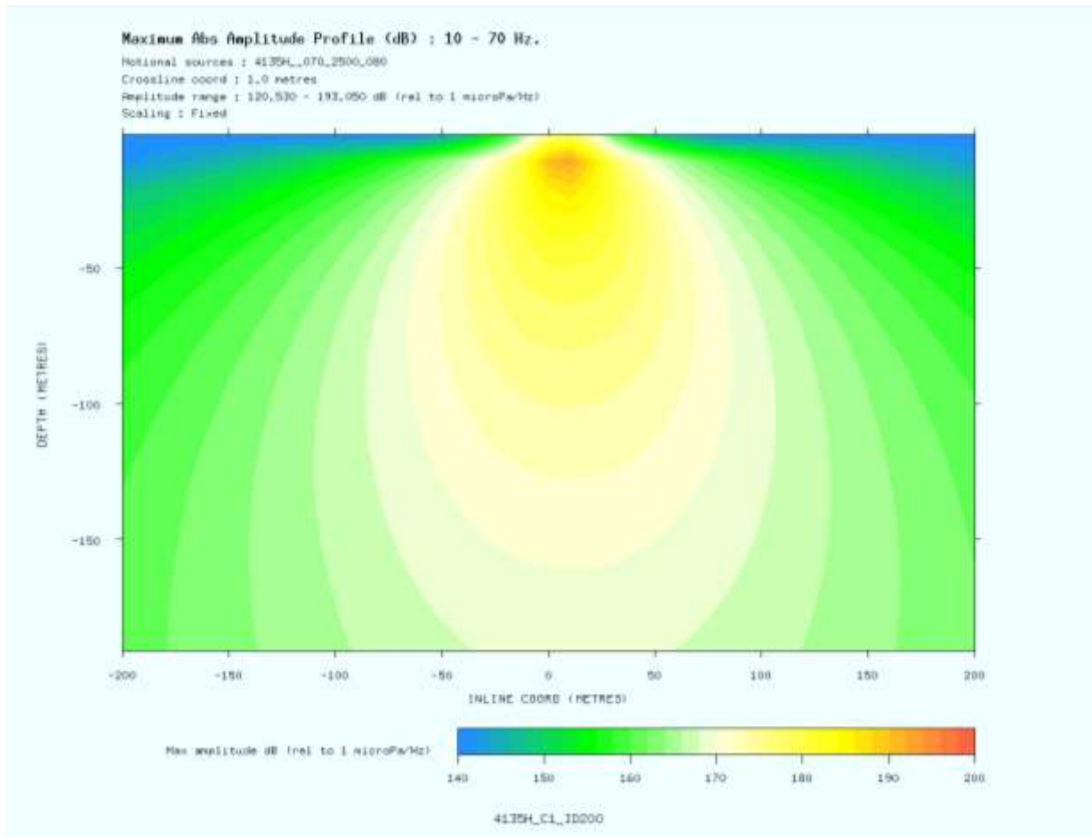
Figura 2.2-2d – Perfil longitudinal (“inline”) na amplitude absoluta máxima do arranjo de canhão 4135H_070_2500_080 a uma profundidade de 200 metros (Escala de cores de 140dB re 1 \mu Pa a 1m (0.001 bar-meters) a 200dB re 1 \mu Pa a 1m).
