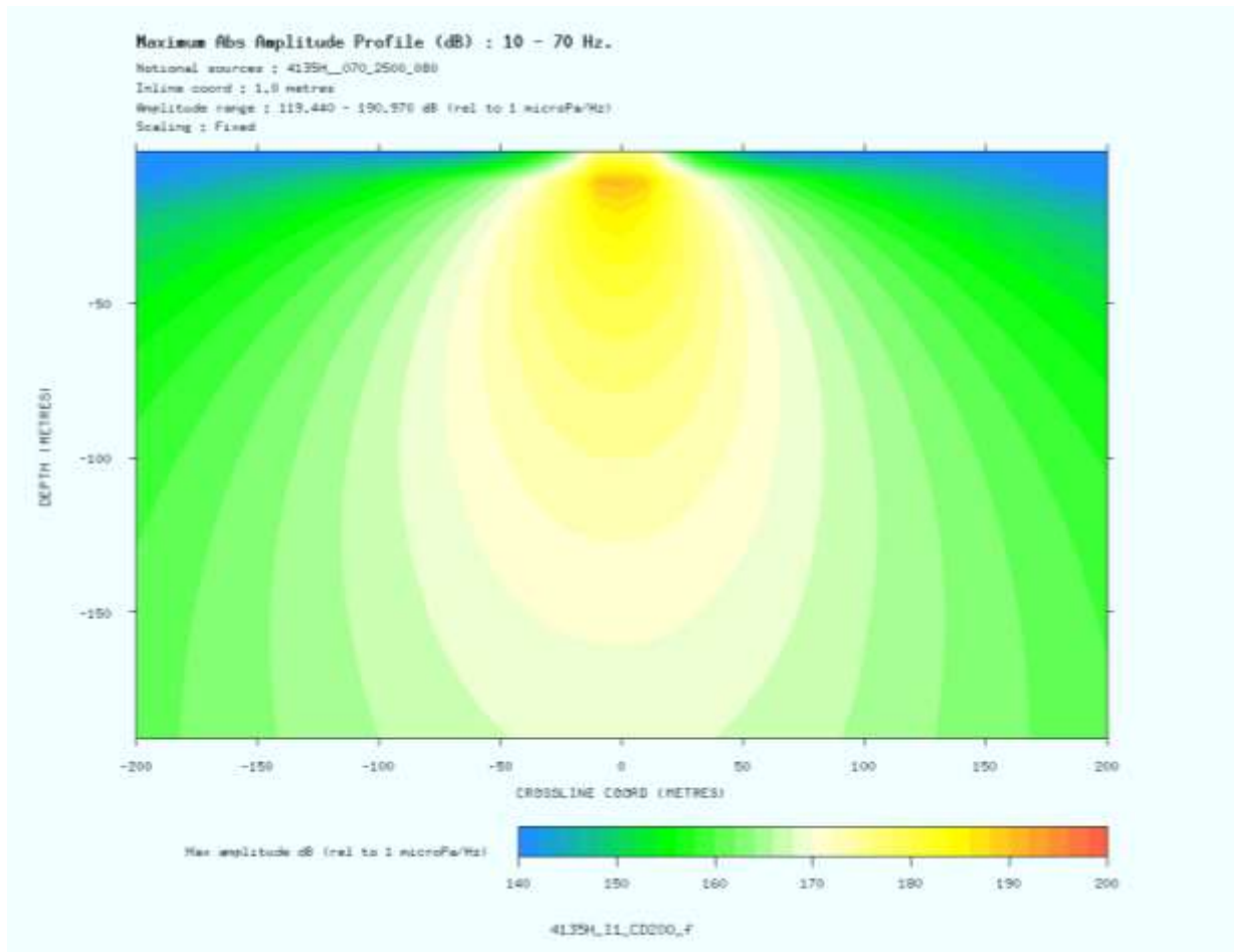
Figura 2.2-2e – Perfil vertical transversal (“crossline”) na amplitude absoluta máxima do arranjo de canhão 4135H_070_2500_080 a uma profundidade de 200 metros (Escala de cores de 140dB re 1 \mu Pa a 1m (0.001 bar-meters) a 200dB re 1 \mu Pa a 1m).
