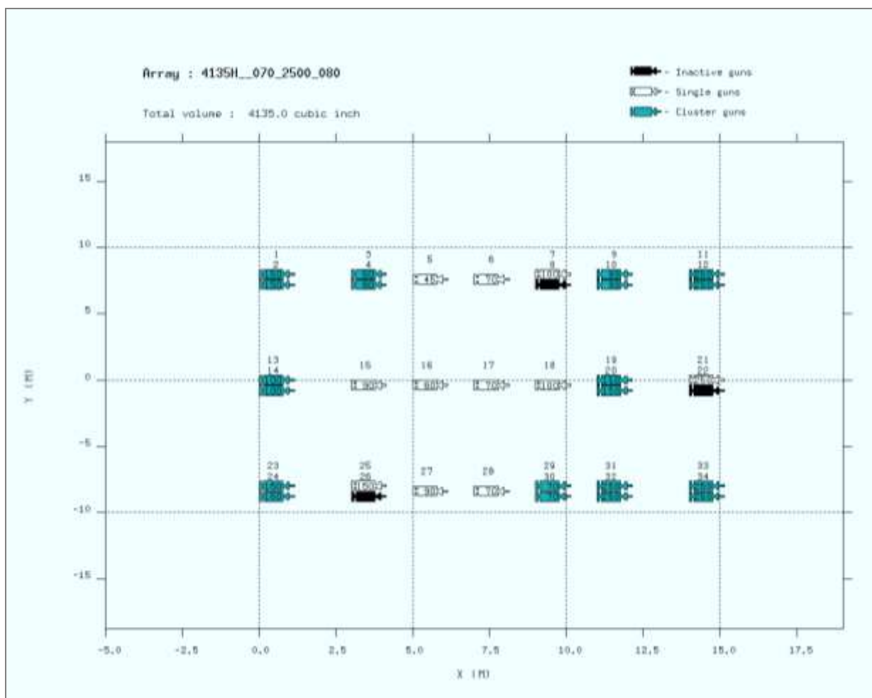
Figura 2.2-1a – Configuração geométrica do Arranjo de Canhões 4135H_070_2500_080.
