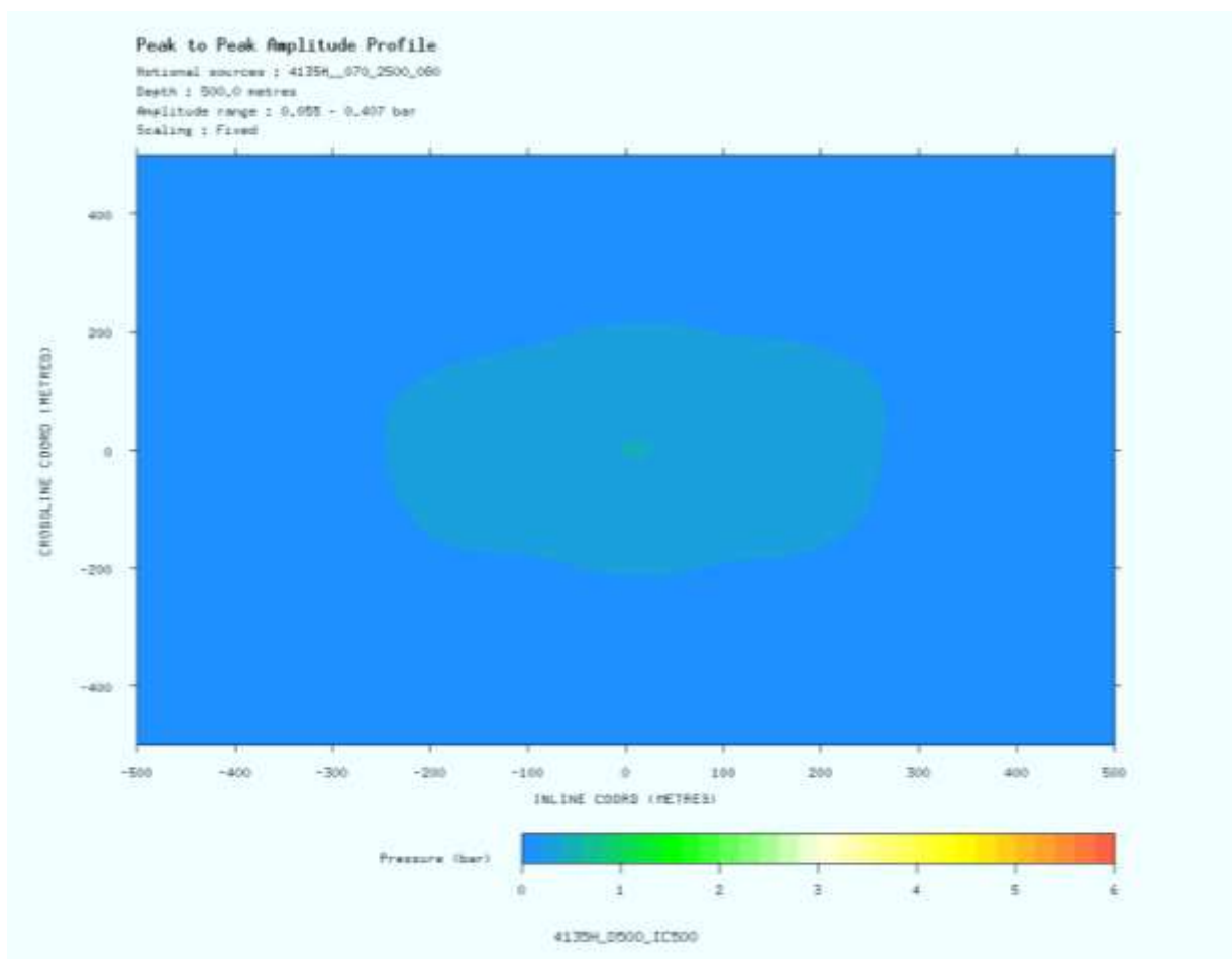
Figura 2.2-2i – Plano de fundo horizontal (“depth plane”) na amplitude pico-a-pico do arranjo de canhão 4135H_070_2500_080 a uma profundidade de 500 metros (Escala de cores de 0 bar-metros a 1,5 bar-metros equivale a 160dB re 1 \mu Pa a 1m (0.001 bar-meters) a 224dB re 1 \mu Pa a 1m).
