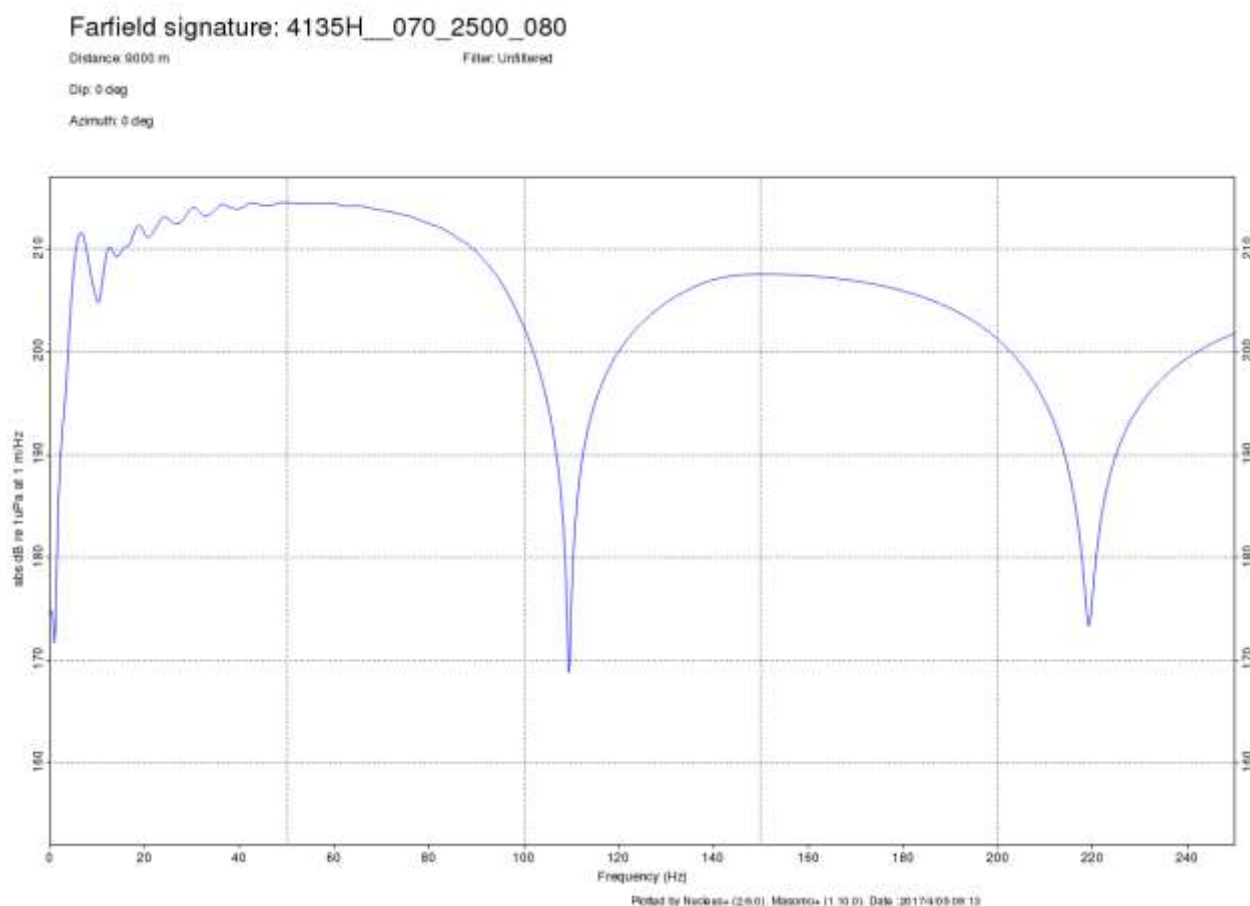
Figura 2.2-1c – Espectro de amplitude vertical (0° ângulo e 0° azimute) do arranjo 4135H_070_2500_080 nas frequências variáveis entre 0 e 200Hz (Amplitudes em dB re: 1 \mu Pa/Hz a 1m da fonte).
