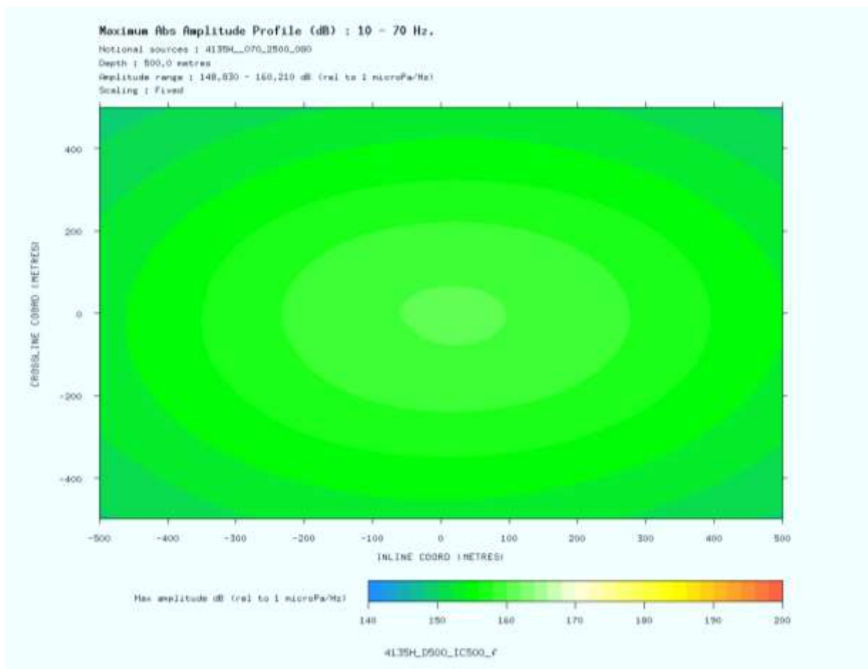
Figura 2.2-2I – Plano de fundo horizontal (“depth plane”) na amplitude absoluta máxima do arranjo de canhão 4135H_070_2500_080 a uma profundidade de 500 metros (Escala de cores de 140dB re 1 \mu Pa a 1m (0.001 bar-meters) a 200dB re 1 \mu Pa a 1m).
