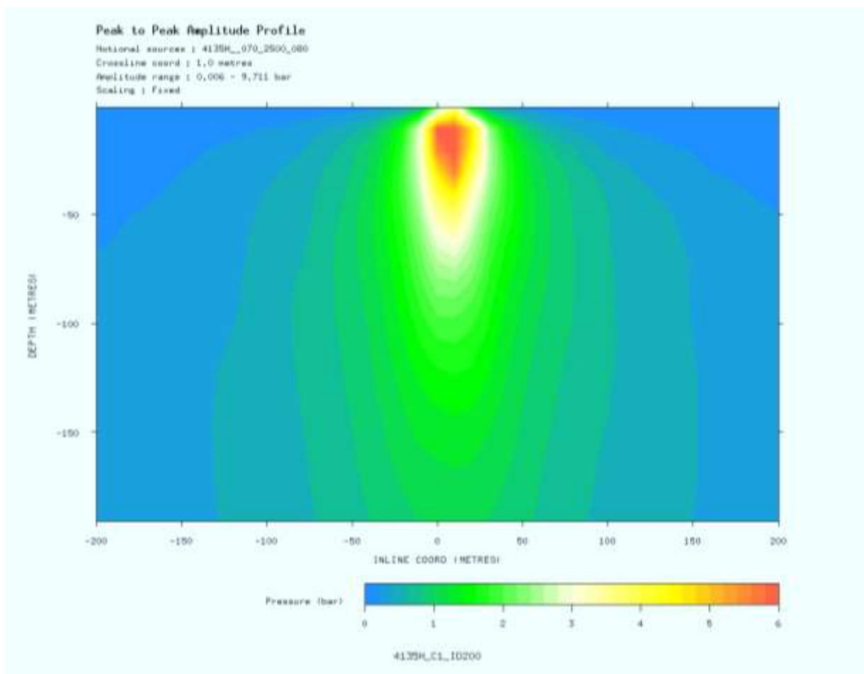
Figura 2.2-2a – Perfil longitudinal (“inline”) na amplitude pico-a-pico do arranjo de canhão 4135H_070_2500_080 a uma profundidade de 200 metros (Escala de cores de 0 bar-metros a 6 bar-metros equivale a 160dB re 1 \mu Pa a 1m (0.001 bar-meters) a 235dB re 1 \mu Pa a 1m).
