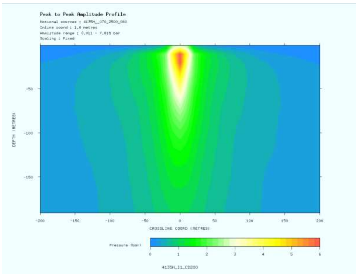
Figura 2.2-2b – Perfil vertical transversal (“crossline”) na amplitude pico-a-pico do arranjo de canhão 4135H_070_2500_080 a uma profundidade de 200 metros (Escala de cores de 0 bar-metros a 6 bar-metros equivale a 160dB re 1 \mu Pa a 1m (0.001 bar-meters) a 235dB re 1 \mu Pa a 1m).
