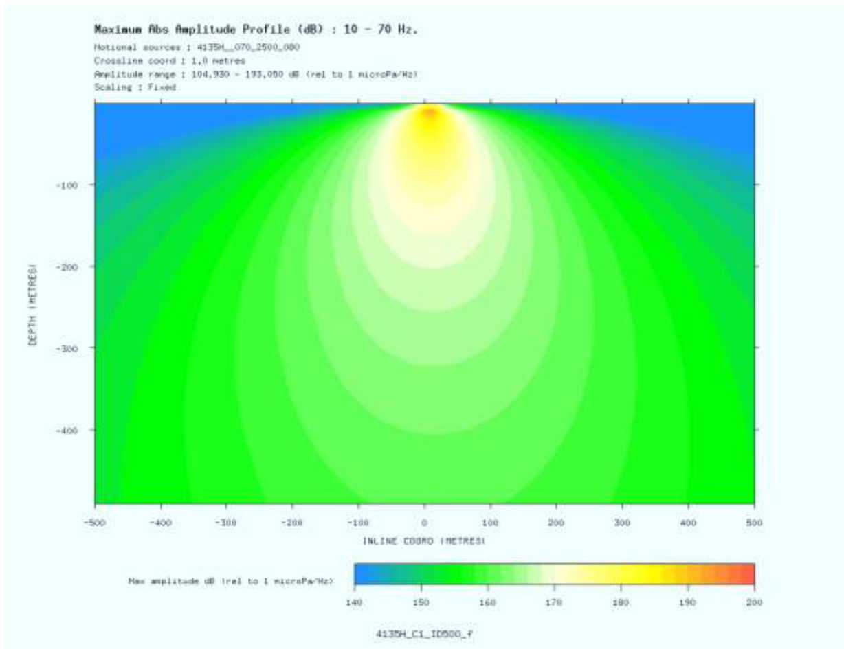
Figura 2.2-2j – Perfil longitudinal (“inline”) na amplitude absoluta m xima do arranjo de canh o 4135H_070_2500_080 a uma profundidade de 500m (Escala de cores de 140dB re 1 Pa a 1m (0.001 bar-meters) a 200dB re 1 Pa a 1m).
