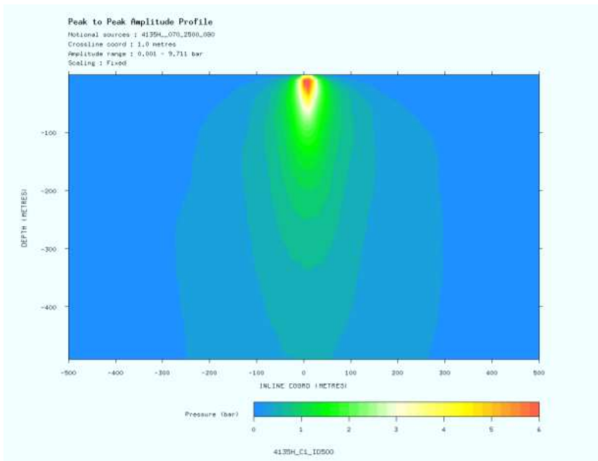
Figura 2.2-2g – Perfil longitudinal (“inline”) na amplitude pico-a-pico do arranjo de canhão 4135H_070_2500_080 a uma profundidade de 500 metros (Escala de cores de 0 bar-metros a 1,5 bar-metros equivale a 160dB re 1 \mu Pa a 1m (0.001 bar-meters) a 224dB re 1 \mu Pa a 1m).
