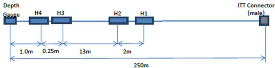
Figura 9.4.6 - Arranjo de hidrofones
