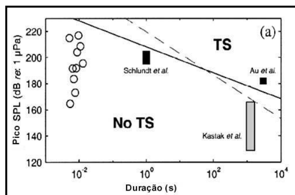
Fig.7.2.1c – Dados de TTS existentes na literatura para mamíferos marinhos. Valores SPL pico versus duração do tempo de fadiga. o = FINNERAN et al. (2000). Linha sólida = indução de perda de 3 dB. Linha tracejada = indução de perda de 5 dB.
