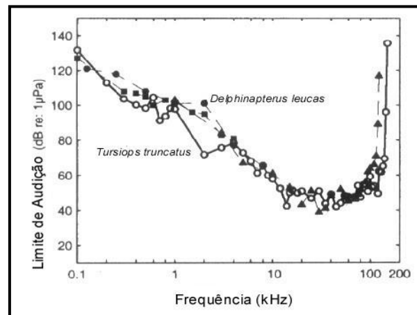
Fig.7.2.1b - Audiogramas comportamentais de Delphinapterus leucas e Tursiops truncatus (SCHLUNDT et al. , 2000).
