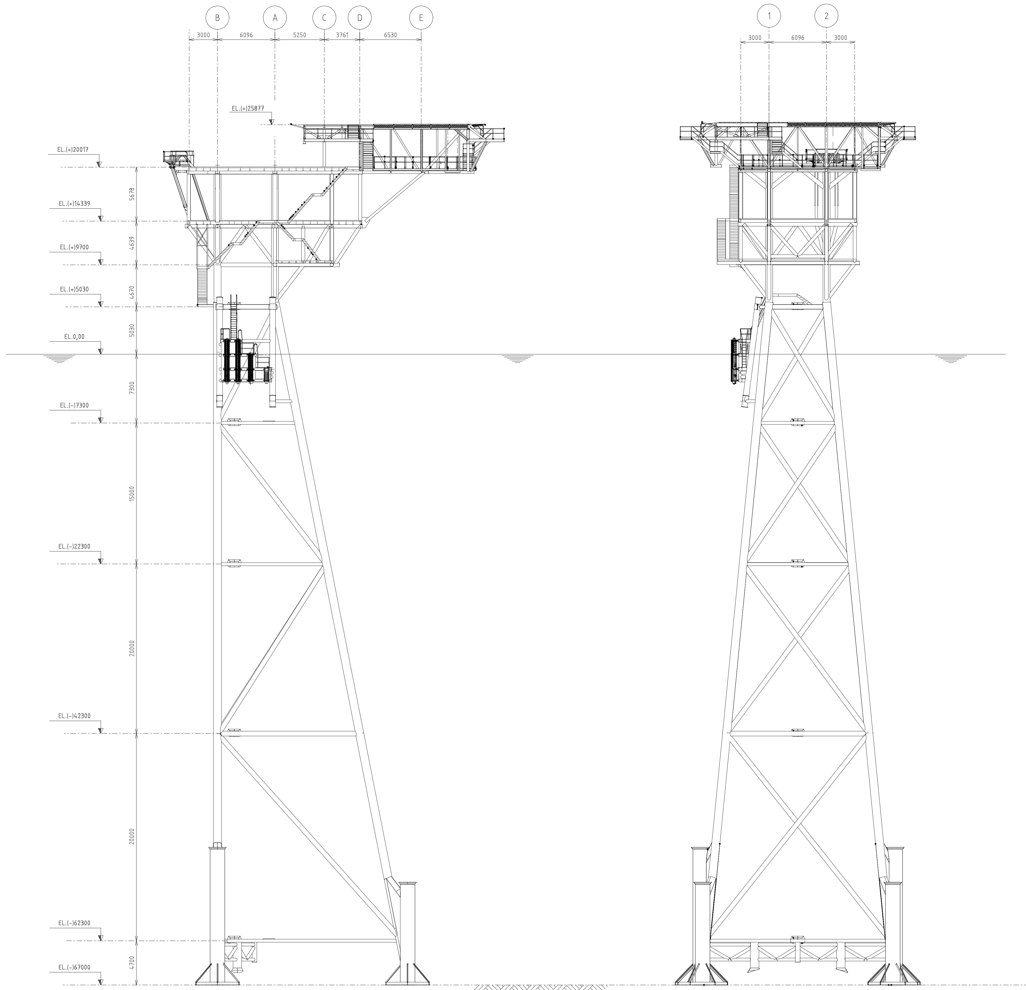
ELEVÇÃO EIXOS 1 - 2 ESC:1:75
