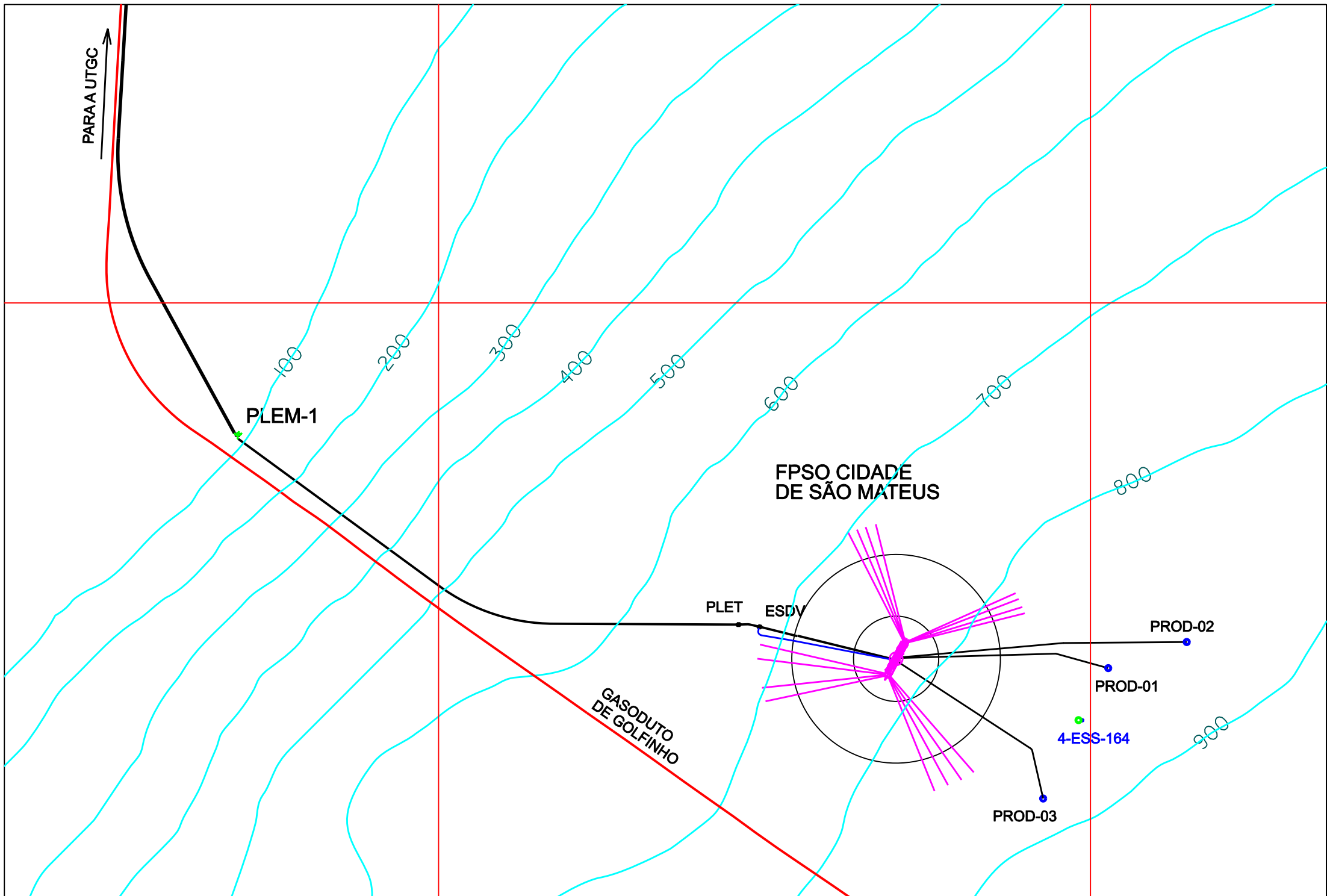
Figura II.2.1-3 - Arranjo submarino do Campo de Camarupim.
