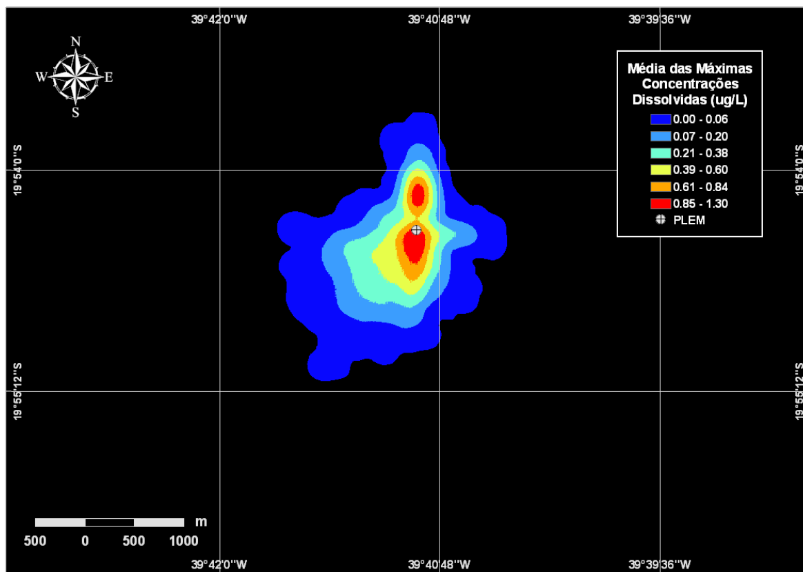
Figura VI.4-2 - Média das máximas concentrações esperadas ( \mu\text{g/L} ) para a pluma de FLUORENE R2, simulada no período de inverno (junho a agosto), após 1 hora, para o PLEM do Campo de Camarupim.
