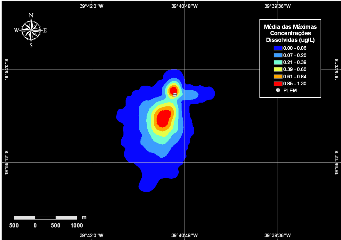
Figura VI.4-1 - Média das máximas concentrações esperadas ( \mu\text{g/L} ) para a pluma de FLUORENE R2, simulada no período de verão (janeiro a março), após 1 hora, para o PLEM do Campo de Camarupim.
