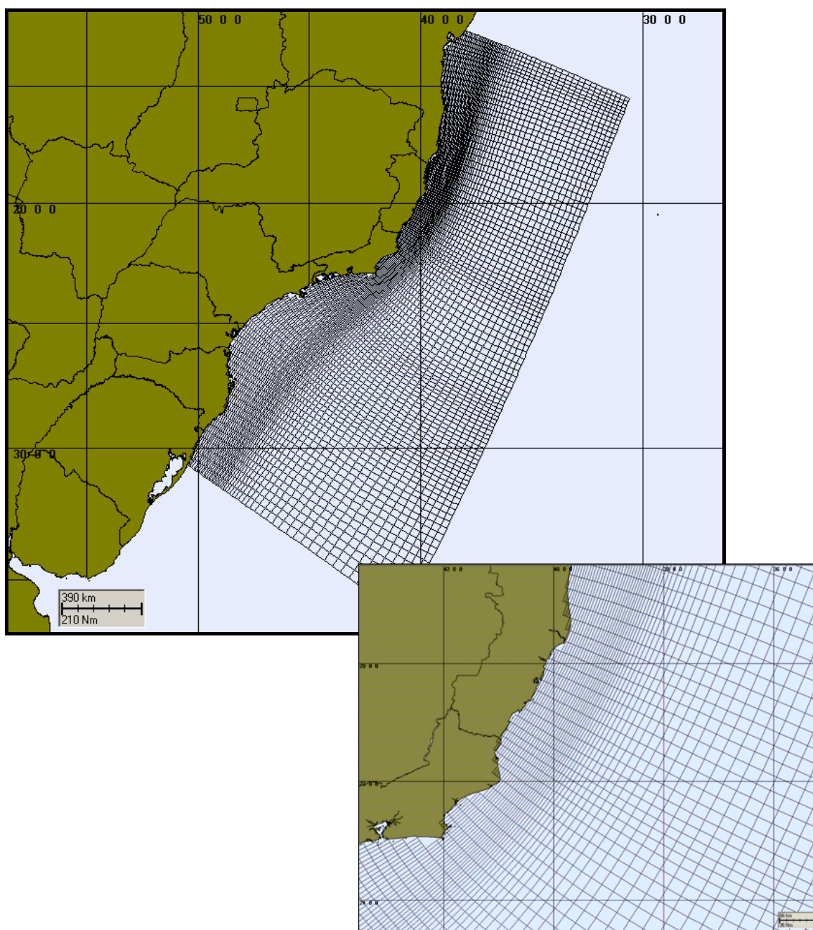
Figura II.3.1-1 - Grade computacional utilizada nas simulações da circulação hidrodinâmica da Bacia do Espírito Santo.
