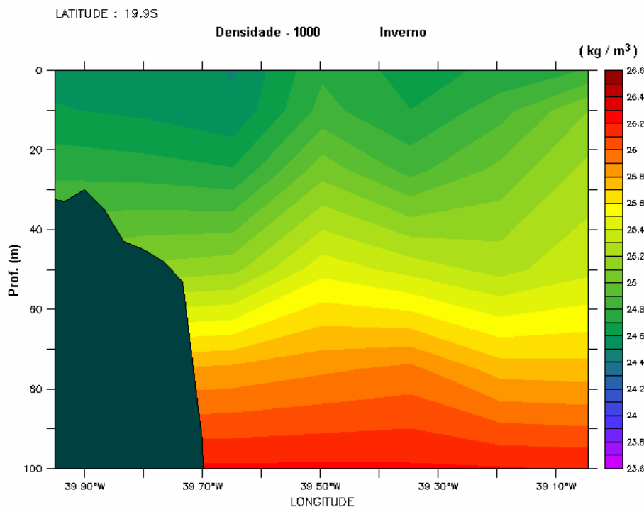
Figura V.2-2 - Seção vertical de densidade (kg/m 3 ) ao longo de 19,9°S, período de inverno. Dados provenientes do Atlas do WOCE.
