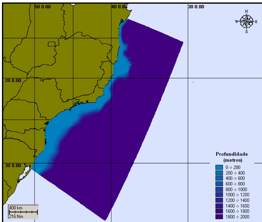
Figura II.3.1-3 - Batimetria discretizada do domínio considerado na Bacia do Espírito Santo.
