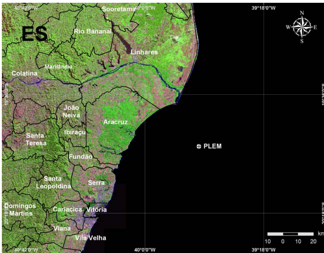
Figura I.1-1 - Localização do ponto de descarte, no Campo de Camarupim, Bacia do Espírito Santo.
