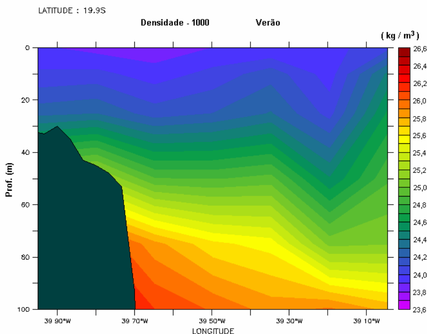
Figura V.2-1 - Seção vertical de densidade ( \text{kg/m}^3 ) ao longo de 19,9°S, período de verão. Dados provenientes do Atlas do WOCE.
