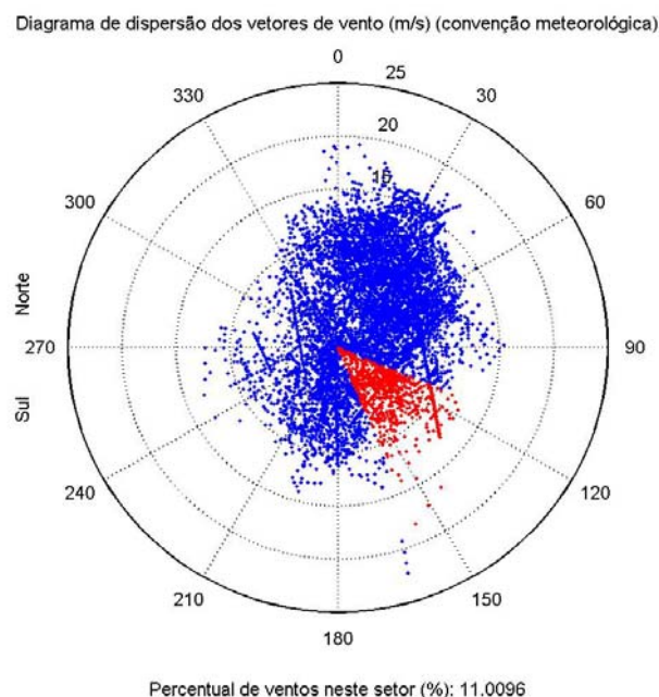
Figura VI.2.2-1 - Diagrama de dispersão do vento para o ano de 1992, na Bacia de Campos.
