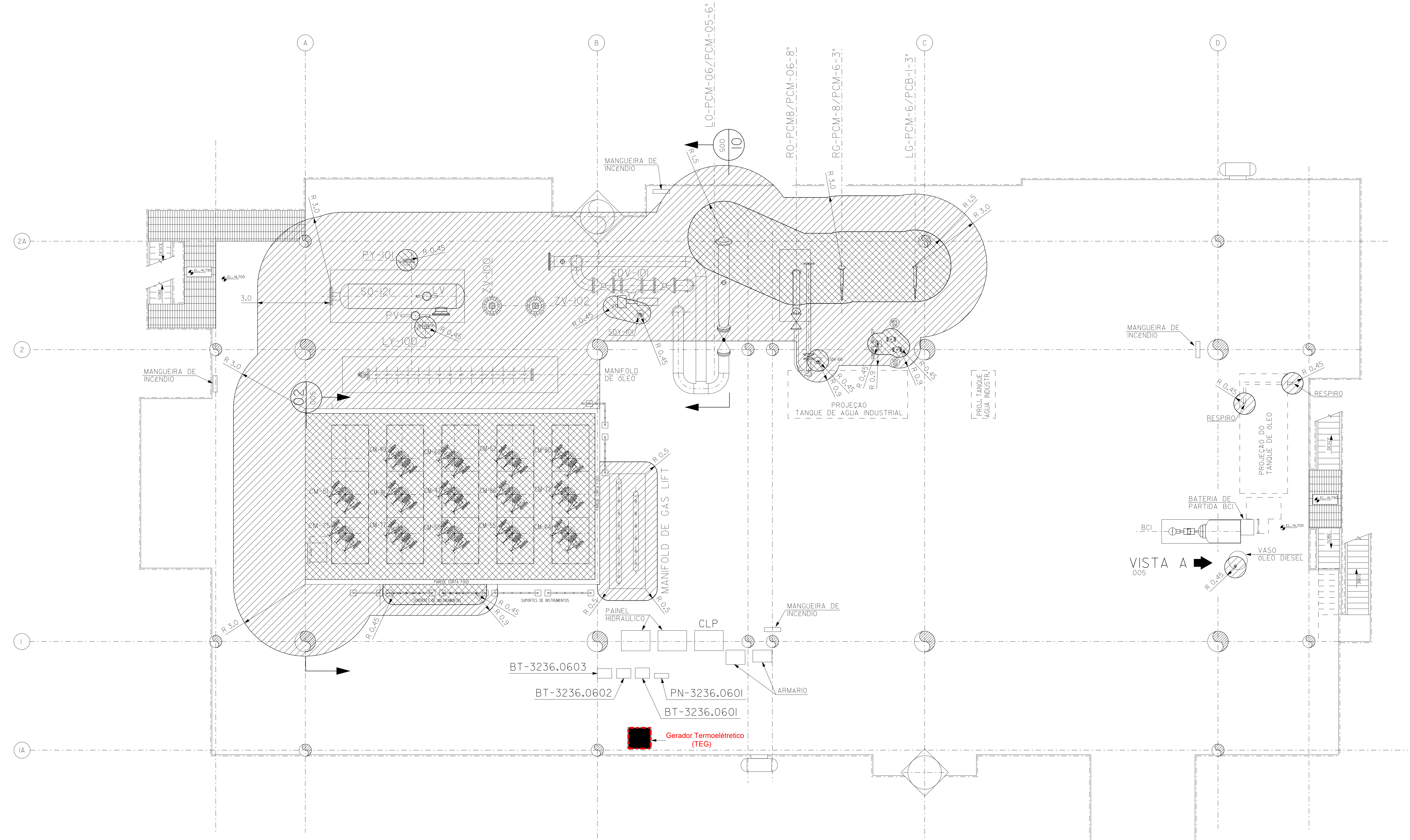
PLANTA BAIXA/ CONVES DE PRODUÇÃO EL. 14.700 ESC: 1/100
