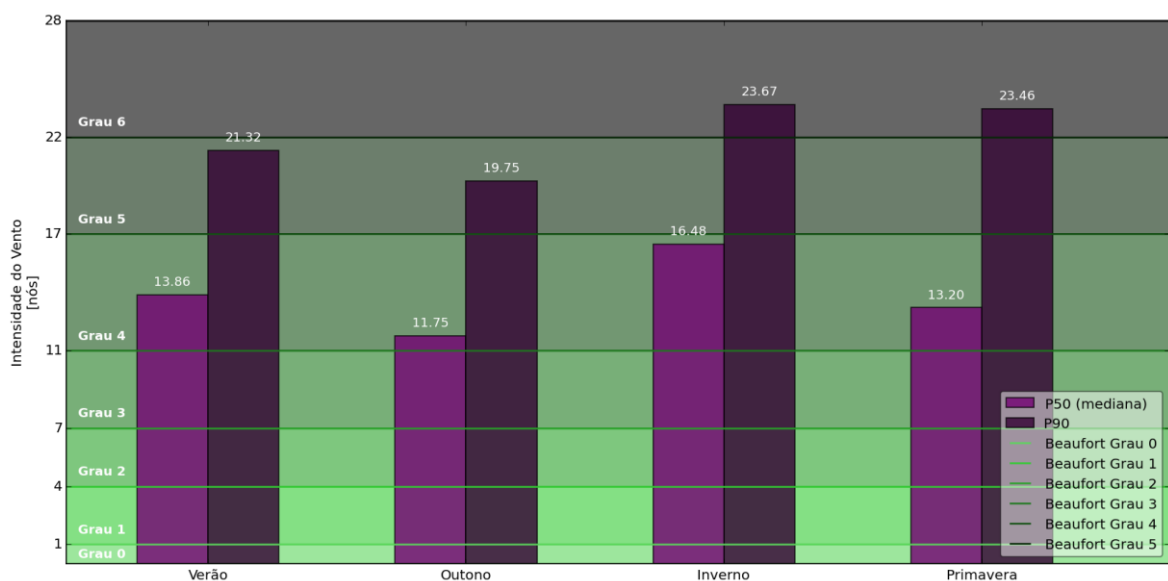
Figura VI.6.2-3 - Diagramas com barras de velocidade de vento com percentis de frequência de 50% e 90% (ventos não excedidos com este percentual) para um ponto da Bacia de Santos. Fonte: Dados do modelo WW3 da NOAA (USA).
