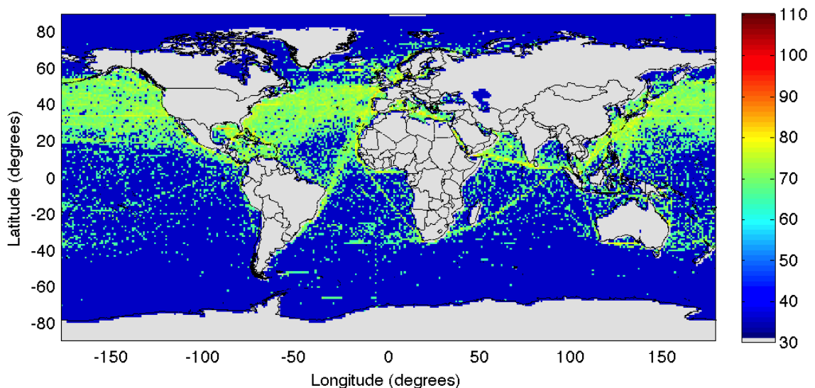
Figura VI.61 – Densidade de intensidade sonora [dB re 1\mu\text{Pa}^2/\text{Hz}@1\text{m}/\text{m}^2 ] em 200 Hz devido ao tráfego de embarcações (Fonte: http://oalib.hlsresearch.com ).
