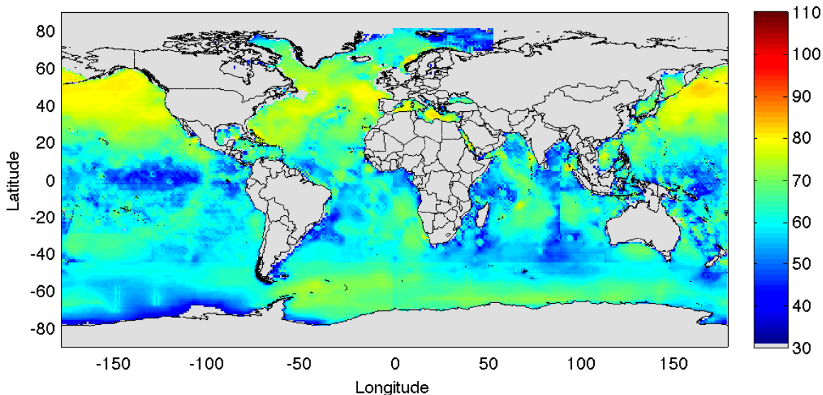
Figura VI.6-2 – Resultado da propagação do som no oceano [dB re 1\mu\text{Pa}^2/\text{Hz} ] obtida a partir da convolução do mapa da Figura VI.6-1 com as características físicas do oceano (Fonte: http://oalib.hlsresearch.com ).
