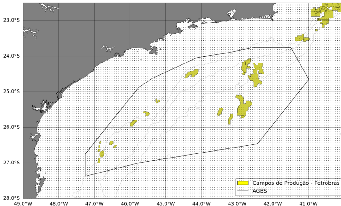
Figura VI.6.2-1 – Domínio de modelagem proposto para o modelo de propagação acústica oceânica. O grid mostrado está discretizado a 1/16 de grau apenas para fins de representação dos limites do domínio do modelo.
