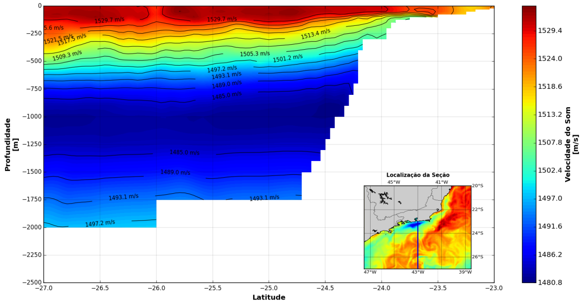
Figura VI.6.2-5 – Perfil de velocidade do som ao longo de uma seção longitudinal obtido de campos de temperatura e salinidade do modelo global HYCOM NCODA Analysis.
