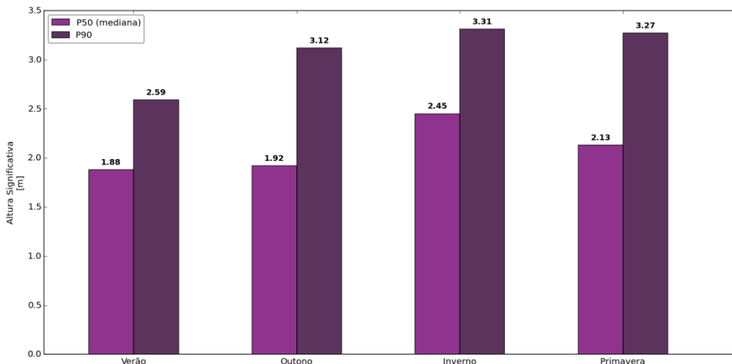
Figura VI.6.2-4 – Diagramas com barras de altura significativa H_s com percentis de frequência de 50% e 90% ( H_s não excedidas com este percentual) para um ponto da Bacia de Santos. Fonte: Dados do modelo WW3 da NOAA (USA).
