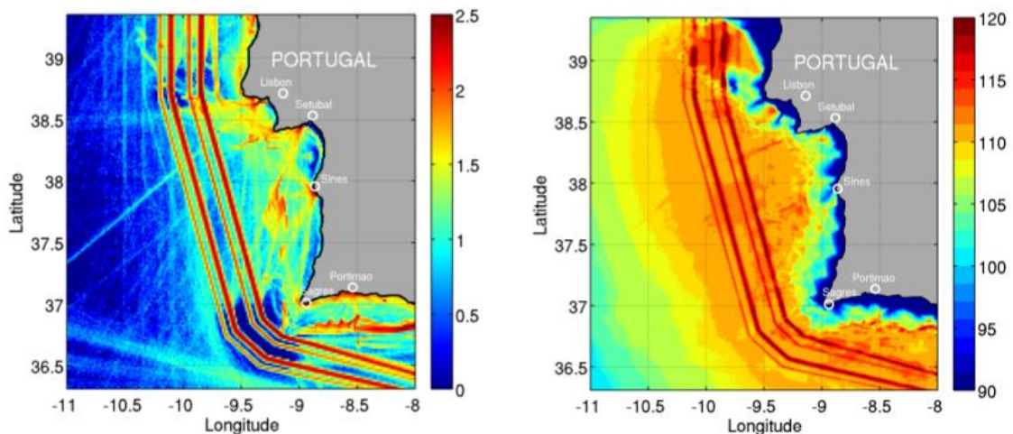
Figura VI.6.3-1 – Densidade acumulada de embarcações obtida a partir de dados de AIS para o ano de 2014 no litoral de Portugal (à esquerda); resultados obtidos com o modelo de propagação de modos normais mostrando o SPL médio [dB re 1 \mu Pa] em 80 m de profundidade considerando uma banda de 32 a 1008 Hz (à direita) (Fonte: Soares et al., 2015).
